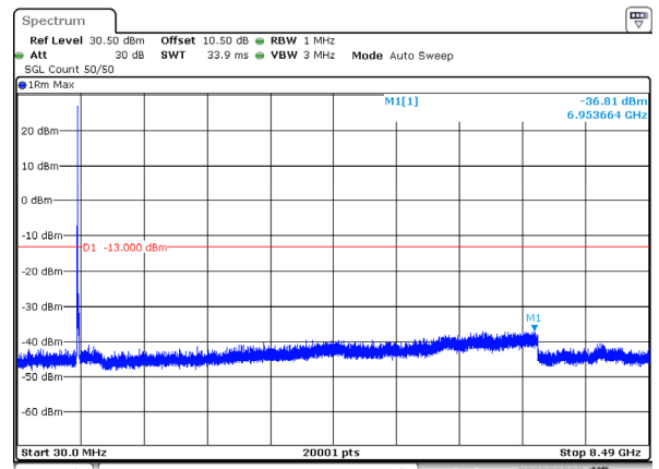
n5_20MHz_15kHz_839MHz_DFT-s-OFDM QPSK_RB1@0 -36.81dBm
