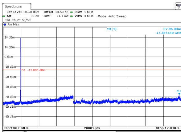
n66_25MHz_15kHz_1745MHz_DFT-s-OFDM QPSK_RB1@132 -37.96dBm
