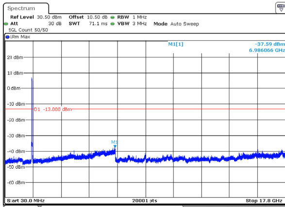
n66_25MHz_15kHz_1722.5MHz_DFT-s-OFDM QPSK_RB128@0 -37.59dBm
