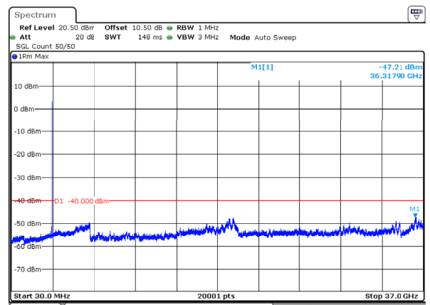
n78_2_15MHz_30kHz_3625MHz_DFT-s-OFDM QPSK_RB36@0 -47.21dBm
