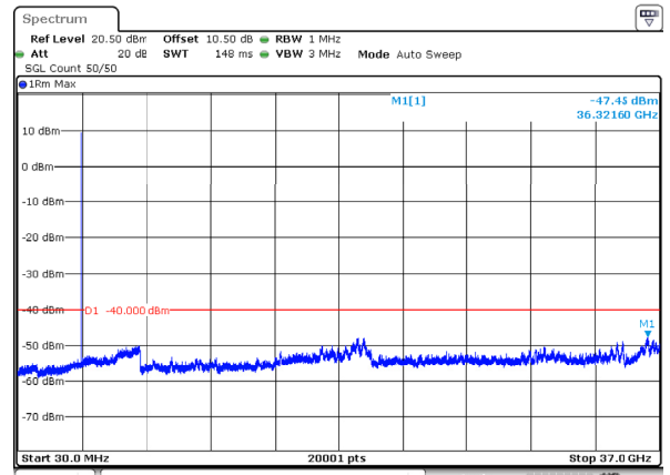
n78_2_15MHz_30kHz_3625MHz_DFT-s-OFDM QPSK_RB1@0 -47.45dBm
