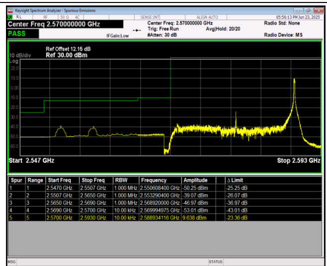
Band38-20MHz-QPSK-38150-1RB#0
