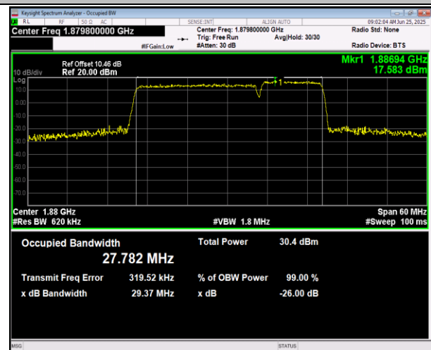
2-2-20MHz-10MHz-16QAM-16QAM-19001-19145-100RB#0-50RB#0-PASS
