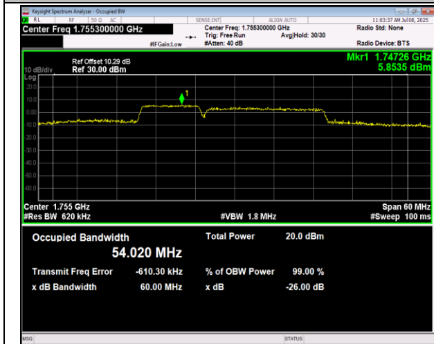
66-66-10MHz-20MHz-QPSK-QPSK-132428-132572-50R B#0-100RB#0-PASS
