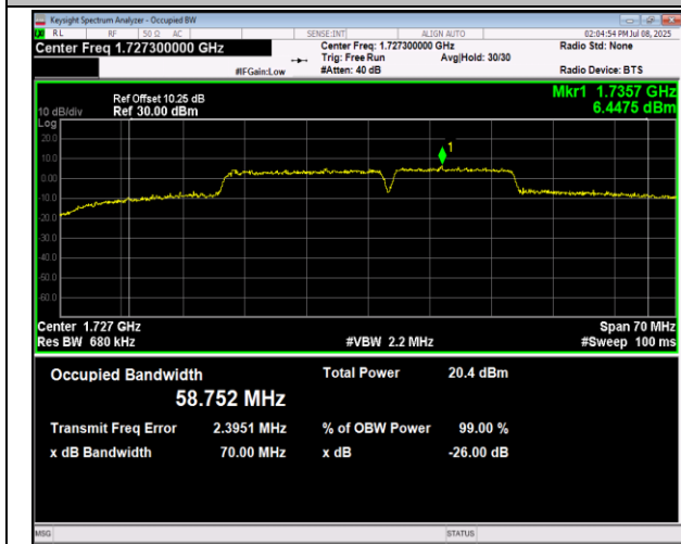
66-66-20MHz-15MHz-QPSK-QPSK-132348-132519-100 RB#0-75RB#0-PASS
