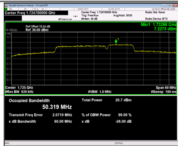
66-66-20MHz-10MHz-16QAM-16QAM-132373-132517-100 RB#0-50RB#0-PASS
