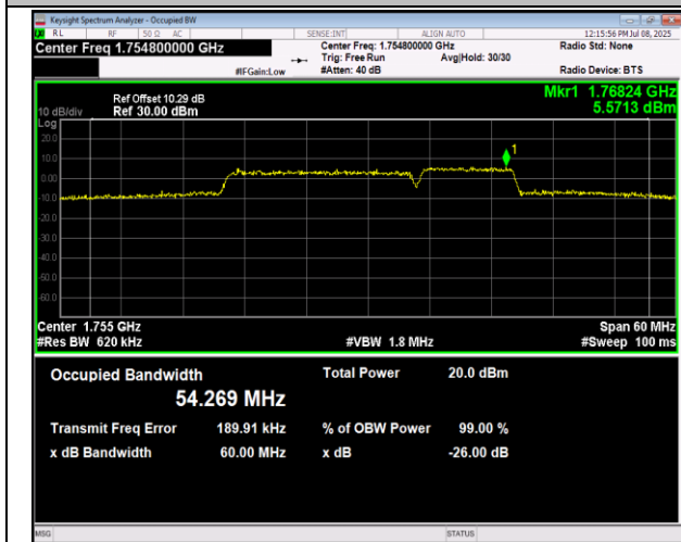
66-66-20MHz-10MHz-QPSK-QPSK-132473-132617-100 RB#0-50RB#0-PASS
