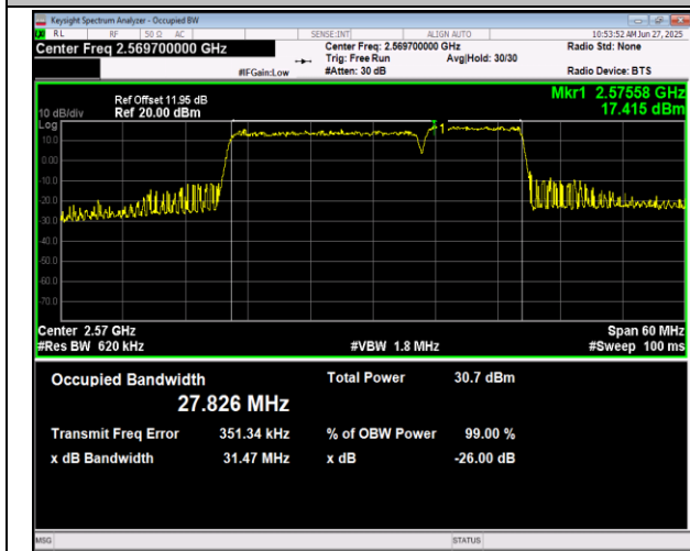
41(2555-2655)-41(2555-2655)-20MHz-10MHz-QPSK-QP SK-40691-40835-100RB#0-50RB#0-PASS
