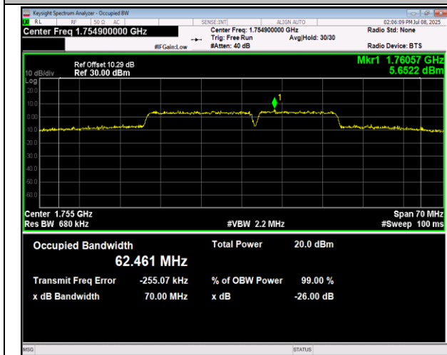
66-66-20MHz-15MHz-QPSK-QPSK-132423-132594-100 RB#0-75RB#0-PASS
