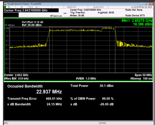
41(2555-2655)-41(2555-2655)-20MHz-10MHz-16QAM-16Q AM-40340-40484-100RB#0-50RB#0-PASS
