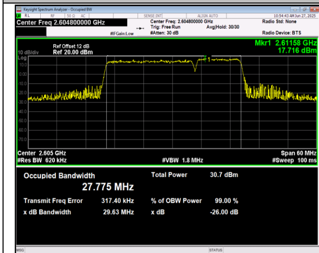
41(2555-2655)-41(2555-2655)-20MHz-10MHz-QPSK-QP SK-41041-41185-100RB#0-50RB#0-PASS
