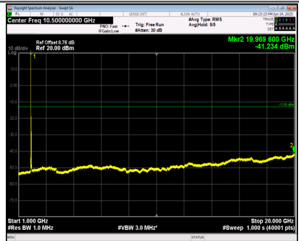
2-2-5MHz-20MHz-16QAM-16QAM-18633-18750-1RB#0-1R B#99-1000~20000MHz-PASS
