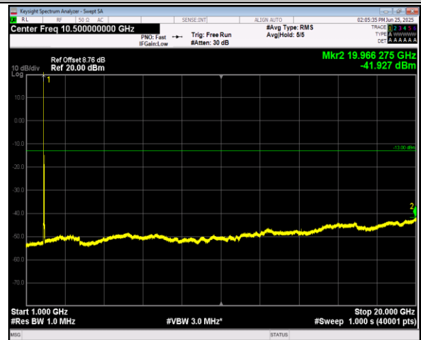
2-2-20MHz-20MHz-16QAM-16QAM-18700-18898-1RB#0-1RB#99-1000~20000MHz-PASS
