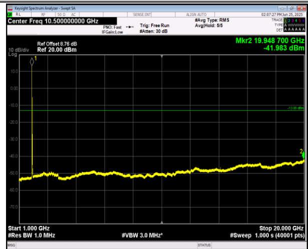
2-2-20MHz-20MHz-QPSK-QPSK-18700-18898-1RB#99-0RB B#0-1000~20000MHz-PASS
