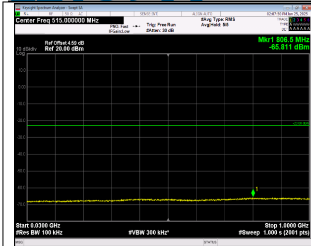
2-2-20MHz-20MHz-16QAM-16QAM-18700-18898-1RB#9 9-0RB#0-30~1000MHz-PASS
