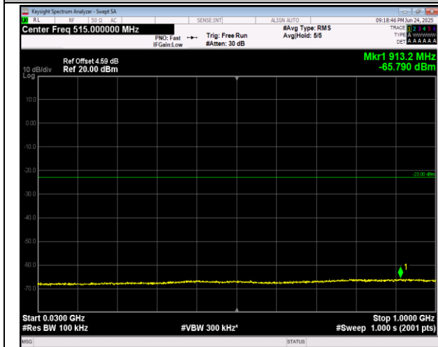
2-2-5MHz-20MHz-QPSK-QPSK-18808-18925-1RB#0-0R B#0-30~1000MHz-PASS
