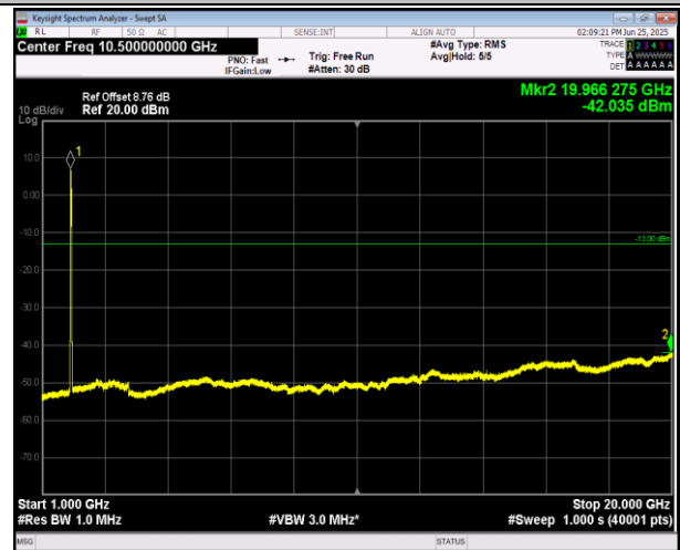
2-2-20MHz-20MHz-QPSK-QPSK-18801-18999-1RB#0-0RB #0-1000~20000MHz-PASS
