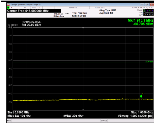
2-2-20MHz-20MHz-16QAM-16QAM-18700-18898-1RB#0-0RB#0-0-30~1000MHz-PASS
