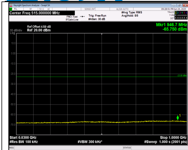
2-2-20MHz-20MHz-QPSK-QPSK-18700-18898-1RB#0-0 RB#0-30~1000MHz-PASS
