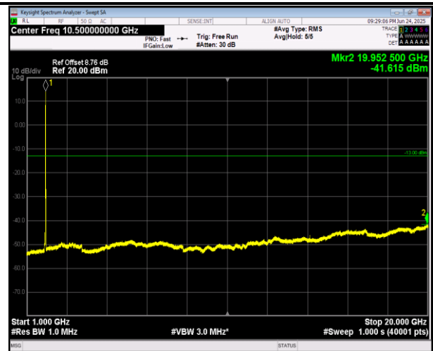
2-2-20MHz-20MHz-QPSK-QPSK-18700-18898-1RB#0-0RB #0-1000~20000MHz-PASS
