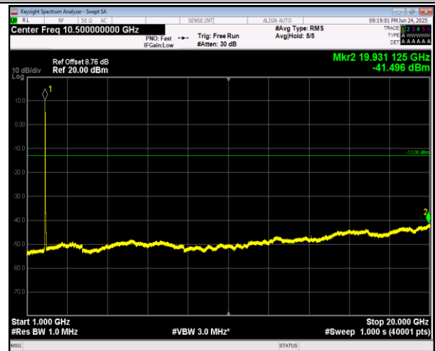
2-2-5MHz-20MHz-QPSK-QPSK-18808-18925-1RB#0-0RB# 0-1000~20000MHz-PASS
