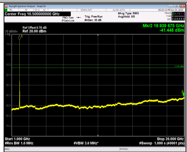
2-2-5MHz-20MHz-QPSK-QPSK-18808-18925-1RB#24-0RB #0-1000~20000MHz-PASS
