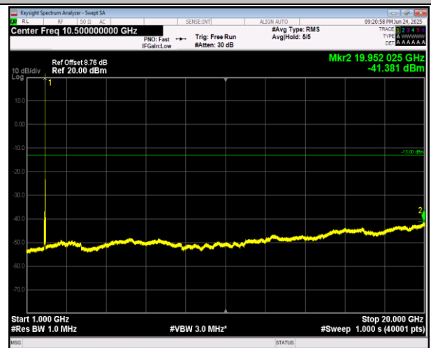
2-2-5MHz-20MHz-QPSK-QPSK-18808-18925-25RB#0-100 RB#0-1000~20000MHz-PASS
