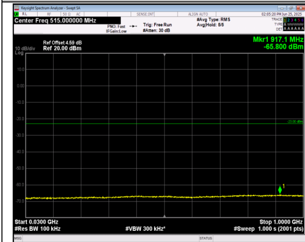
2-2-20MHz-20MHz-16QAM-16QAM-18700-18898-1RB#0-1RB#99-30~1000MHz-PASS
