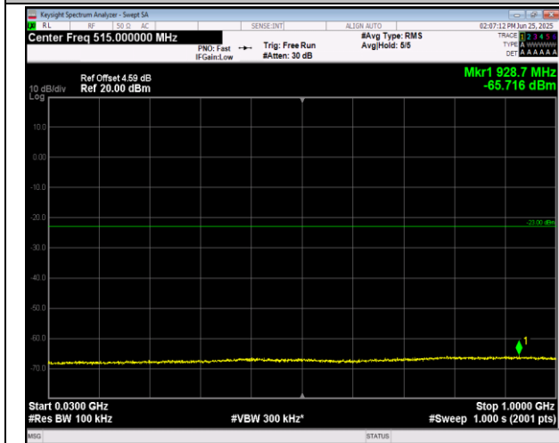
2-2-20MHz-20MHz-QPSK-QPSK-18700-18898-1RB#99-0 RB#0-30~1000MHz-PASS
