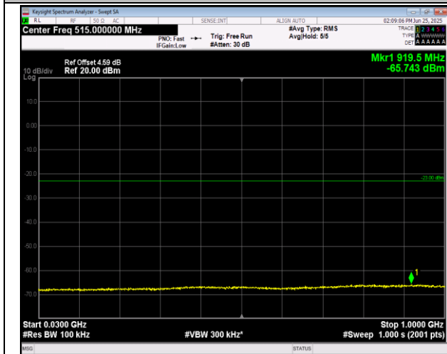
2-2-20MHz-20MHz-QPSK-QPSK-18801-18999-1RB#0-0 RB#0-30~1000MHz-PASS
