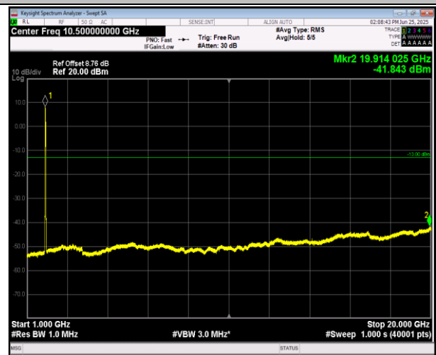
2-2-20MHz-20MHz-16QAM-16QAM-18700-18898-1RB#0-0RB#0-1000~20000MHz-PASS
