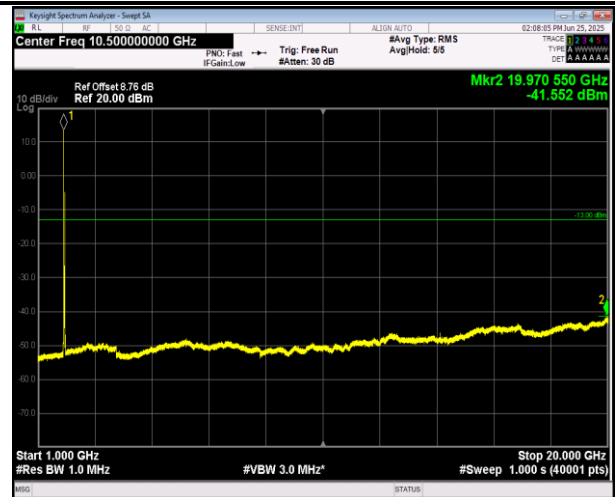
2-2-20MHz-20MHz-16QAM-16QAM-18700-18898-1RB#99- 0RB#0-1000~20000MHz-PASS
