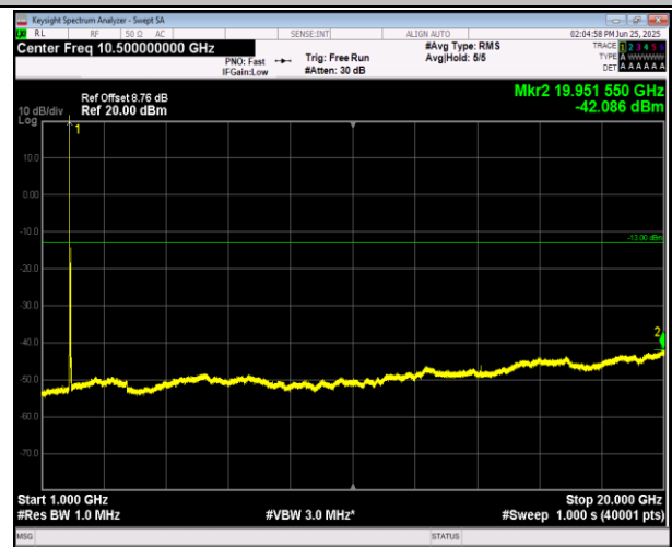
2-2-20MHz-20MHz-QPSK-QPSK-18700-18898-1RB#0-1RB #99-1000~20000MHz-PASS
