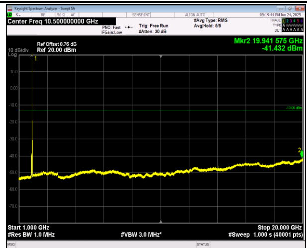
2-2-5MHz-20MHz-QPSK-QPSK-18808-18925-1RB#0-1RB# 99-1000~20000MHz-PASS
