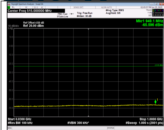
2-2-20MHz-20MHz-QPSK-QPSK-18700-18898-100RB#0-100RB#0-30~1000MHz-PASS
