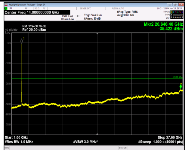
7-7-20MHz-10MHz-QPSK-QPSK-20850-20994-1RB#0-0RB #0-1000~27000MHz-PASS
