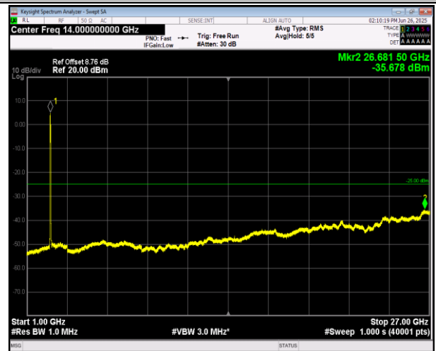
7-7-20MHz-20MHz-QPSK-QPSK-21001-21199-1RB#0-0RB #0-1000~27000MHz-PASS
