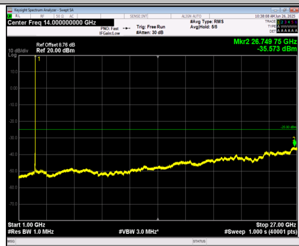
7-7-20MHz-10MHz-QPSK-QPSK-21251-21395-100RB#0-50RB#0-30~1000MHz-PASS ORB#0-1000~27000MHz-PASS
