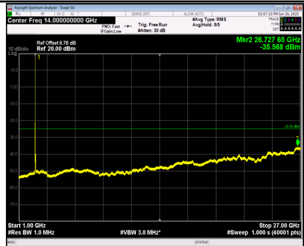
7-7-20MHz-20MHz-QPSK-QPSK-20850-21048-100RB#0-100RB#0-1000~27000MHz-PASS
