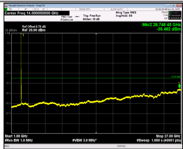
7-7-20MHz-10MHz-QPSK-QPSK-20850-20994-1RB#0-1RB #49-1000~27000MHz-PASS
