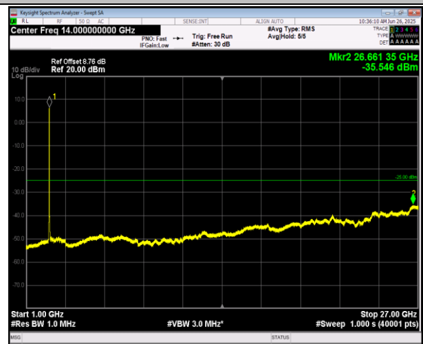
7-7-20MHz-10MHz-QPSK-QPSK-21251-21395-1RB#0-0RB #0-1000~27000MHz-PASS
