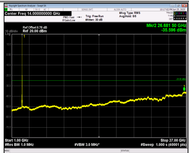
7-7-10MHz-20MHz-QPSK-QPSK-21206-21350-1RB#0-1RB#99-1000~27000MHz-PASS
