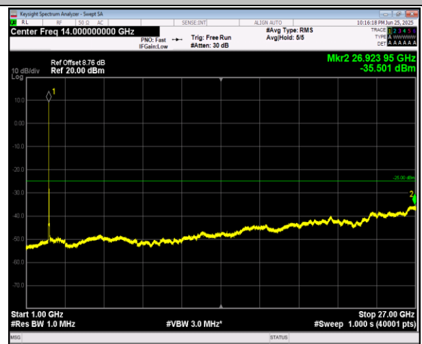
7-7-10MHz-20MHz-QPSK-QPSK-21206-21350-1RB#0-0RB#0-1000~27000MHz-PASS
