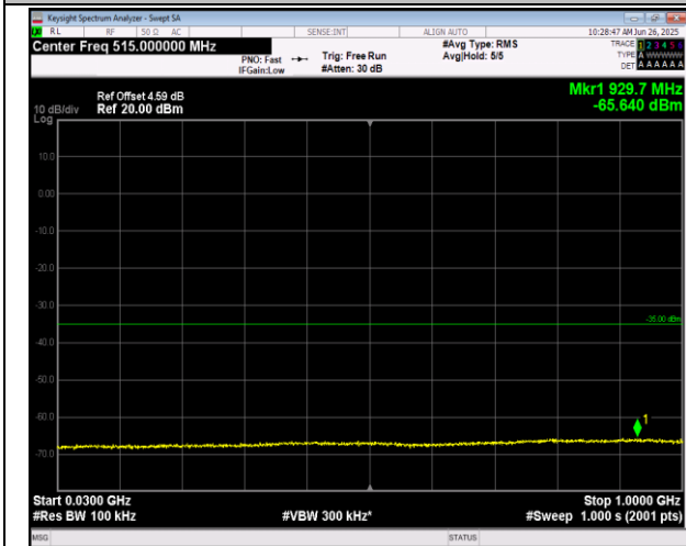
7-7-20MHz-10MHz-QPSK-QPSK-20850-20994-1RB#99-0 RB#0-30~1000MHz-PASS
