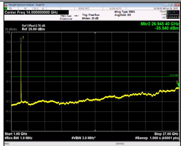
7-7-20MHz-10MHz-QPSK-QPSK-20850-20994-1RB#99-0R B#0-1000~27000MHz-PASS
