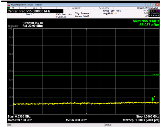
38-38-20MHz-20MHz-QPSK-QPSK-37901-38099-1RB#0- ORB#0-30~1000MHz-PASS
