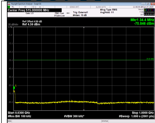
41(2555-2655)-41(2555-2655)-20MHz-20MHz-16QAM-16 QAM-40641-40839-1RB#0-0RB#0-30~1000MHz-PASS
