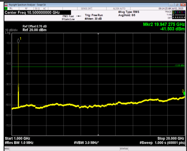
66-66-5MHz-20MHz-QPSK-QPSK-132330-132447-1RB#0- 1RB#99-1000~20000MHz-PASS
