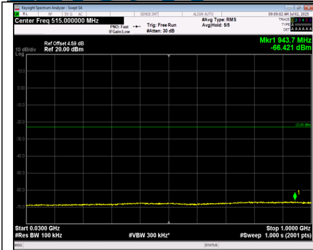
66-66-5MHz-20MHz-QPSK-QPSK-132005-132122-25RB #0-100RB#0-30~1000MHz-PASS
