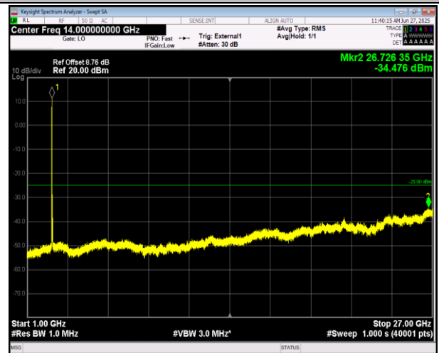
41(2555-2655)-41(2555-2655)-20MHz-20MHz-16QAM-16Q AM-40641-40839-1RB#99-0RB#0-1000~27000MHz-PASS
