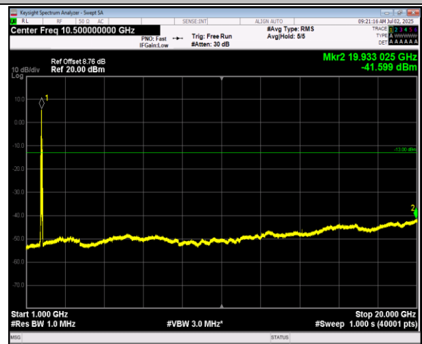
66-66-5MHz-20MHz-QPSK-QPSK-132330-132447-1RB#24 -0RB#0-1000~20000MHz-PASS
