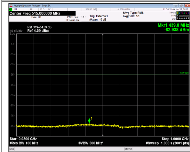
41(2555-2655)-41(2555-2655)-20MHz-20MHz-16QAM-16 QAM-40641-40839-1RB#0-1RB#99-30~1000MHz-PASS
