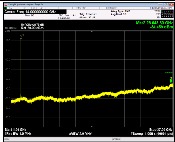
41(2555-2655)-41(2555-2655)-20MHz-20MHz-QPSK-QPS K-40942-41140-1RB#99-0RB#0-1000~27000MHz-PASS
