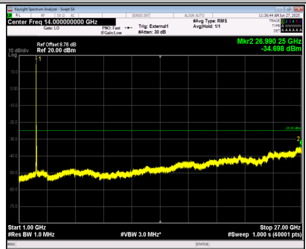
41(2555-2655)-41(2555-2655)-20MHz-20MHz-16QAM-16Q AM-40641-40839-1RB#0-1RB#99-1000~27000MHz-PASS
