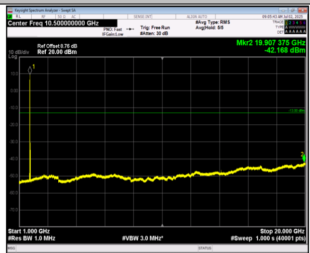
66-66-5MHz-20MHz-QPSK-QPSK-132005-132122-1RB#0- 1RB#99-1000~20000MHz-PASS
