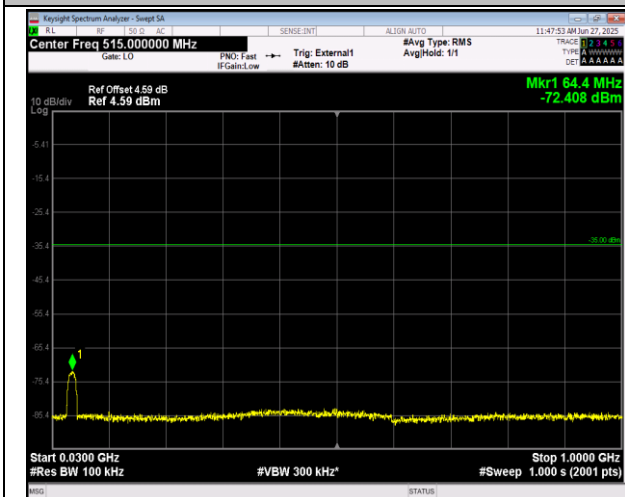
41(2555-2655)-41(2555-2655)-20MHz-20MHz-16QAM-16 QAM-40942-41140-1RB#0-0RB#0-30~1000MHz-PASS
