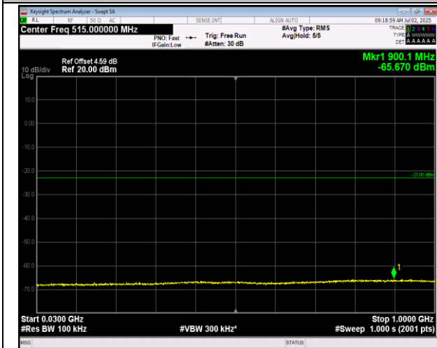
66-66-5MHz-20MHz-QPSK-QPSK-132330-132447-25RB #0-100RB#0-30~1000MHz-PASS
