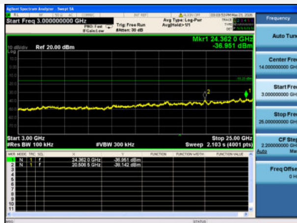
3 GHz ~ 25 GHz
