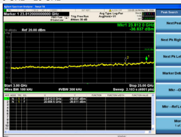
3 GHz ~ 25 GHz
