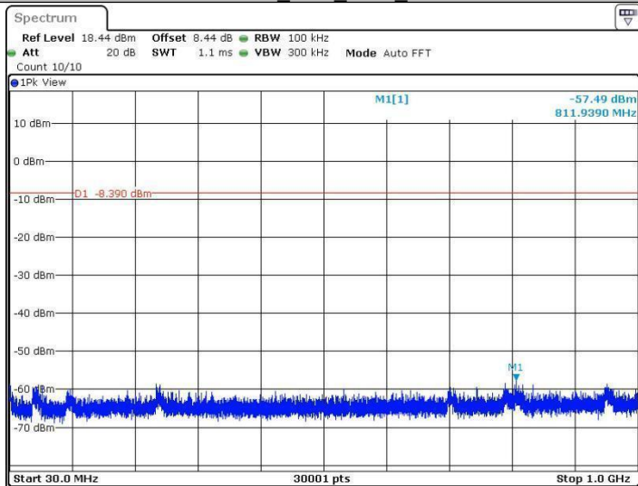
2.4G custom_Ant2_2404_30~1000
