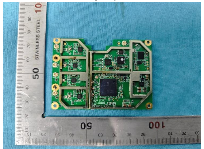
EUT 12
