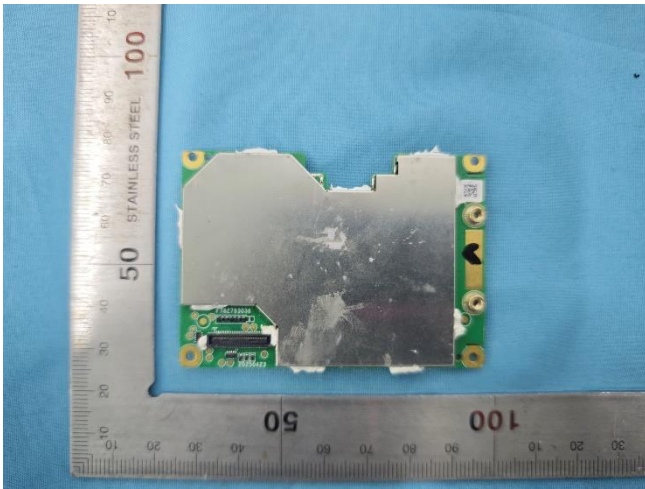
EUT 13
