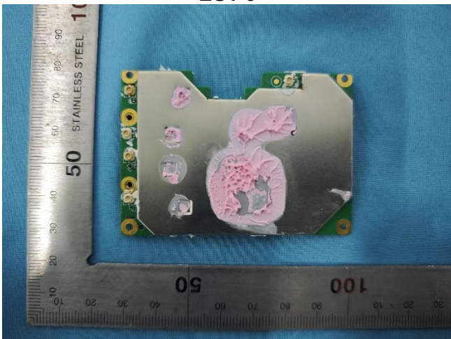
EUT 11
