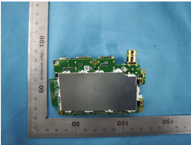
EUT 9
