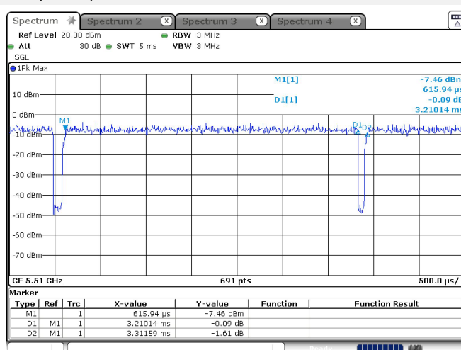
11n(HT40)-5510 MHz
