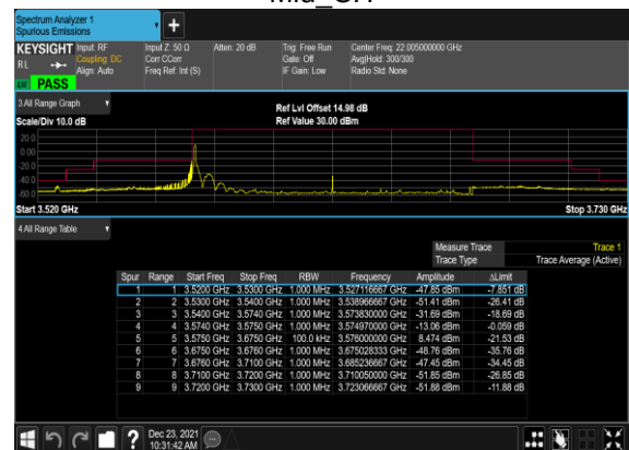
N48(100M)_CP-OFDM_QPSK_Edge_1RB_Left_
