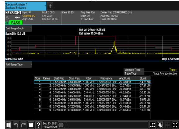
N48(50M)_CP-OFDM_QPSK_Edge_1RB_Left_ High CH
