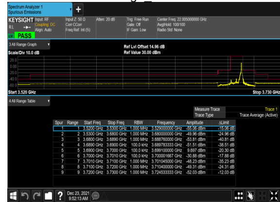
N48(50M)_CP-OFDM_QPSK_Edge_1RB_Left_ Low CH
