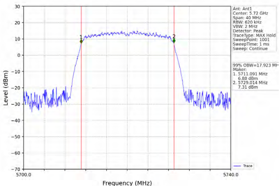
802.11n(HT20)_HCH_5720MHz_Ant1_NTNV
