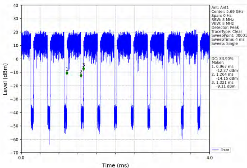
802.11ax(HEW80)_HCH_5690MHz_RU996_Left_Ant1_NTNV
