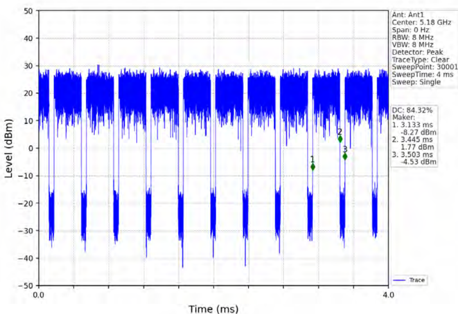
802.11ax(HEW20)_LCH_5180MHz_RU242_Left_Ant1_NTNV
