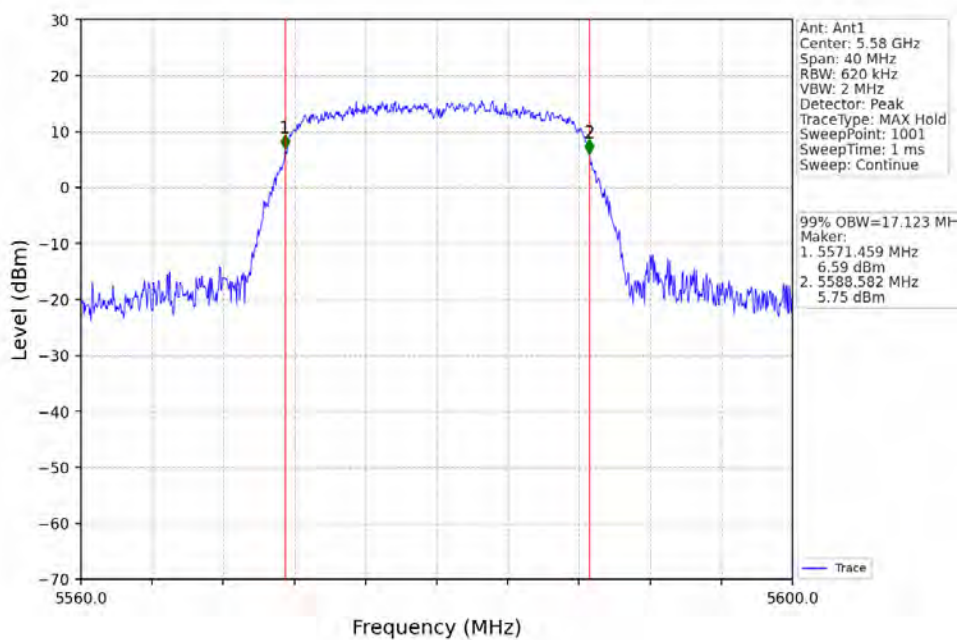
802.11a_MCH_5580MHz_Ant1_NTNV
