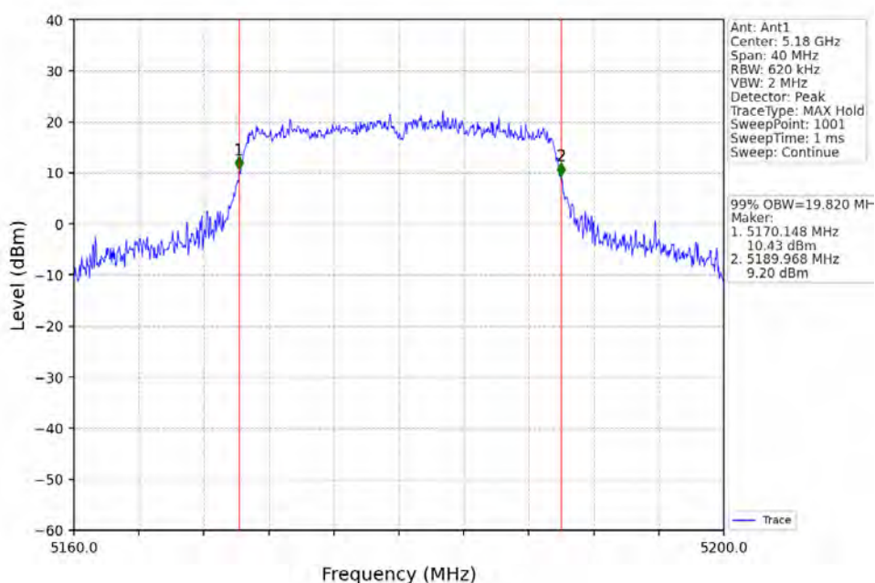
802.11ax(HEW20)_LCH_5180MHz_RU242_Left_Ant1_NTNV
