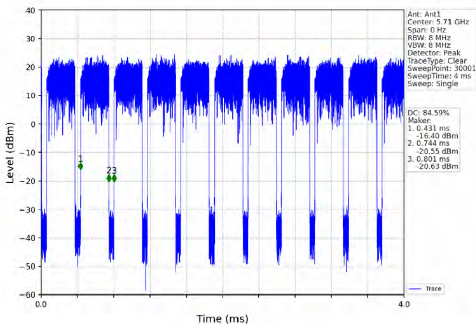
802.11ax(HEW40)_HCH_5710MHz_RU484_Left_Ant1_NTNV
