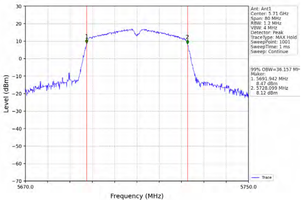
802.11n(HT40)_HCH_5710MHz_Ant1_NTNV
