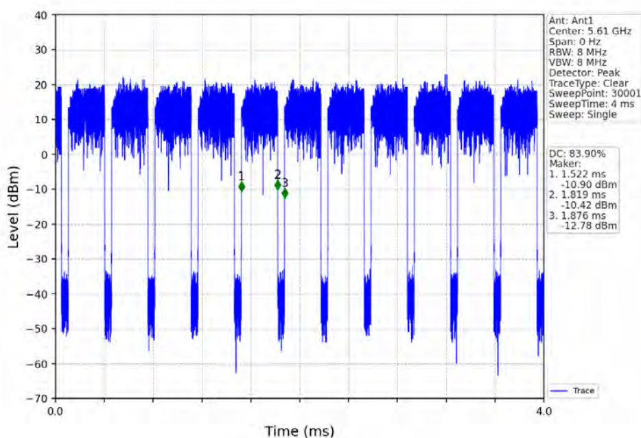
802.11ax(HEW80)_HCH_5610MHz_RU996_Left_Ant1_NTNV
