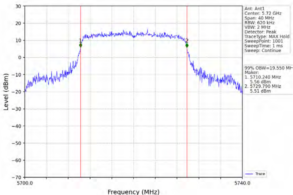
802.11ax(HEW20)_HCH_5720MHz_RU242_Left_Ant1_NTNV
