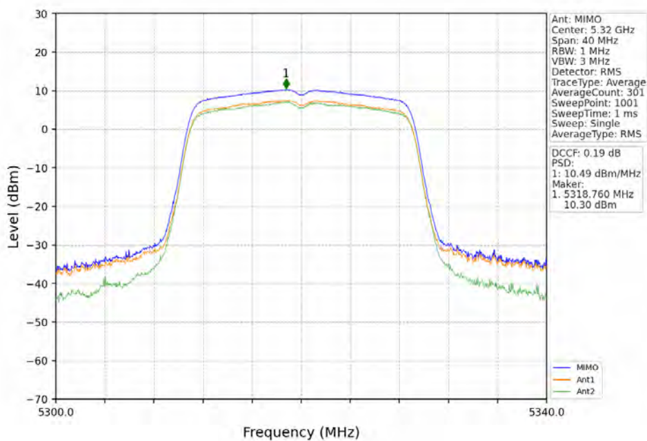
802.11n(HT20)_HCH_5320MHz_MIMO_NTNV
