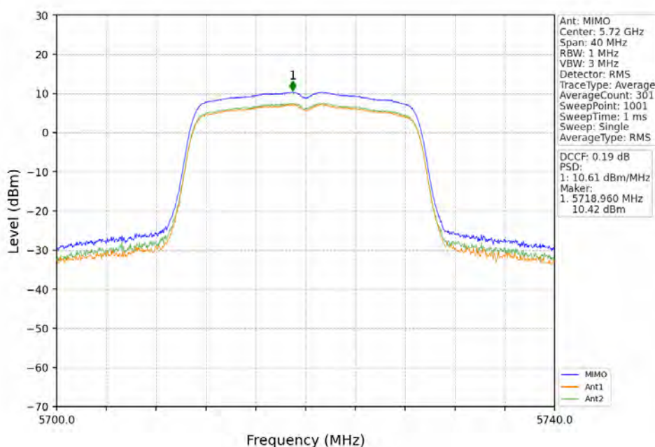
802.11n(HT20)_HCH_5720MHz_MIMO_NTNV
