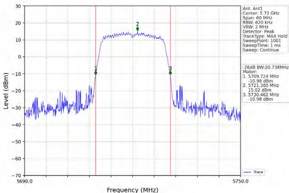
802.11ac(VHT20)_HCH_5720MHz_Ant1_NTNV
