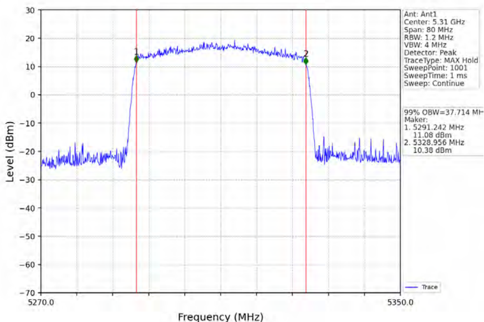
802.11ax(HEW40)_HCH_5310MHz_RU484_Left_Ant1_NTNV
