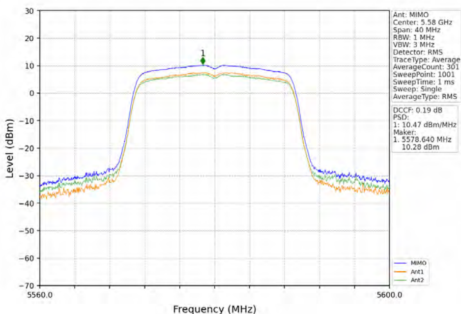
802.11n(HT20)_MCH_5580MHz_MIMO_NTNV
