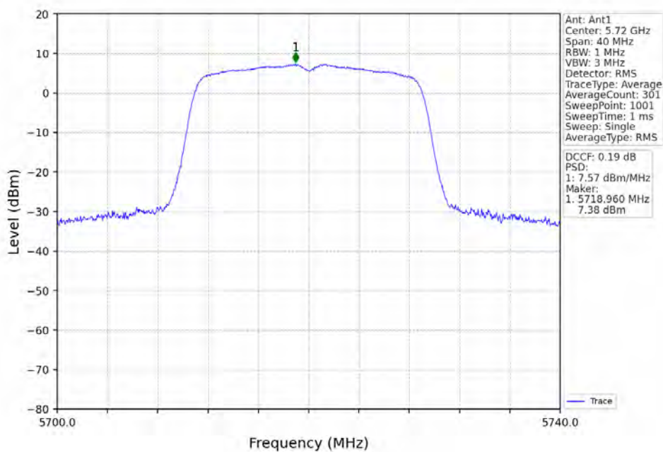
802.11n(HT20)_HCH_5720MHz_Ant1_NTNV
