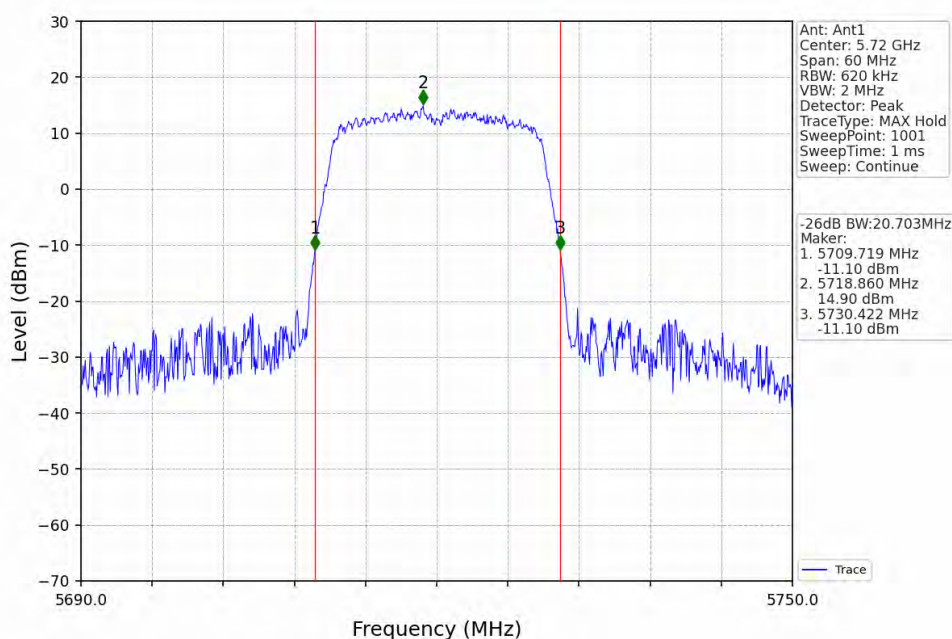
802.11n(HT20)_HCH_5720MHz_Ant1_NTNV
