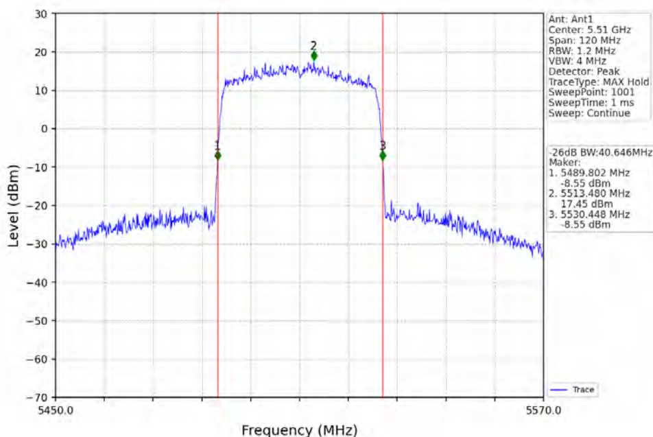
802.11ax(HEW40)_LCH_5510MHz_RU484_Left_Ant1_NTNV
