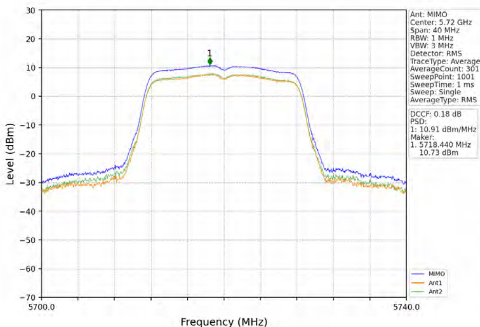
802.11a_HCH_5720MHz_MIMO_NTNV
