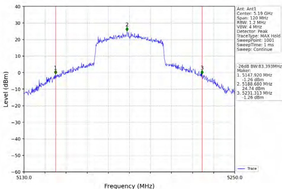
802.11ax(HEW40)_LCH_5190MHz_RU484_Left_Ant1_NTNV
