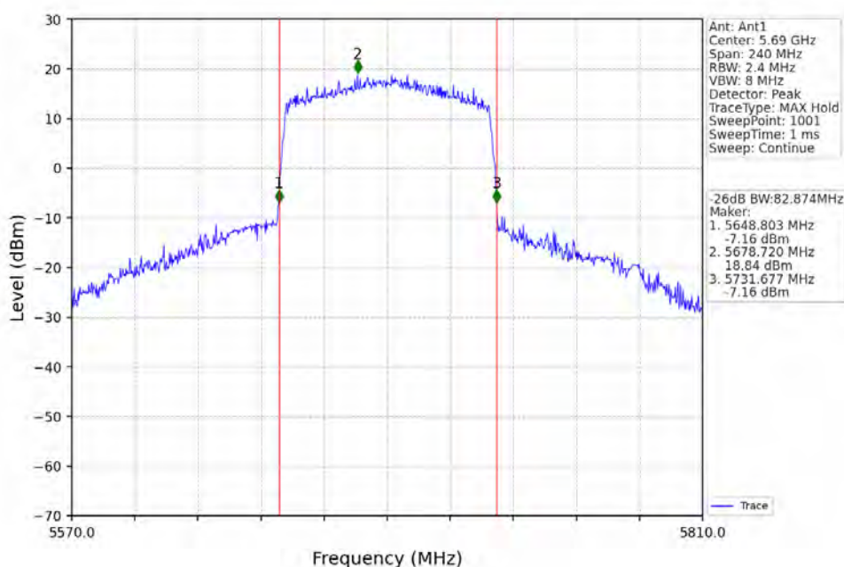
802.11ax(HEW80)_HCH_5690MHz_RU996_Left_Ant1_NTNV
