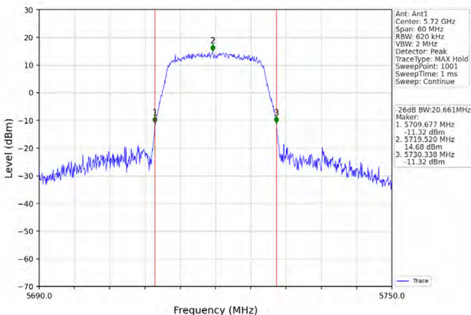
802.11a_HCH_5720MHz_Ant1_NTNV
