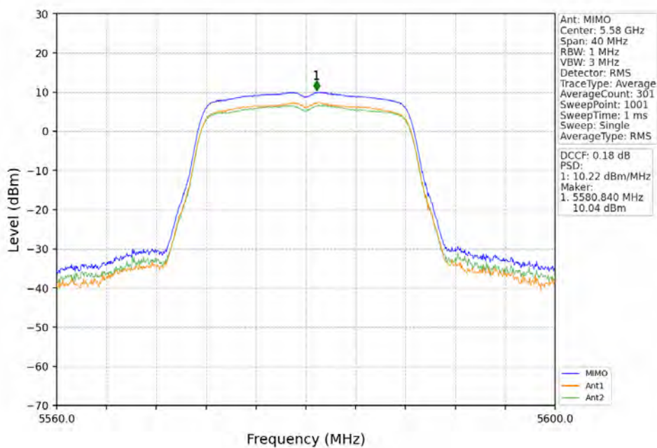
802.11a_MCH_5580MHz_MIMO_NTNV
