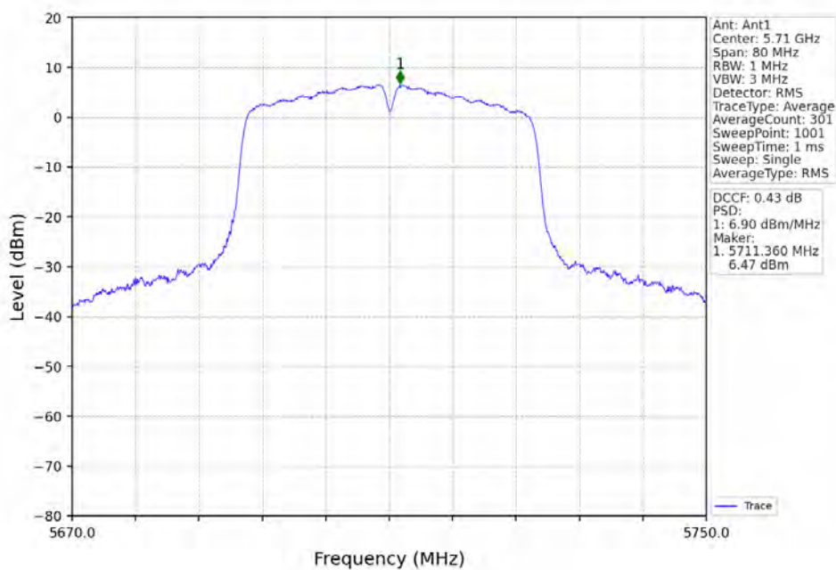
802.11n(HT40)_HCH_5710MHz_Ant1_NTNV
