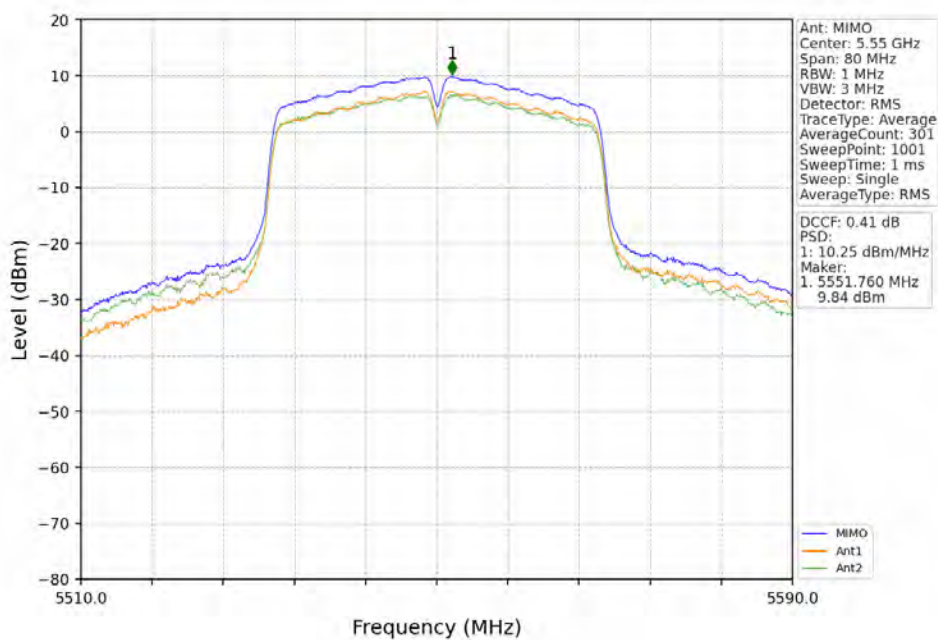
802.11n(HT40)_MCH_5550MHz_MIMO_NTNV
