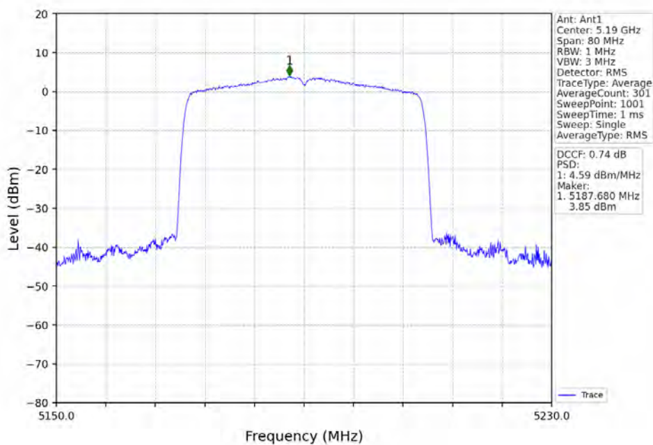
802.11ax(HEW40)_LCH_5190MHz_RU484_Left_Ant1_NTNV
