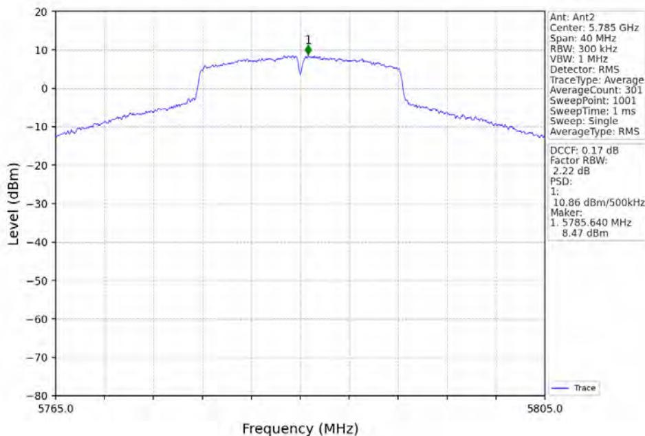
802.11a_MCH_5785MHz_MIMO_NTNV
