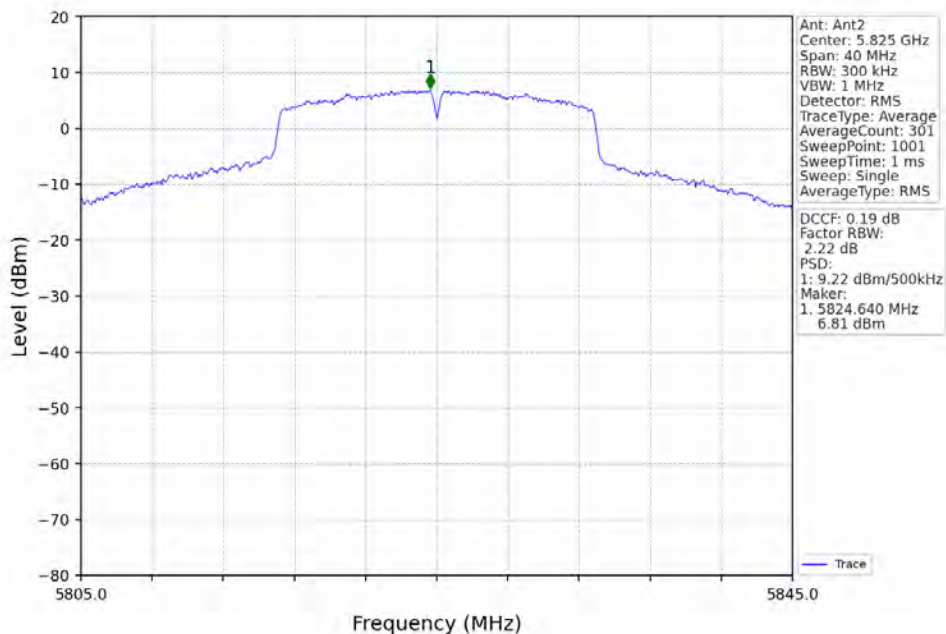
802.11n(HT20)_HCH_5825MHz_MIMO_NTNV
