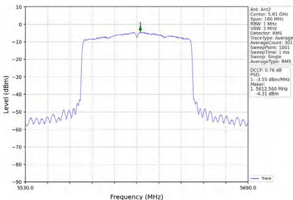
802.11ax(HEW80)_HCH_5610MHz_RU996_Left_Ant2_NTNV
