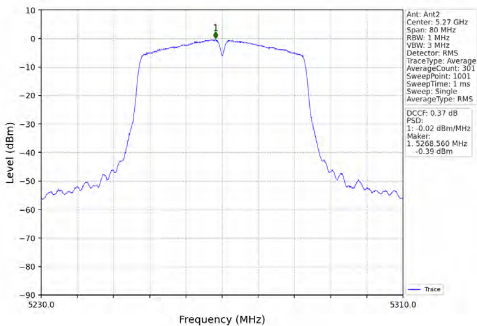
802.11ac(VHT40)_LCH_5270MHz_Ant2_NTNV
