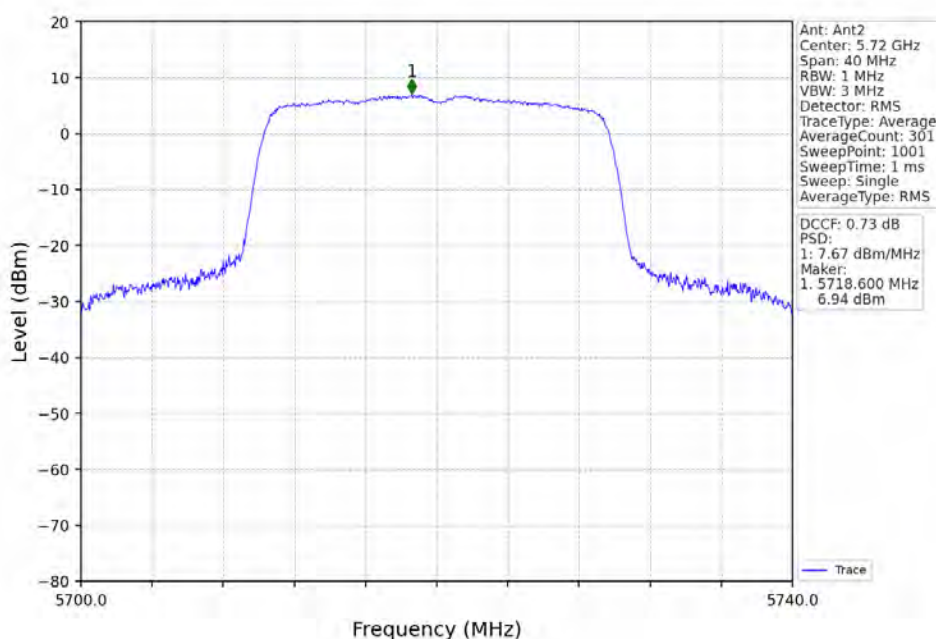
802.11ax(HEW20)_HCH_5720MHz_RU242_Left_Ant2_NTNV
