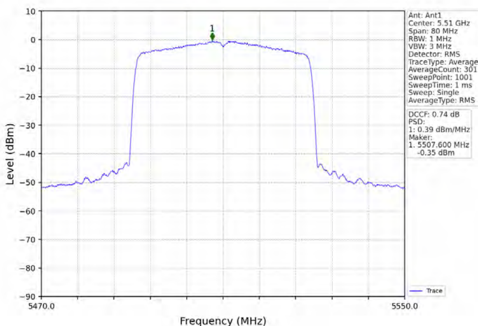
802.11ax(HEW40)_LCH_5510MHz_RU484_Left_Ant1_NTNV
