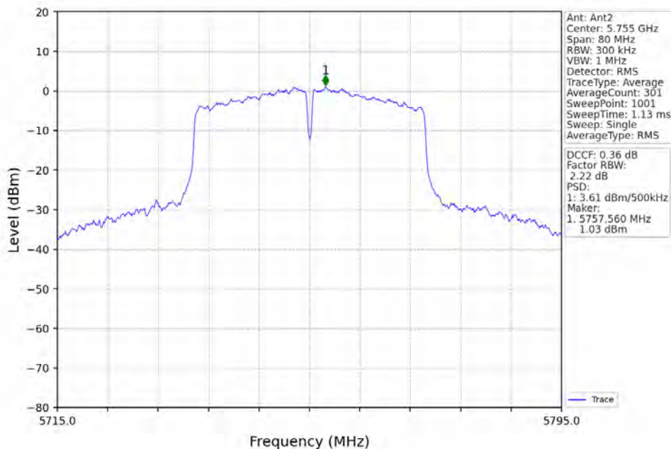
802.11ac(VHT40)_LCH_5755MHz_MIMO_NTNV
