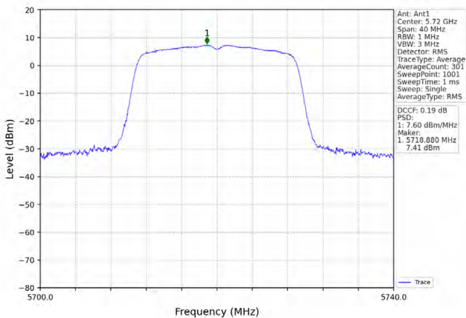
802.11ac(VHT20)_HCH_5720MHz_Ant1_NTNV
