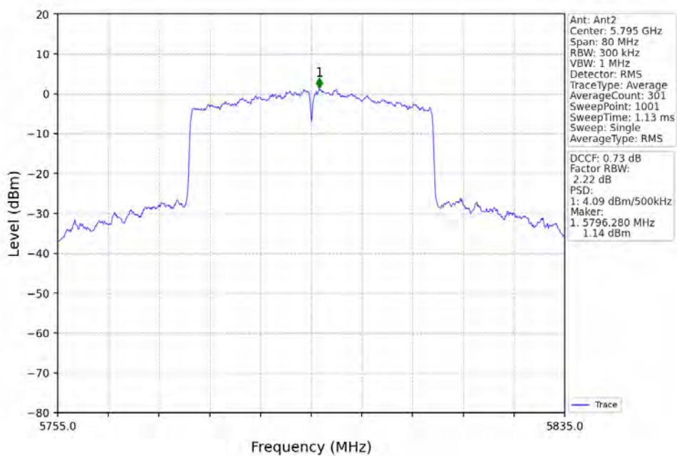
802.11ax(HEW40)_HCH_5795MHz_RU484_Left_Ant2_NTNV
