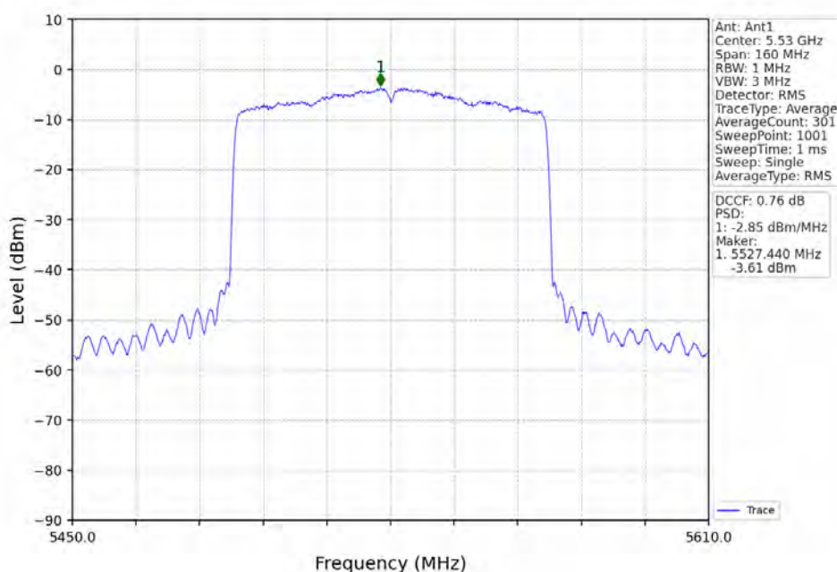
802.11ax(HEW80)_LCH_5530MHz_RU996_Left_Ant1_NTNV
