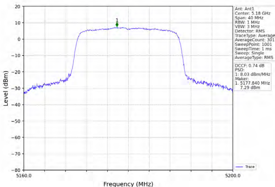
802.11ax(HEW20)_LCH_5180MHz_RU242_Left_Ant1_NTNV
