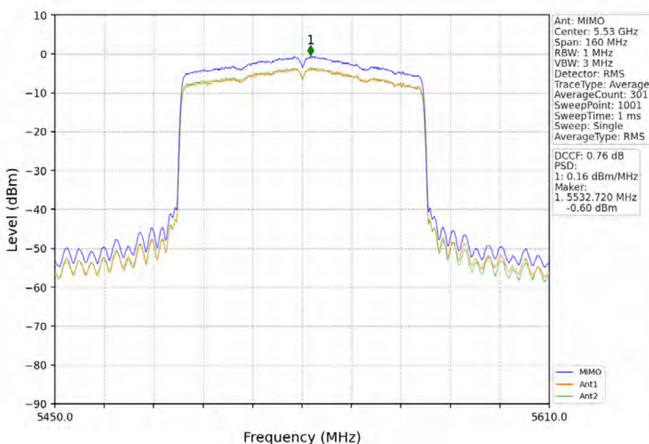
802.11ax(HEW80)_LCH_5530MHz_RU996_Left_MIMO_NTNV
