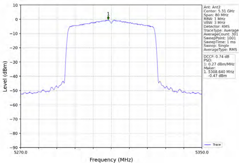
802.11ax(HEW40)_HCH_5310MHz_RU484_Left_Ant2_NTNV
