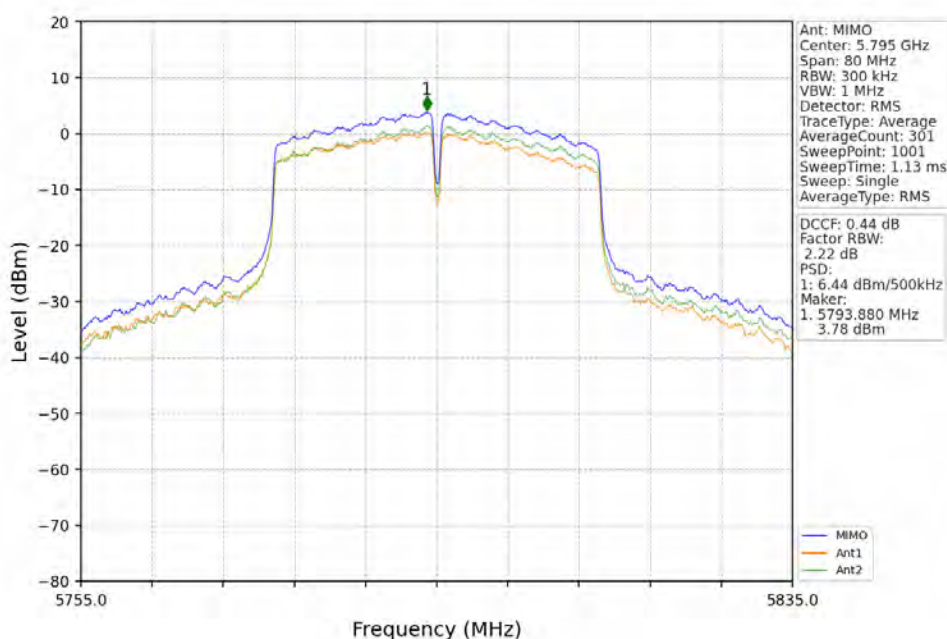
802.11n(HT40)_HCH_5795MHz_MIMO_NTNV
