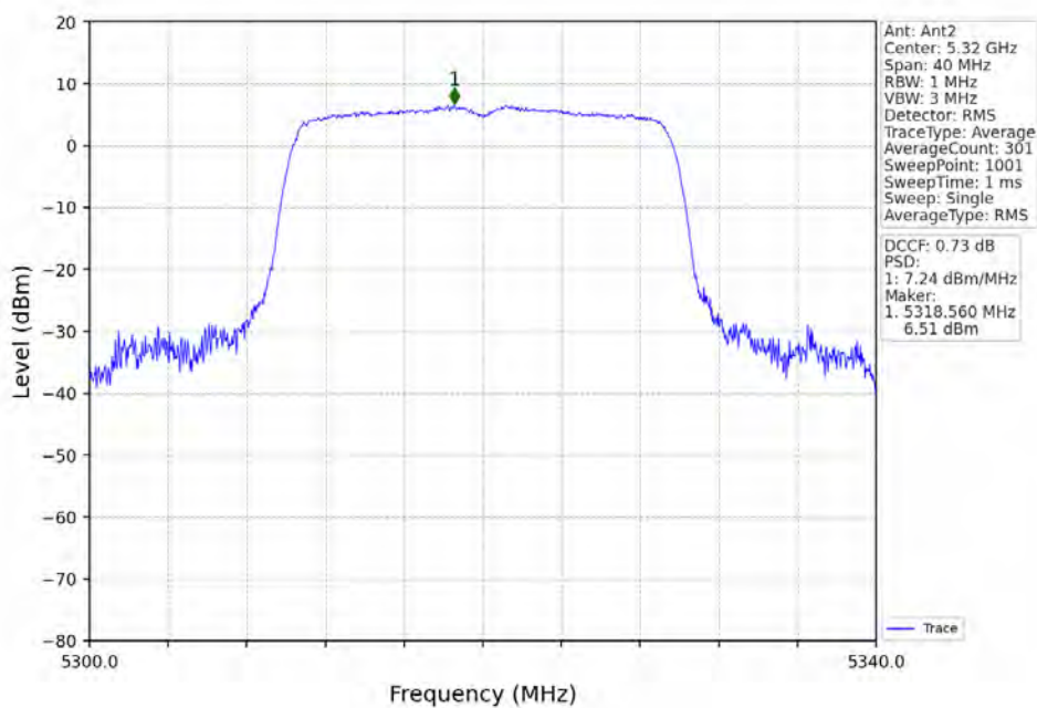
802.11ax(HEW20)_HCH_5320MHz_RU242_Left_Ant2_NTNV
