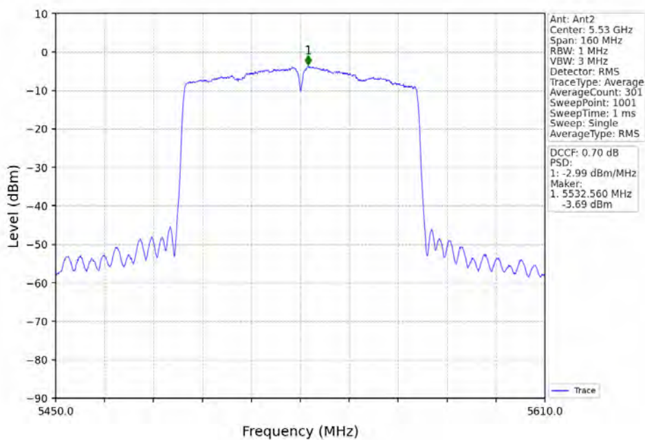
802.11ac(VHT80)_LCH_5530MHz_Ant2_NTNV
