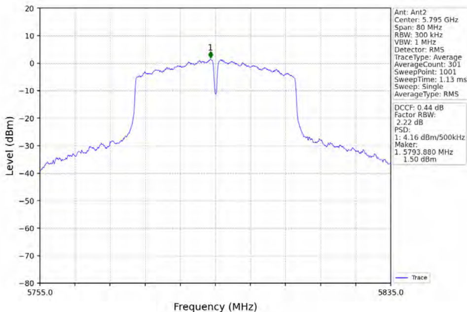
802.11n(HT40)_HCH_5795MHz_MIMO_NTNV
