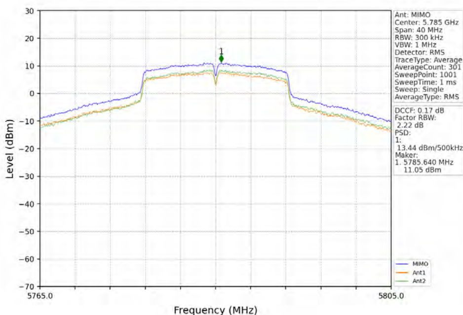
802.11a_MCH_5785MHz_MIMO_NTNV
