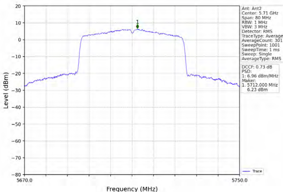
802.11ax(HEW40)_HCH_5710MHz_RU484_Left_Ant2_NTNV
