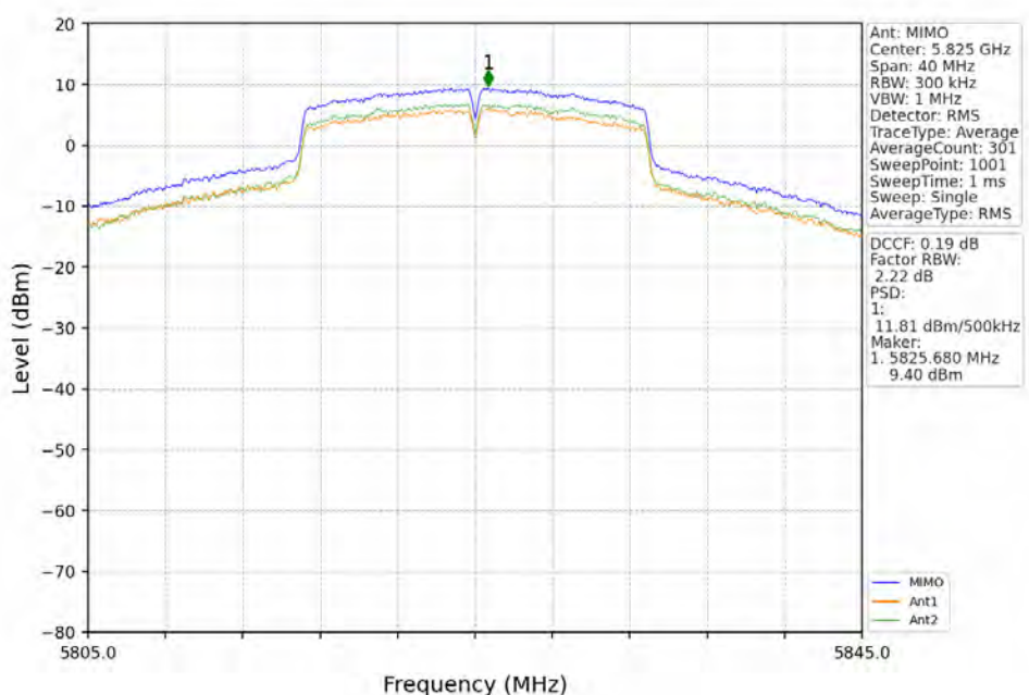
802.11n(HT20)_HCH_5825MHz_MIMO_NTNV
