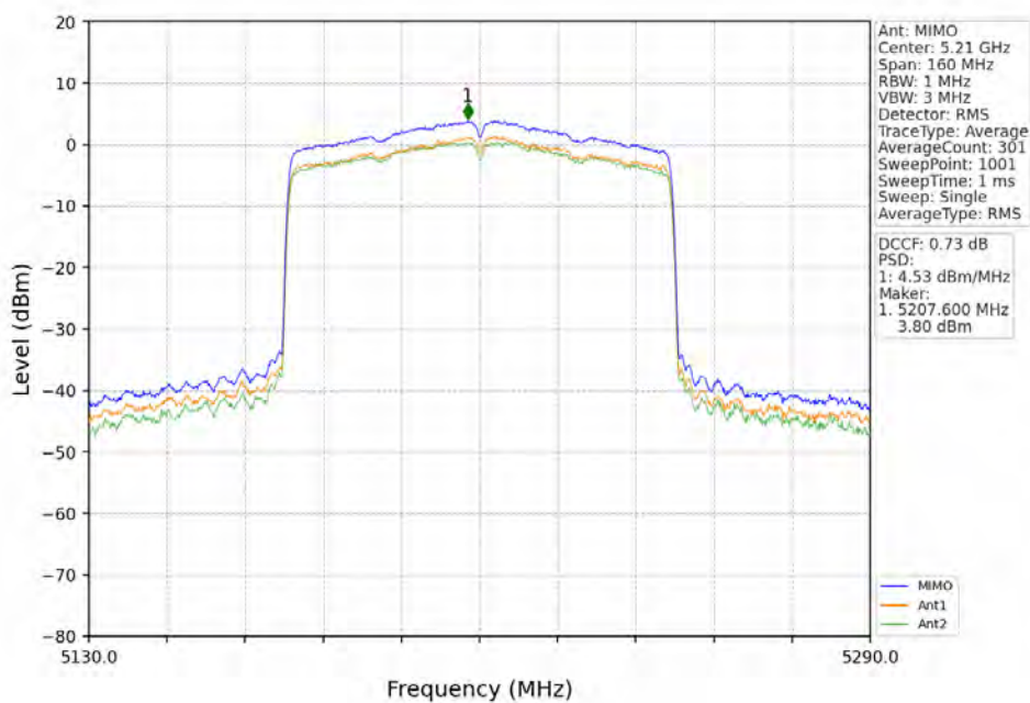
802.11ax(HEW80)_MCH_5210MHz_RU996_Left_MIMO_NTNV
