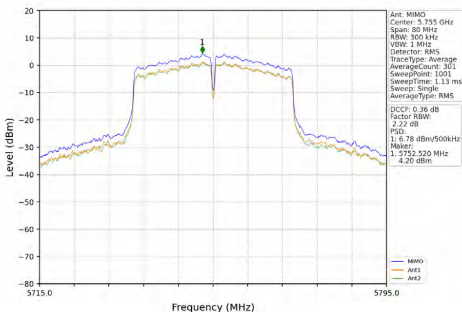
802.11ac(VHT40)_LCH_5755MHz_MIMO_NTNV
