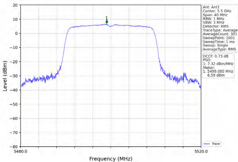
802.11ax(HEW20)_LCH_5500MHz_RU242_Left_Ant1_NTNV
