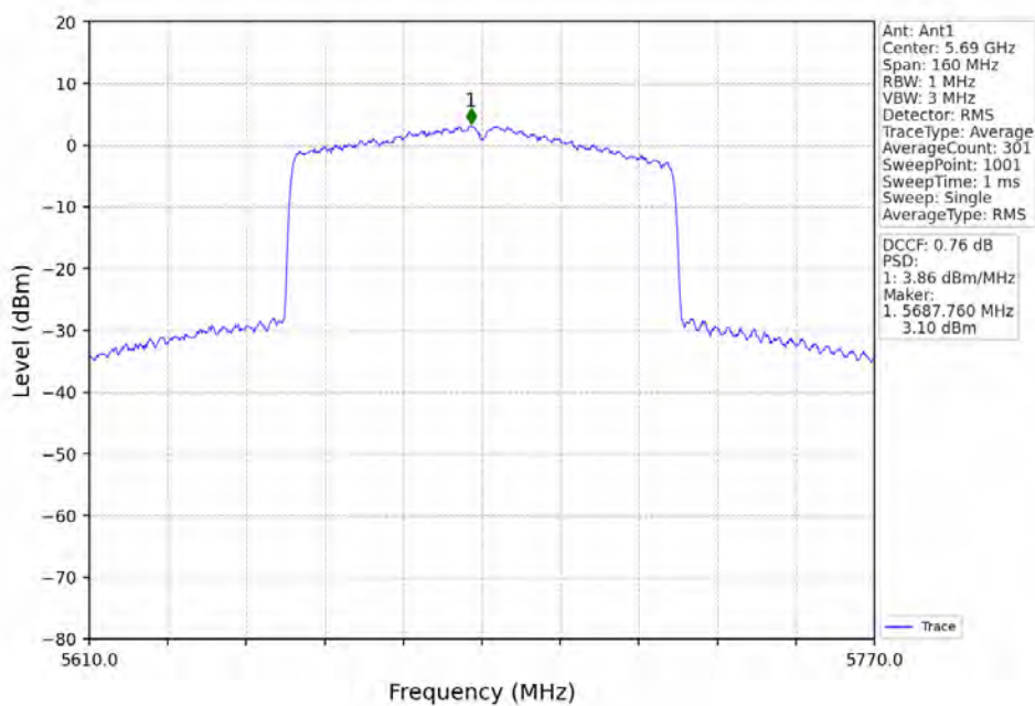
802.11ax(HEW80)_HCH_5690MHz_RU996_Left_Ant1_NTNV
