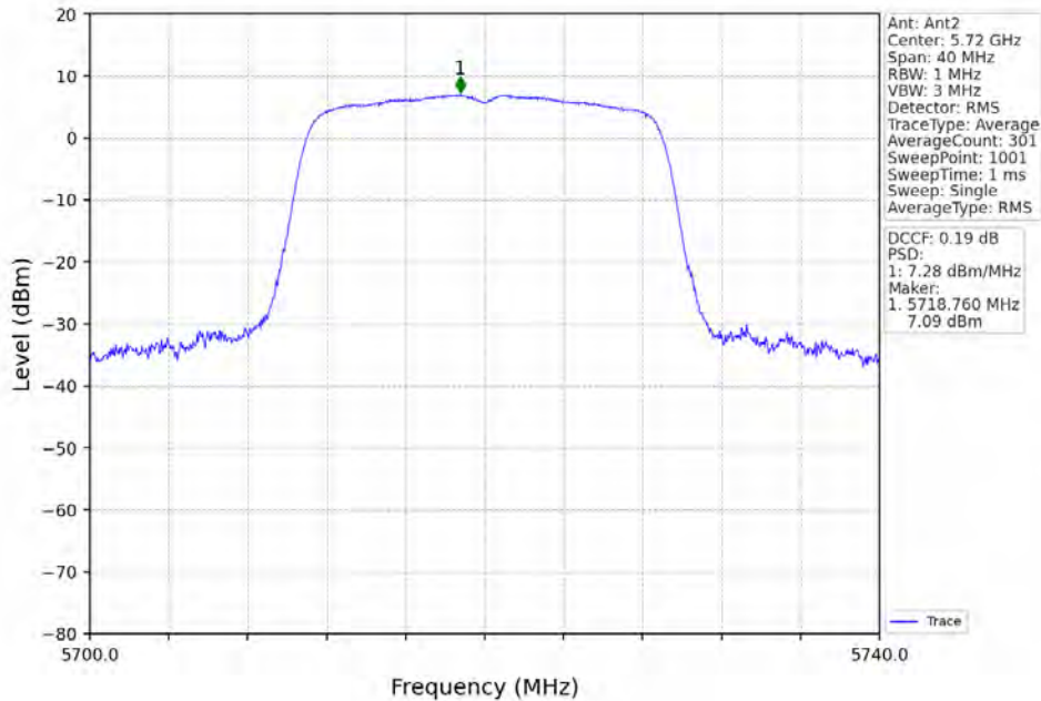
802.11n(HT20)_HCH_5720MHz_MIMO_NTNV
