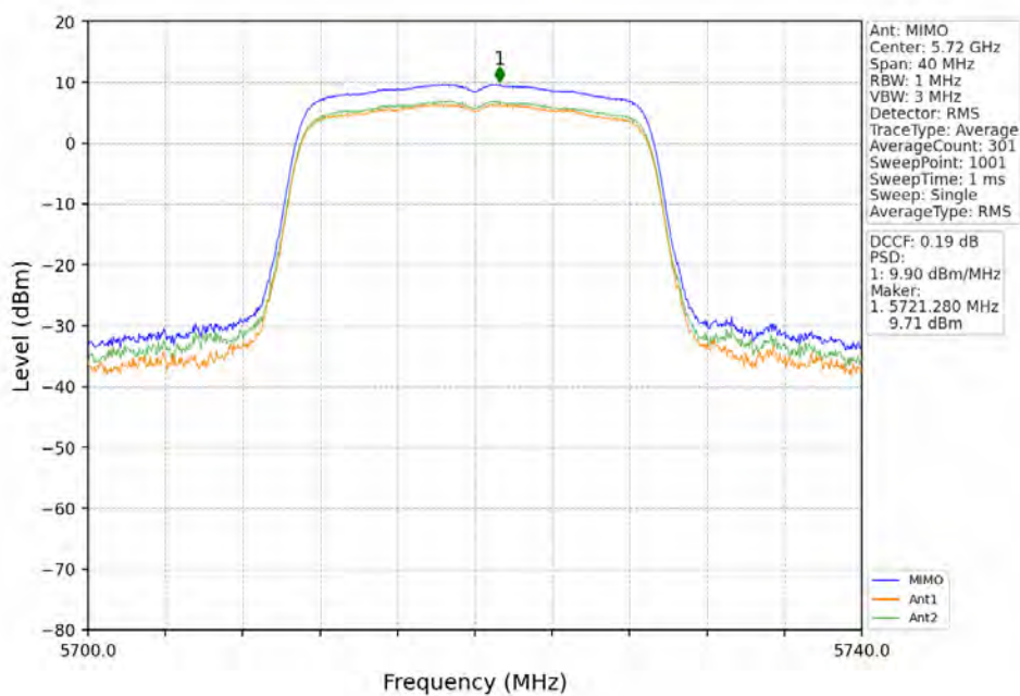
802.11n(HT20)_HCH_5720MHz_MIMO_NTNV
