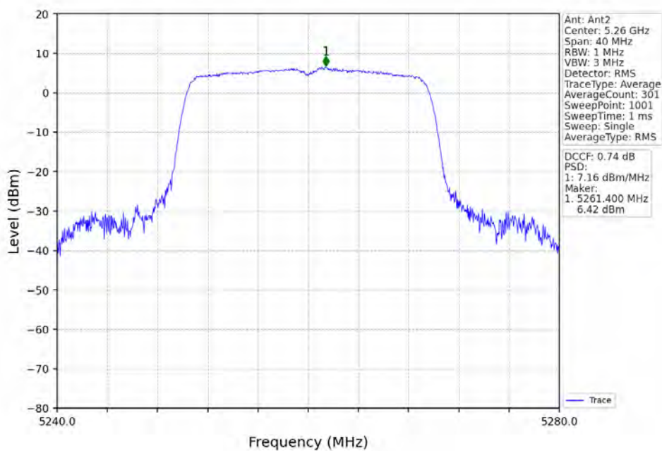
802.11ax(HEW20)_LCH_5260MHz_RU242_Left_Ant2_NTNV
