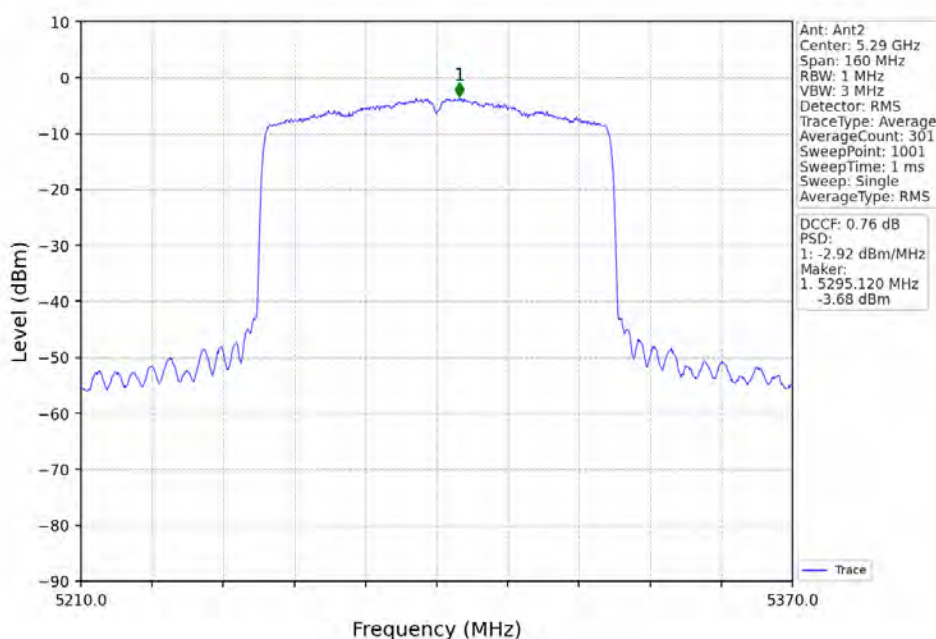
802.11ax(HEW80)_MCH_5290MHz_RU996_Left_Ant2_NTNV
