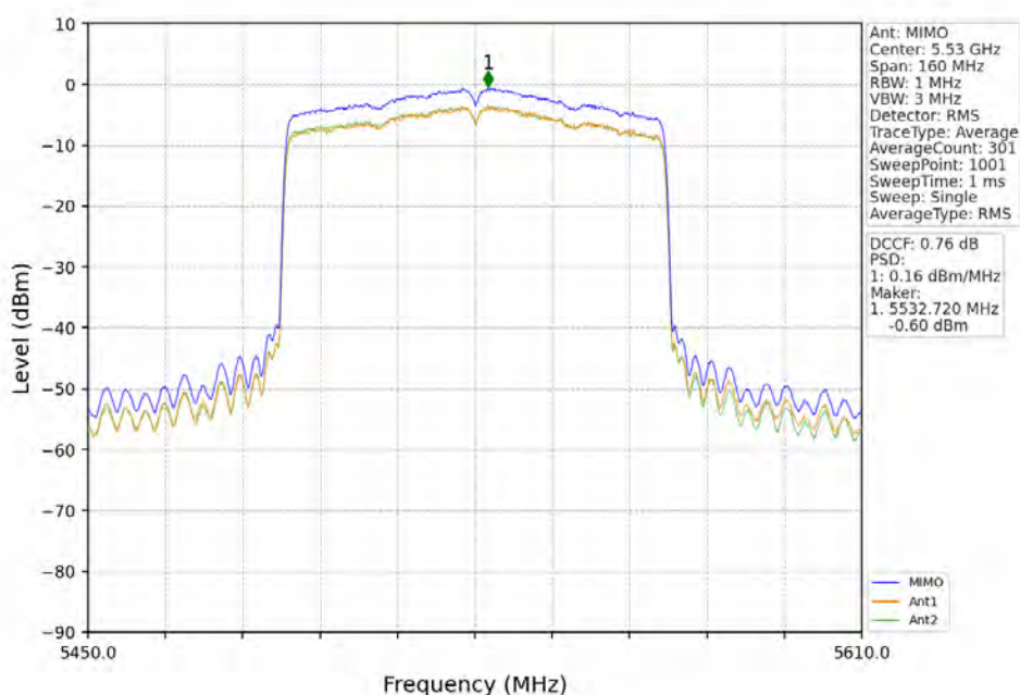
802.11ax(HEW80)_LCH_5530MHz_RU996_Left_MIMO_NTNV
