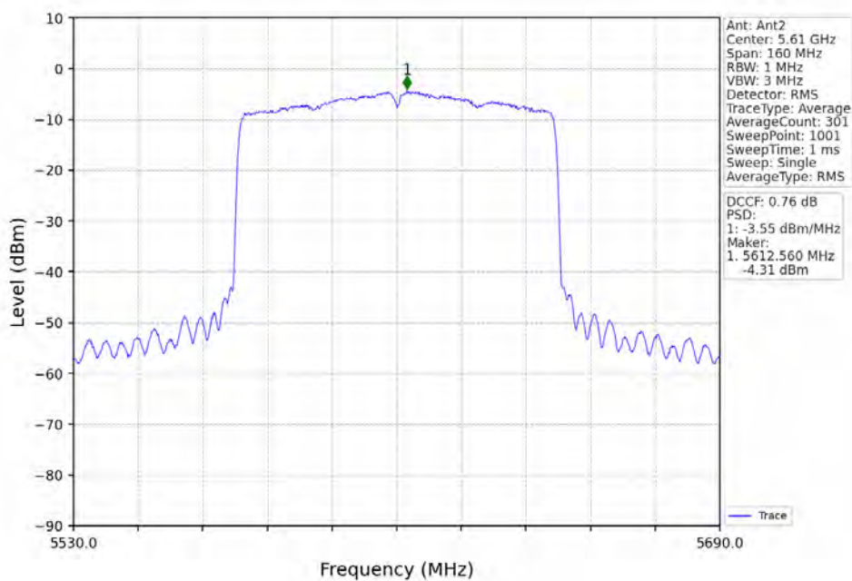
802.11ax(HEW80)_HCH_5610MHz_RU996_Left_Ant2_NTNV
