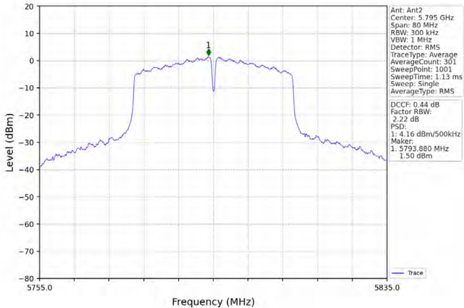
802.11n(HT40)_HCH_5795MHz_MIMO_NTNV
