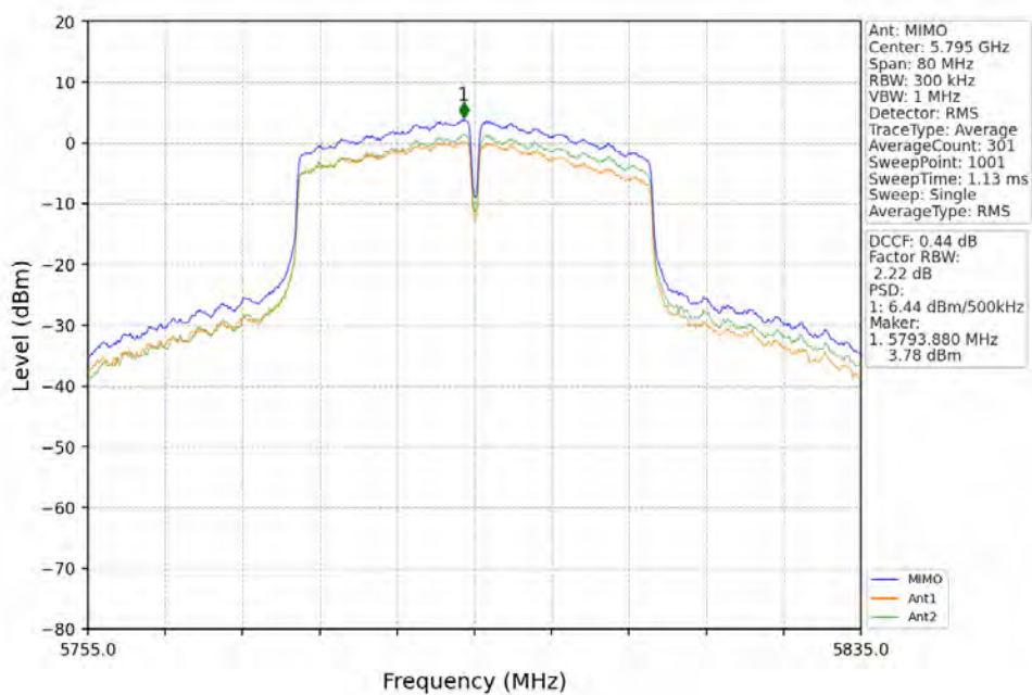
802.11n(HT40)_HCH_5795MHz_MIMO_NTNV
