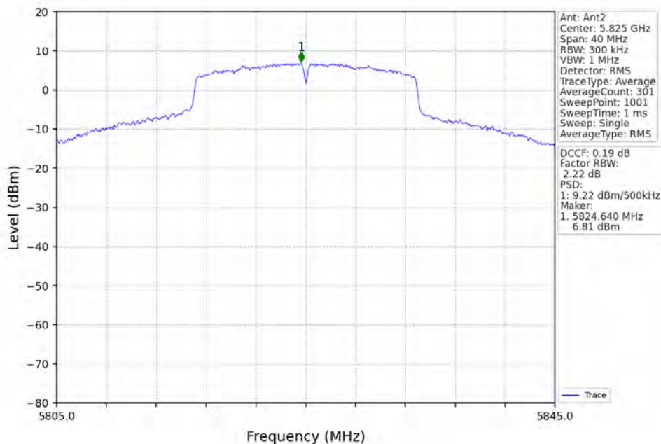
802.11n(HT20)_HCH_5825MHz_MIMO_NTNV
