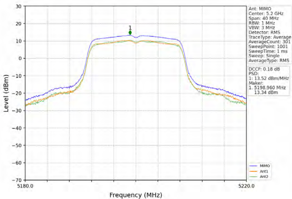
802.11a_MCH_5200MHz_MIMO_NTNV
