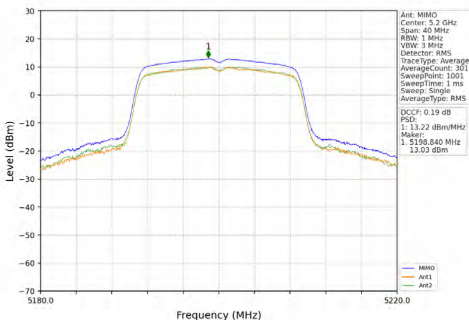
802.11n(HT20)_MCH_5200MHz_MIMO_NTNV
