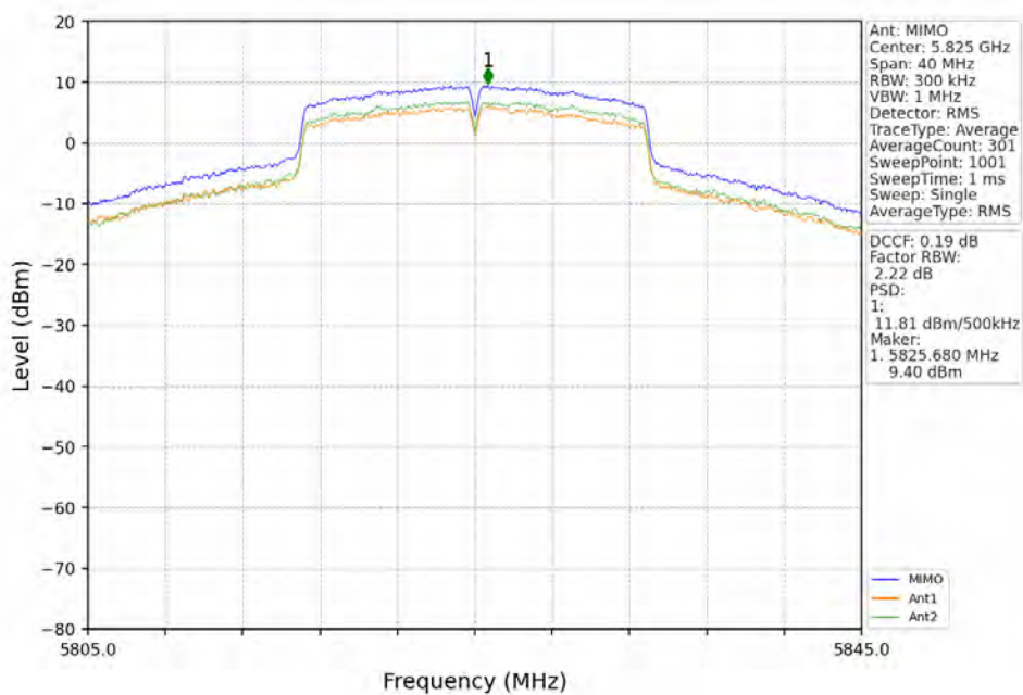
802.11n(HT20)_HCH_5825MHz_MIMO_NTNV
