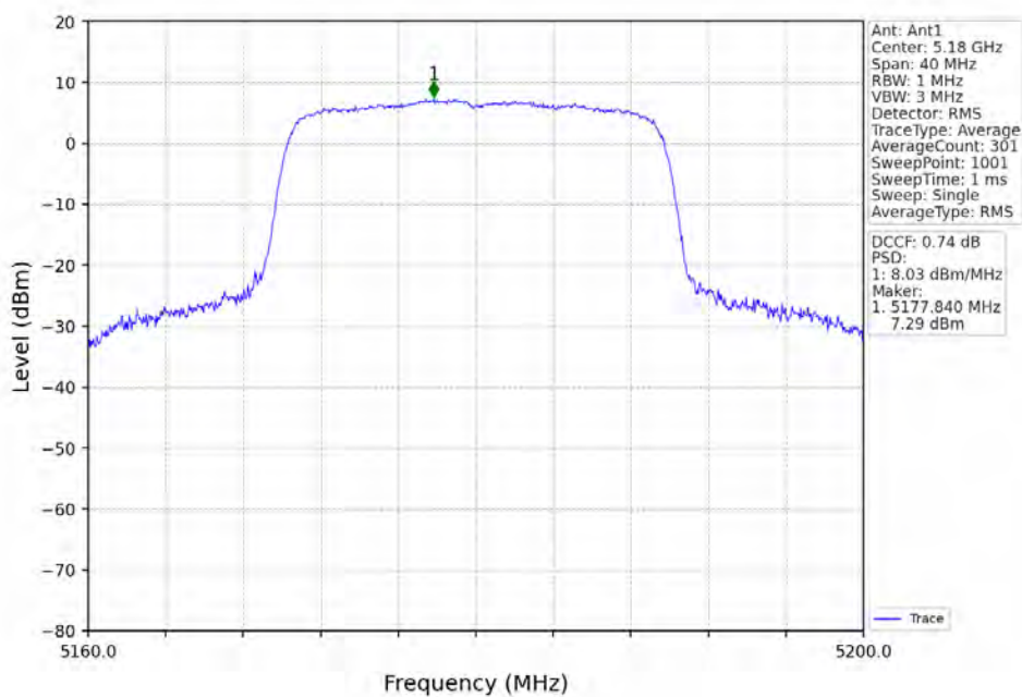
802.11ax(HEW20)_LCH_5180MHz_RU242_Left_Ant1_NTNV
