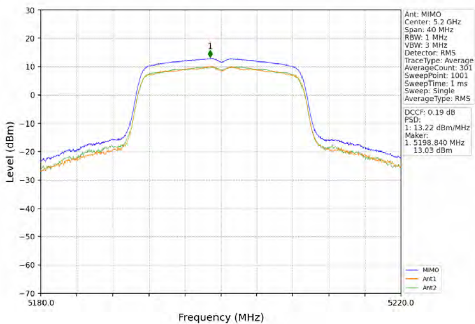
802.11n(HT20)_MCH_5200MHz_MIMO_NTNV
