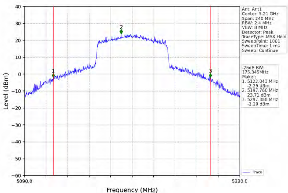
802.11ax(HEW80)_MCH_5210MHz_RU996_Left_Ant1_NTNV
