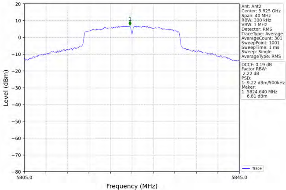
802.11n(HT20)_HCH_5825MHz_MIMO_NTNV
