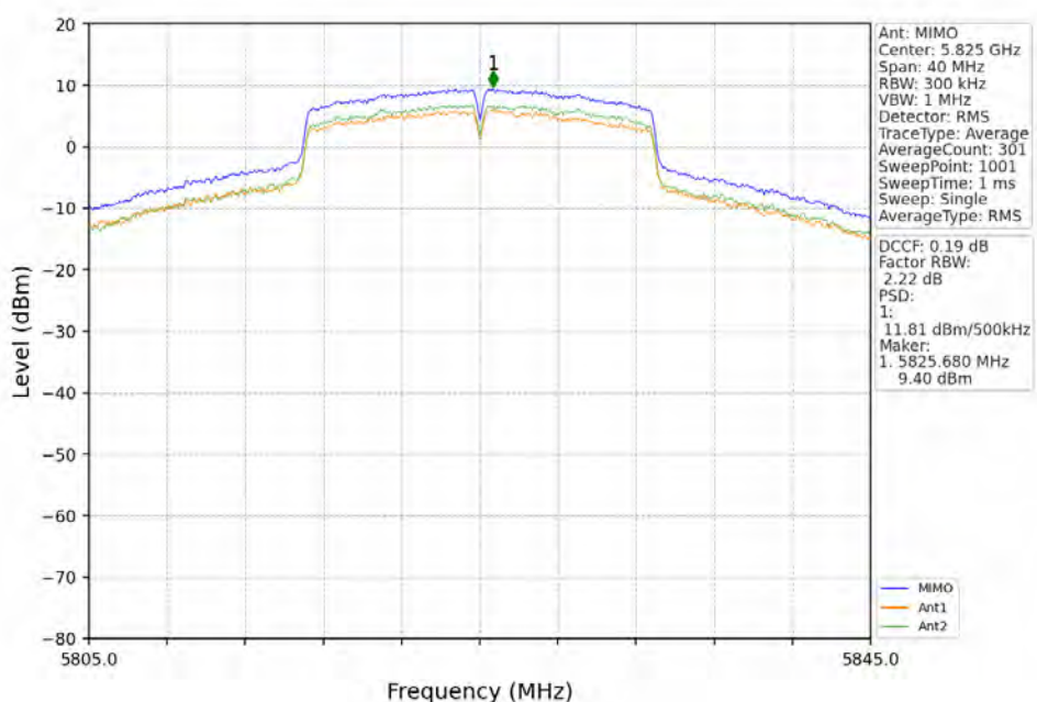
802.11n(HT20)_HCH_5825MHz_MIMO_NTNV
