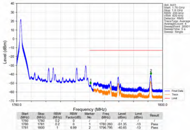
Band66_20MHz_QPSK_HCH_1770MHz_RB_1_99_NTNV
