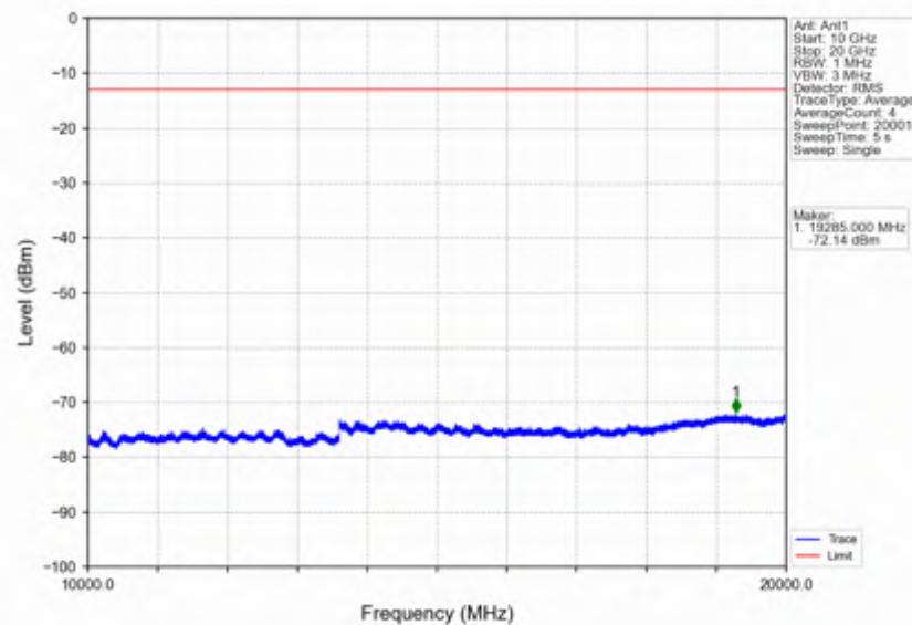
Band66_20MHz_256QAM_LCH_1720MHz_RB_100_0_NTNV
