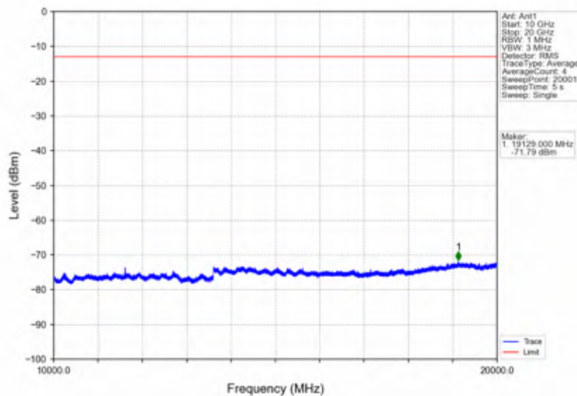
Band66_20MHz_QPSK_HCH_1770MHz_RB_1_0_NTNV
