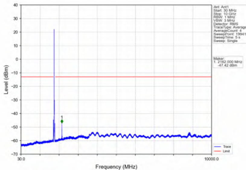
Band66_20MHz_QPSK_HCH_1770MHz_RB_1_0_NTNV
