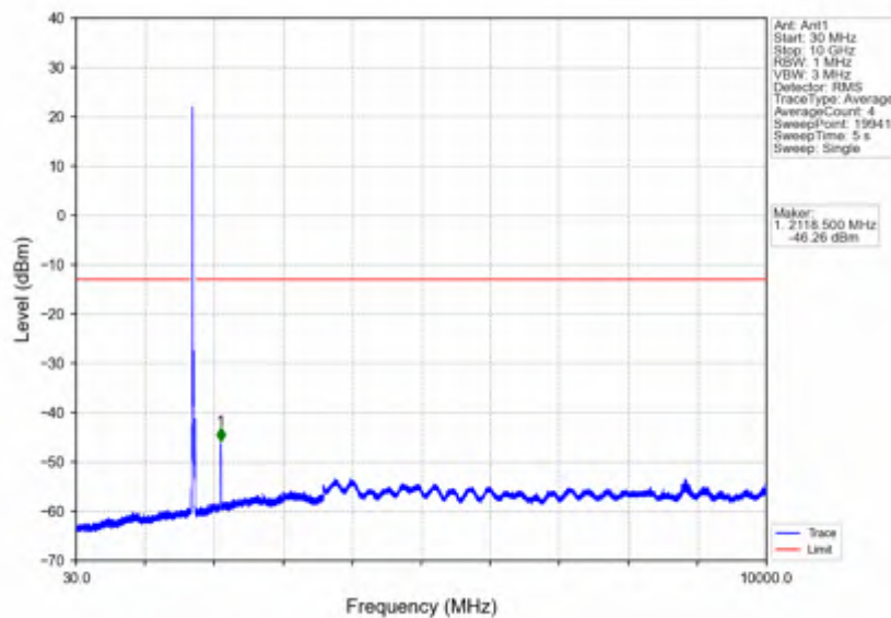
Band66 20MHz 64QAM LCH 1720MHz RB 1 0 NTNV
