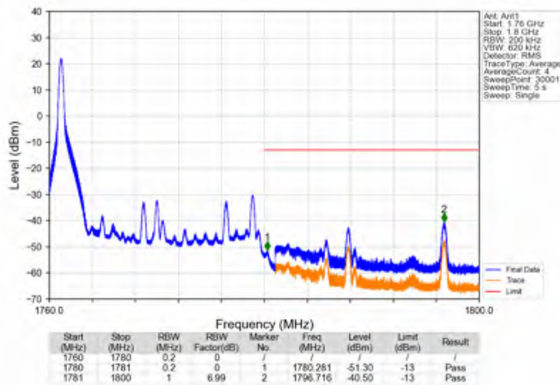
Band66_20MHz_QPSK_HCH_1770MHz_RB_100_0_NTNV
