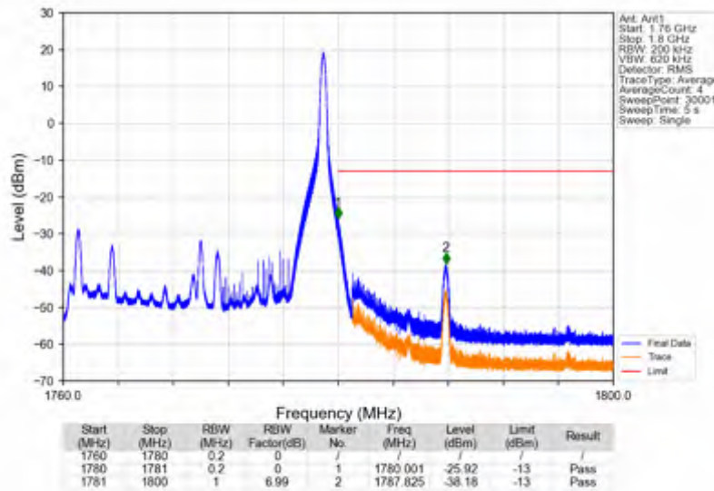
Band66_20MHz_256QAM_HCH_1770MHz_RB_1_99_NTNV
