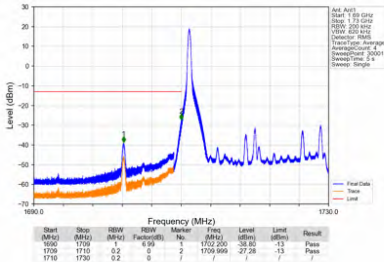
Band66 20MHz 256QAM LCH 1720MHz RB 1 0 NTNV
