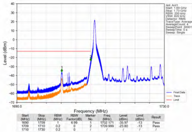
Band66 20MHz QPSK LCH 1720MHz RB 1 0 NTNV
