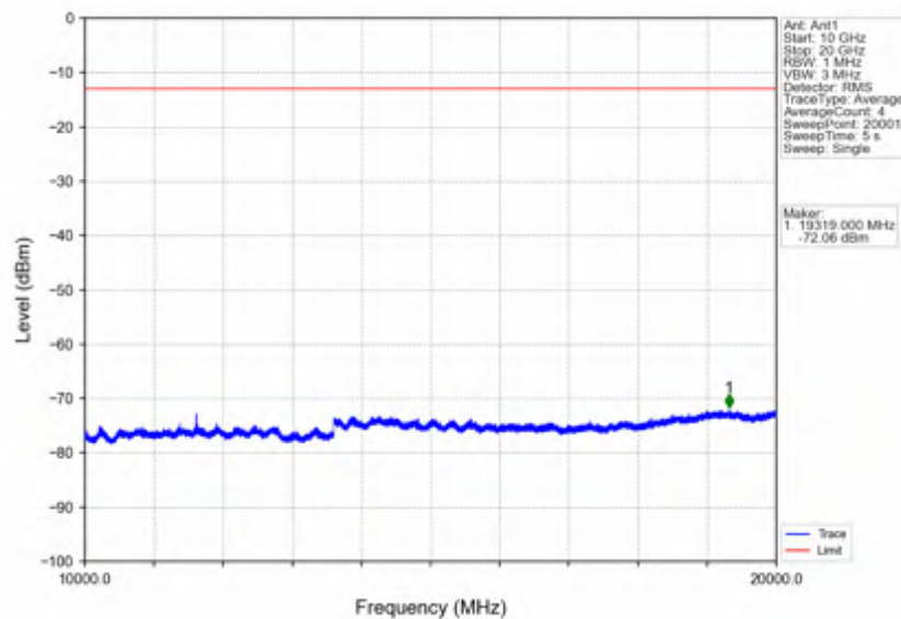
Band66_20MHz_16QAM_LCH_1720MHz_RB_100_0_NTNV
