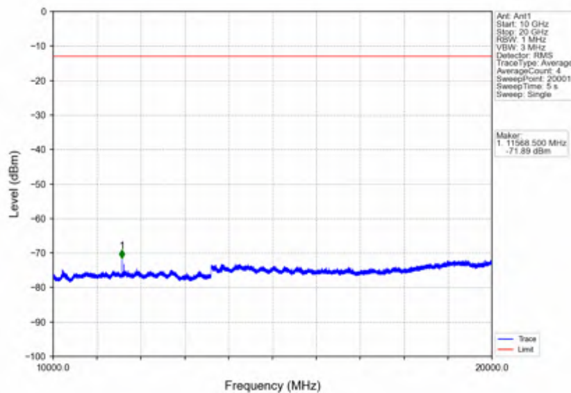
Band66_20MHz_QPSK_MCH_1745MHz_RB_1_0_NTNV
