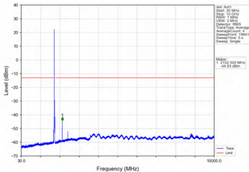
Band66_20MHz_QPSK_MCH_1745MHz_RB_1_0_NTNV
