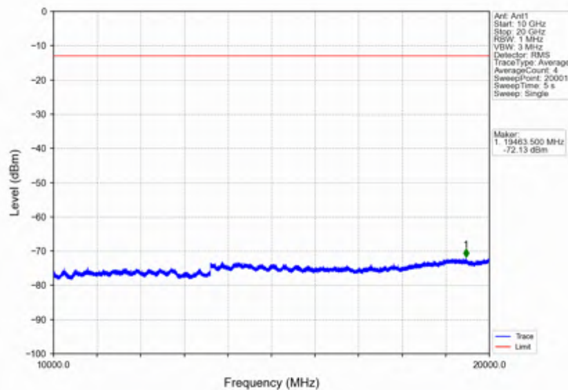
Band66 20MHz QPSK LCH 1720MHz RB 100 0 NTN
