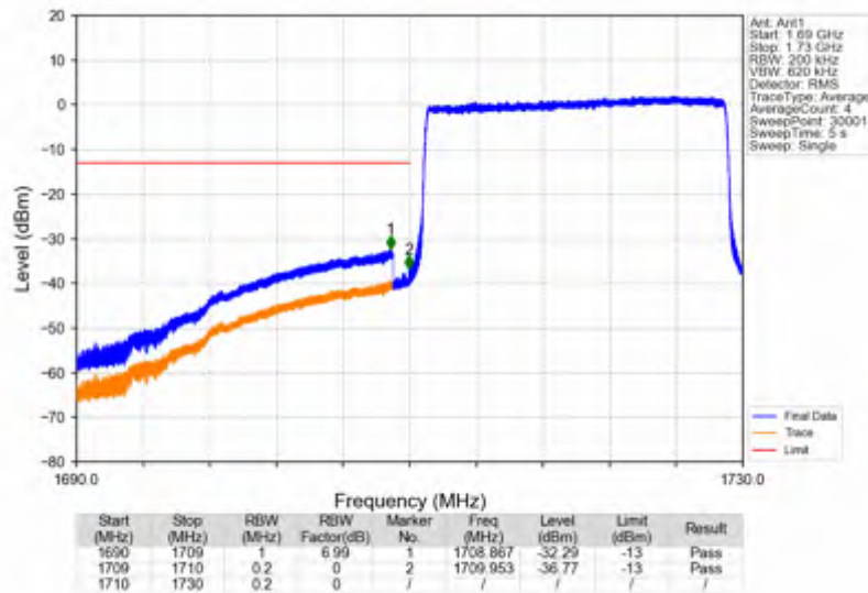
Band66_20MHz_256QAM_LCH_1720MHz_RB_100_0_NTNV
