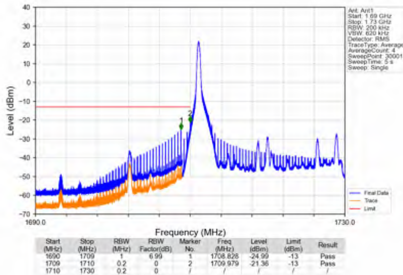
Band66 20MHz 64QAM LCH 1720MHz RB 1 0 NTNV
