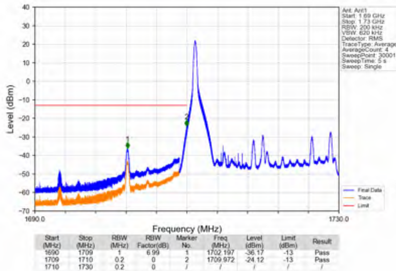
Band66_20MHz_16QAM_LCH_1720MHz_RB_100_0_NTNV
