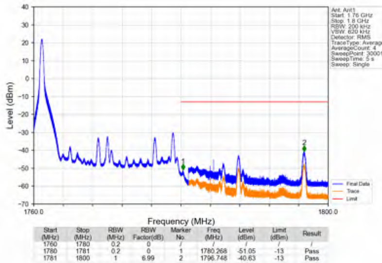
Band66_20MHz_16QAM_HCH_1770MHz_RB_1_99_NTNV
