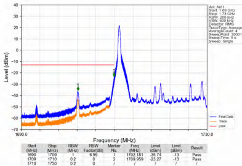
Band66 20MHz QPSK LCH 1720MHz RB 100 0 NTN
