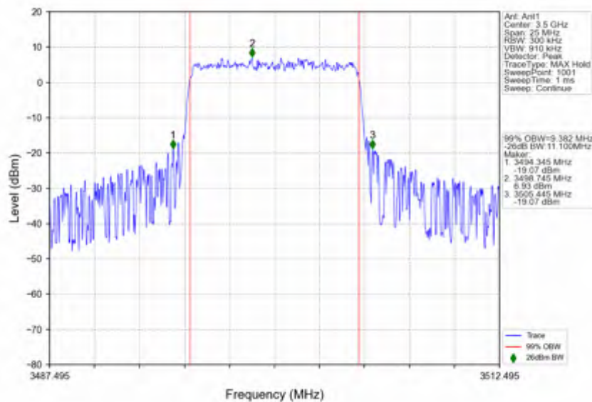
n78e 15kHz SISO NTNV 10MHz CP-OFDM 256 QAM 3499.995MHz Outer Full
