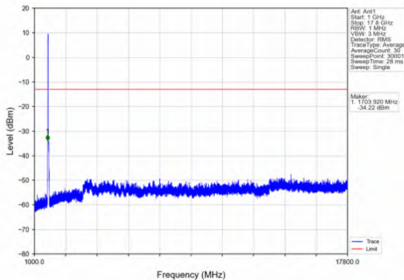
n66_15kHz_SISO_NTNV_30MHz_DFT-s-OFDM QPSK_1725MHz_Inner_1RB_Left
