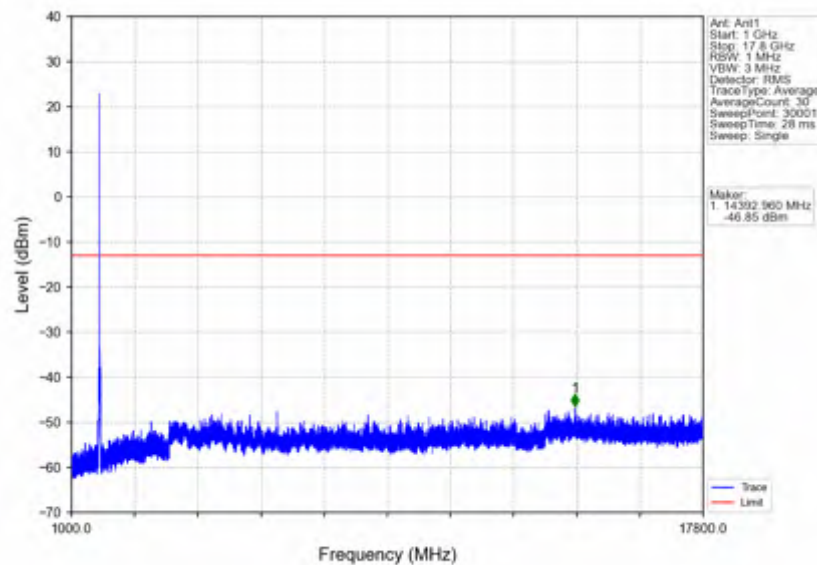
n66_15kHz_SISO_NTNV_20MHz_DFT-s-OFDM_PI/2_BPSK_1745MHz_Edge_1RB_Left
