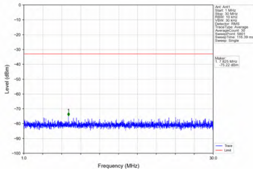
n66_15kHz_SISO_NTNV_20MHz_CP-OFDM QPSK_1770MHz_Inner_1RB_Right
