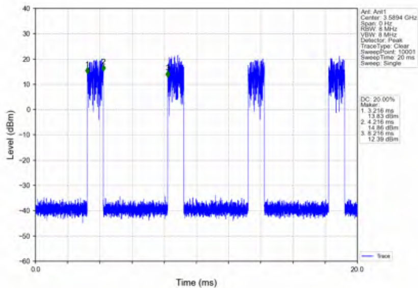
n78d 15kHz SISO NTNV 40MHz CP-OFDM 16 QAM 3570MHz Edge 1RB Right
