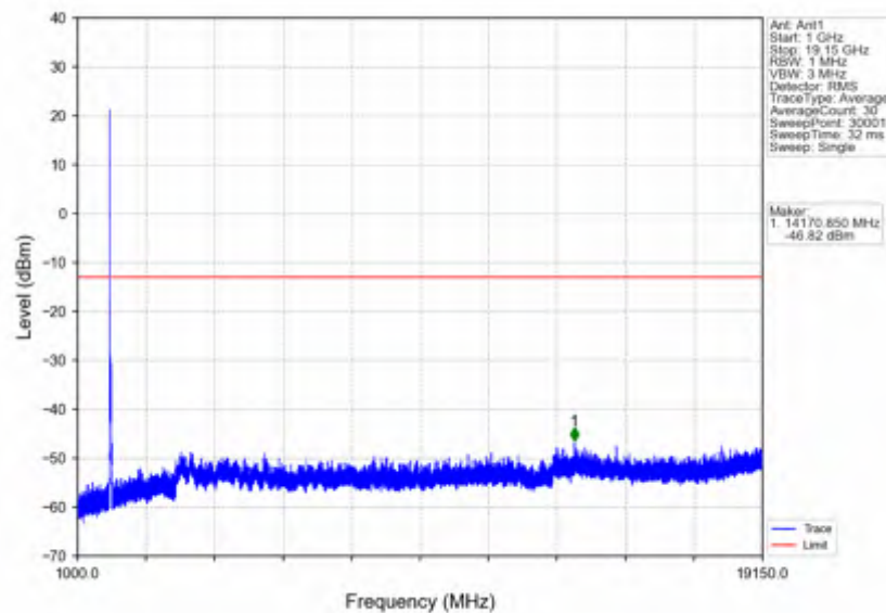
n25 30kHz SISO NTNv 40MHz DFT-s-OFDM QPSK 1870MHz Edge 1RB Left
