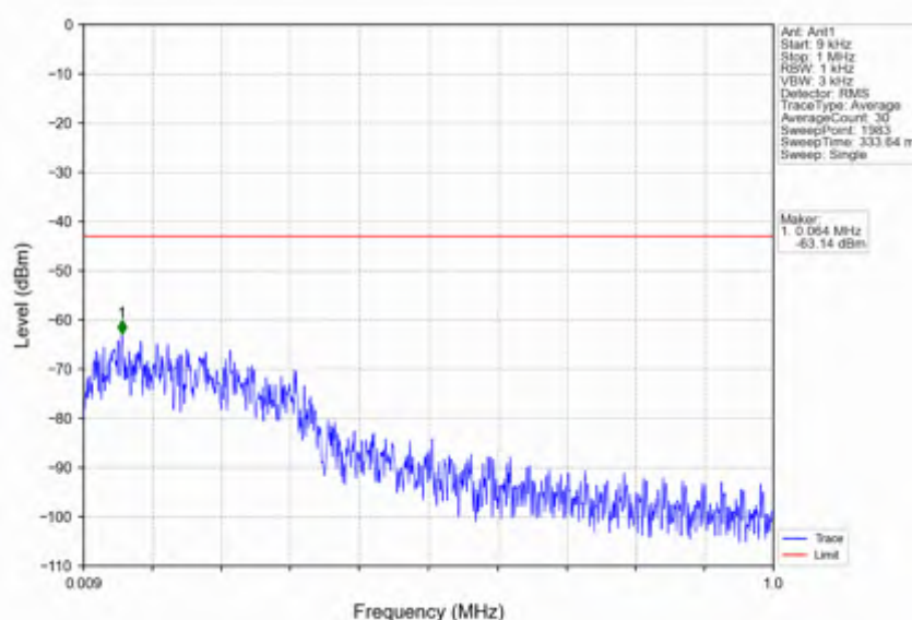
n25 30kHz SISO NTNV 30MHz CP-OFDM QPSK 1900MHz Edge 1RB Right
