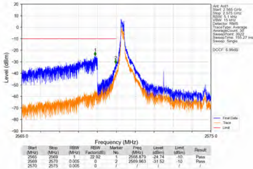
n38 15kHz SISO NTN 5MHz DFT-s-OFDM PI/2 BPSK 2572.5MHz Edge 1RB Left
