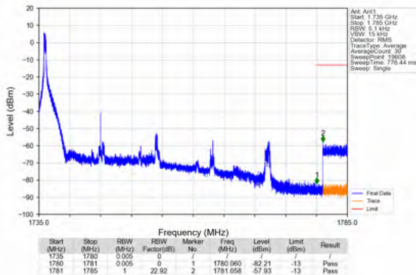
n66_30kHz_SISO_NTNV_20MHz_DFT-s-OFDM PI/2 BPSK_1745MHz_Edge_1RB_Left
