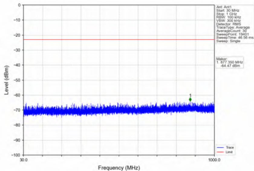
n66 30kHz SISO NTV 10MHz DFT-s-OFDM QPSK 1775MHz Inner 1RB Right
