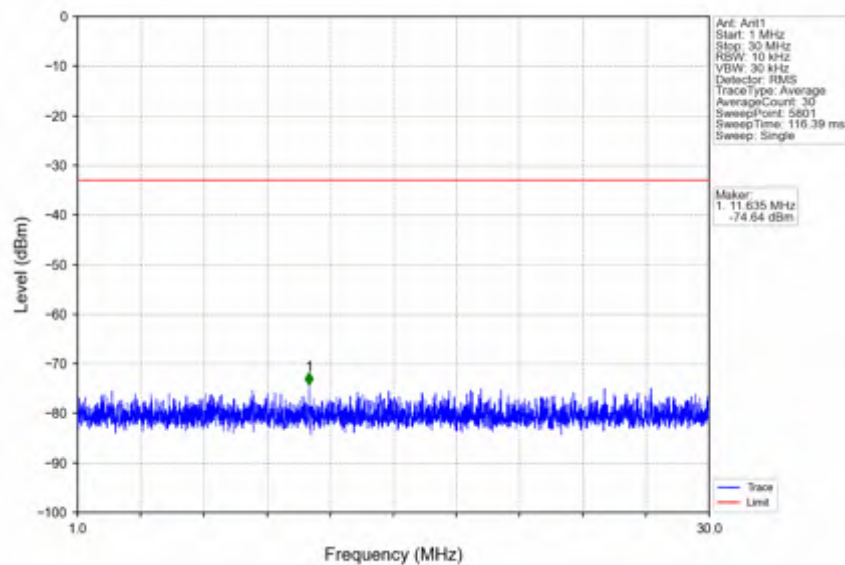
n66_30kHz_SISO_NTNV_20MHz_DFT-s-OFDM PI/2 BPSK_1720MHz_Edge_1RB_Left
