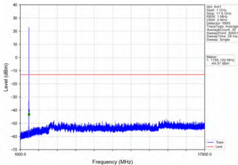
n66 30kHz SISO NTV 10MHz DFT-s-OFDM QPSK 1775MHz Inner 1RB Right
