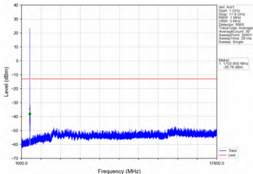
n66_30kHz_SISO_NTNV_20MHz_DFT-s-OFDM PI/2 BPSK_1745MHz_Edge_1RB_Left
