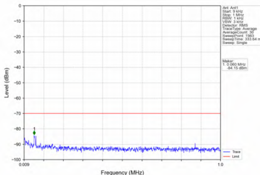
n78d_15kHz_SISO_NTNV_40MHz_DFT-s-OFDM PI/2 BPSK_3570MHz_Inner_1RB_Left
