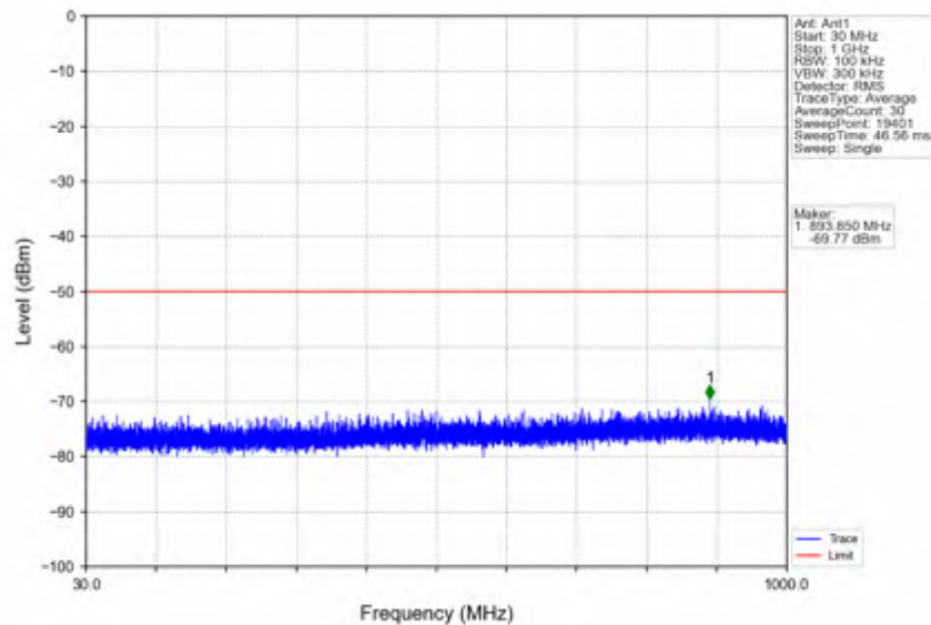
n78d_15kHz_SISO_NTNV_40MHz_CP-OFDM QPSK_3570MHz_Inner_1RB_Left
