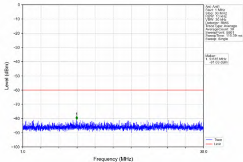
n78d 15kHz SISO NTNv 40MHz CP-OFDM QPSK 3625.005MHz Edge 1RB Left
