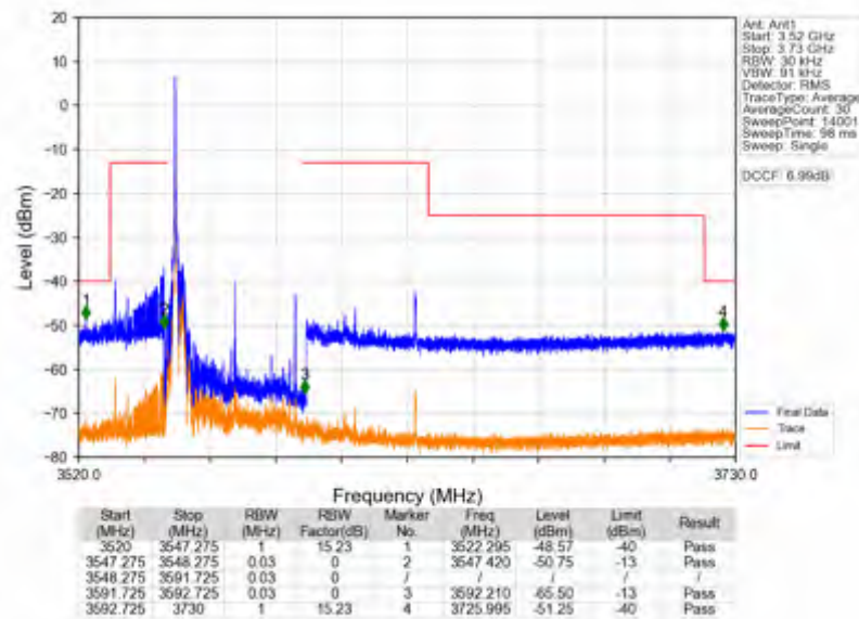
n78d_15kHz_SISO_NTNV_40MHz_DFT-s-OFDM PI/2 BPSK_3570MHz_Inner_1RB_Left
