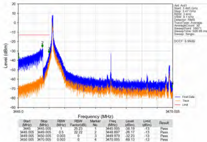
n78e_15kHz_SISO_NTNV_20MHz_DFT-s-OFDM_PI/2_BPSK_3460.005MHz_Edge_1RB_Left
