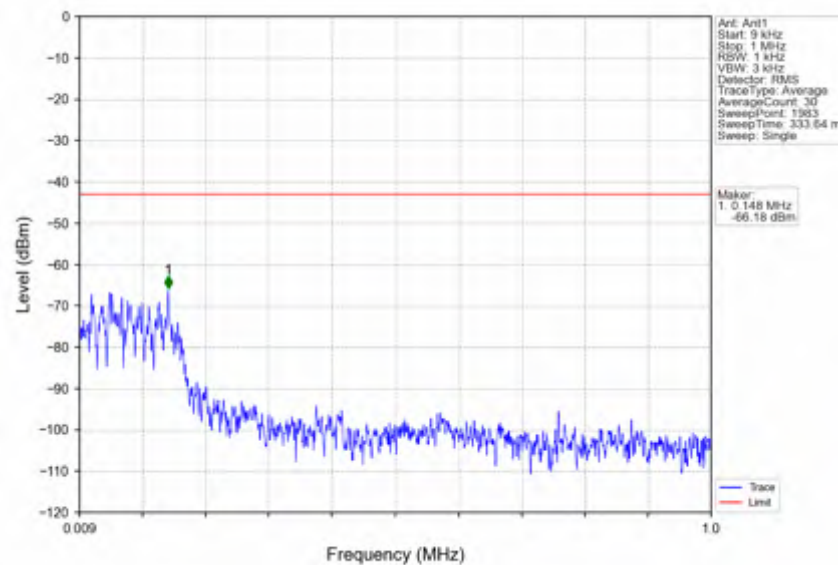
n78e_15kHz_SISO_NTNV_20MHz_DFT-s-OFDM QPSK_3499.995MHz_Edge_1RB_Left
