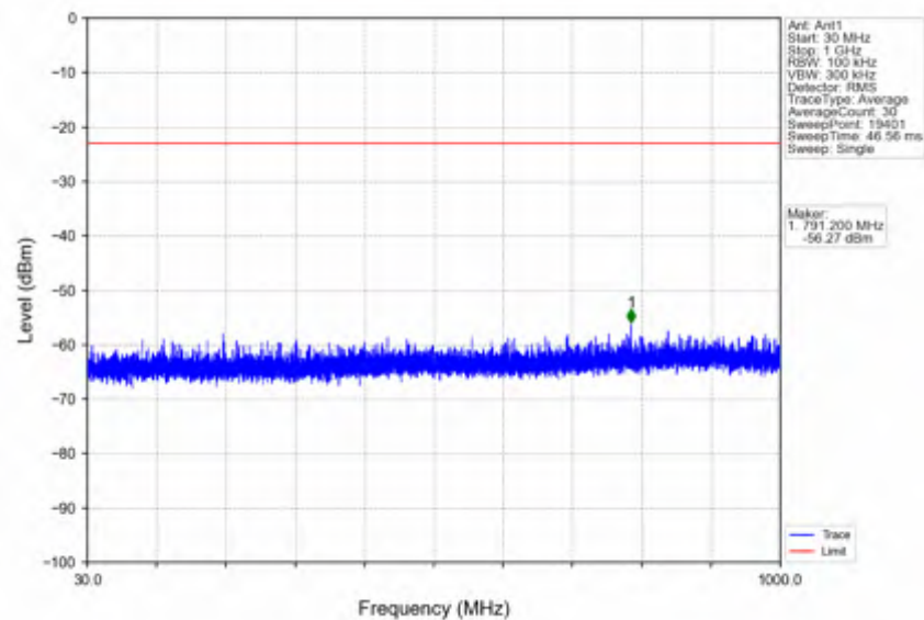
n78e_15kHz_SISO_NTNV_20MHz_DFT-s-OFDM QPSK_3499.995MHz_Edge_1RB_Left
