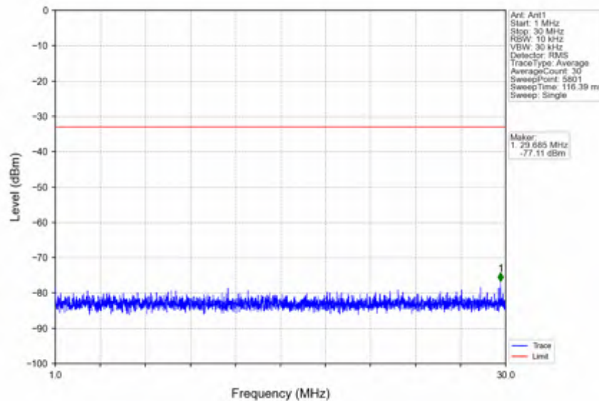
n78e_15kHz_SISO_NTNV_30MHz_CP-OFDM QPSK_3465MHz_Inner_1RB_Left
