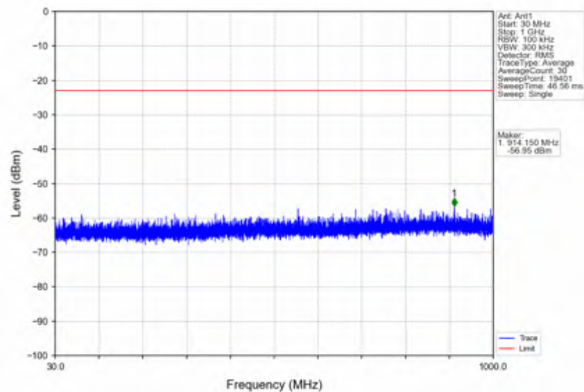
n78e_15kHz_SISO_NTNV_30MHz_CP-OFDM QPSK_3499.995MHz_Edge_1RB_Left
