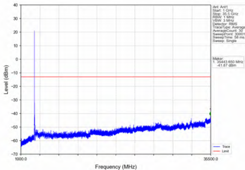
n78e_15kHz_SISO_NTV_30MHz_CP-OFDM QPSK_3499.995MHz_Edge_1RB_Left
