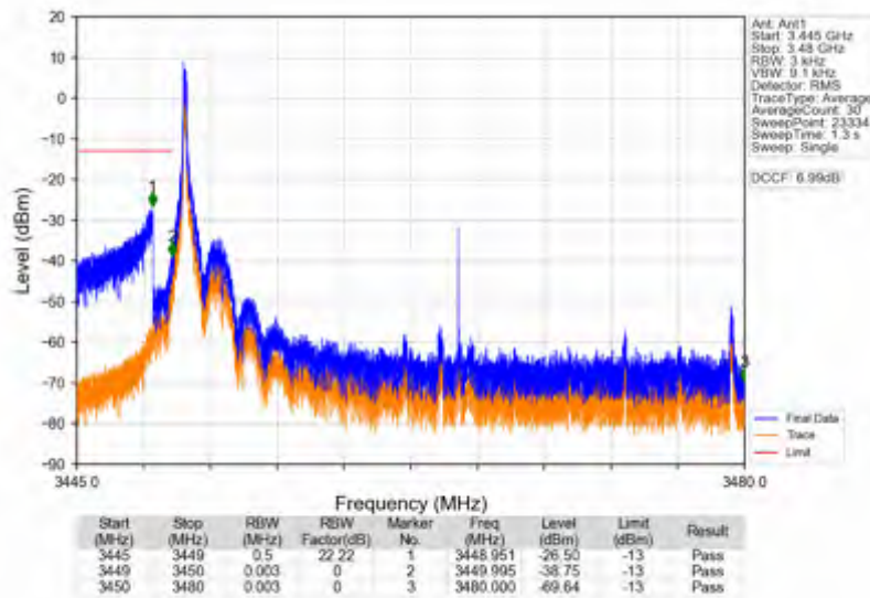
n78e_15kHz_SISO_NTNV_30MHz_DFT-s-OFDM_PI/2_BPSK_3465MHz_Edge_1RB_Left
