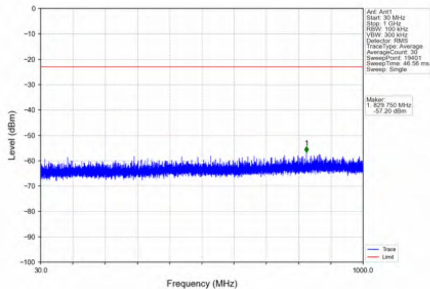
n78e_15kHz_SISO_NTNV_20MHz_CP-OFDM QPSK_3499.995MHz_Edge_1RB_Left
