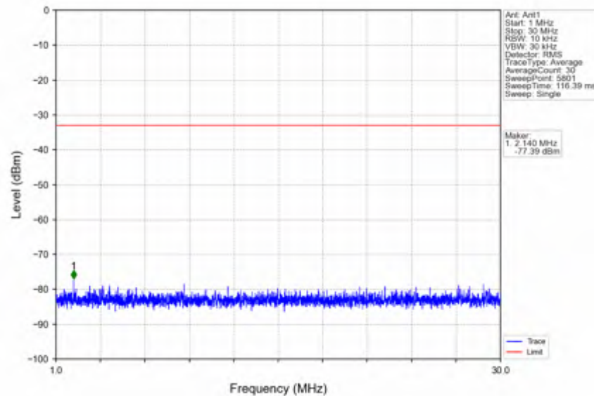
n78e_15kHz_SISO_NTNV_20MHz_CP-OFDM_QPSK_3460.005MHz_Inner_1RB_Left
