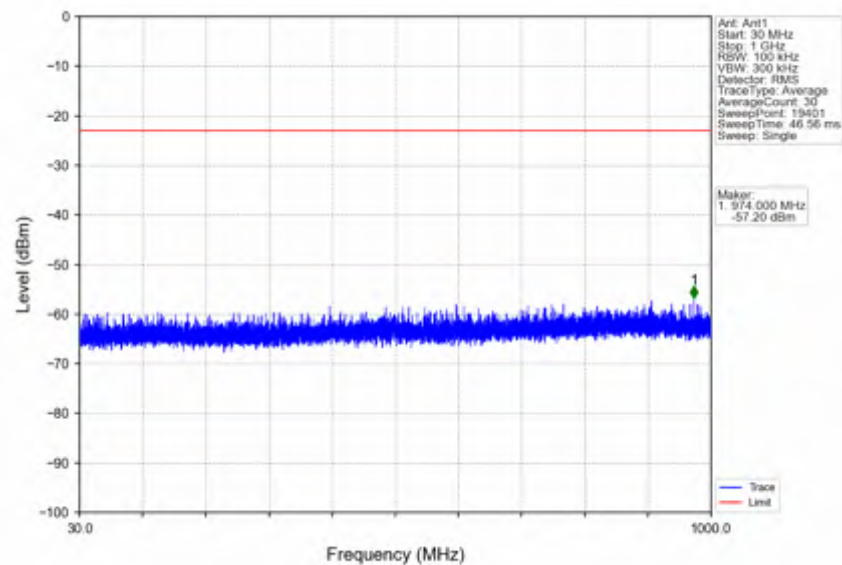
n78e_15kHz_SISO_NTNV_30MHz_DFT-s-OFDM QPSK_3465MHz_Edge_1RB_Left
