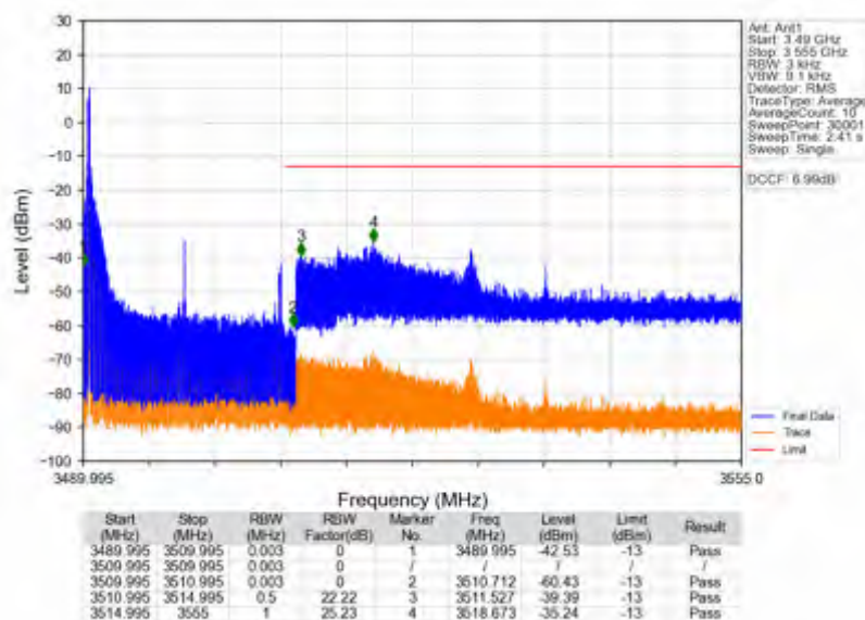
n78e_15kHz_SISO_NTNV_20MHz_CP-OFDM QPSK_3499.995MHz_Edge_1RB_Left
