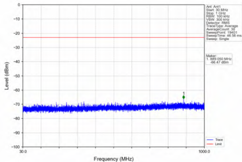
n78e_15kHz_SISO_NTNV_20MHz_DFT-s-OFDM QPSK_3460.005MHz_Inner_1RB_Left
