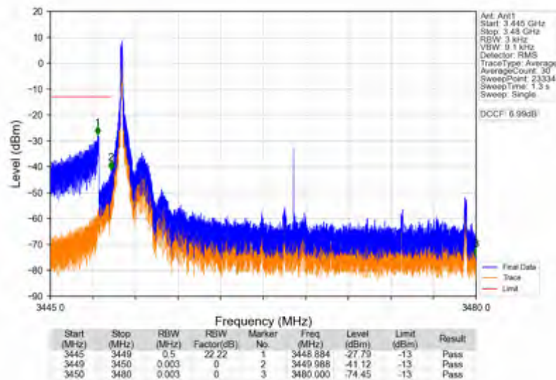
n78e_15kHz_SISO_NTNV_30MHz_DFT-s-OFDM_QPSK_3465MHz_Inner_1RB_Left
