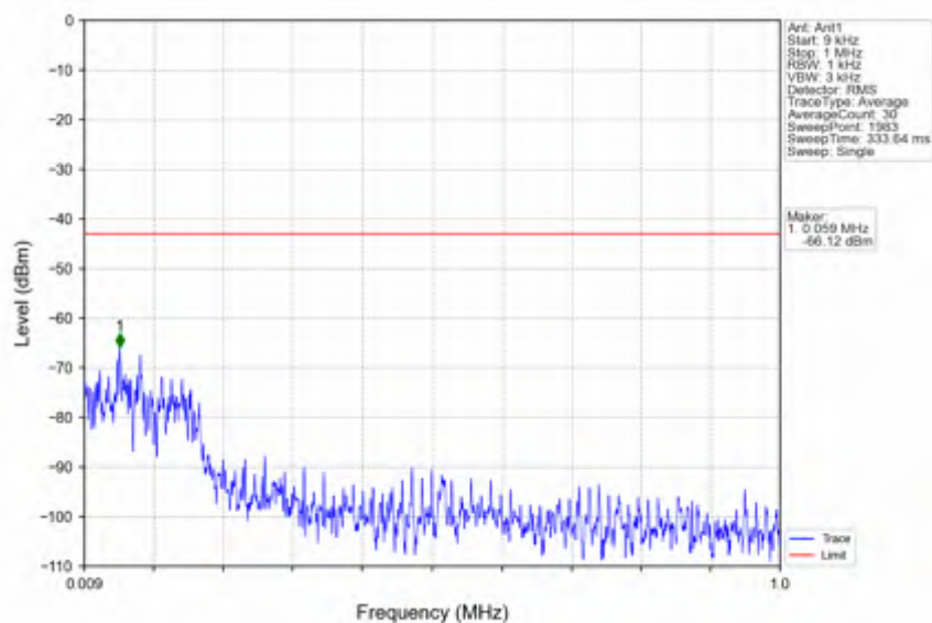
n78e_15kHz_SISO_NTNV_30MHz_DFT-s-OFDM_PI/2_BPSK_3465MHz_Edge_1RB_Left
