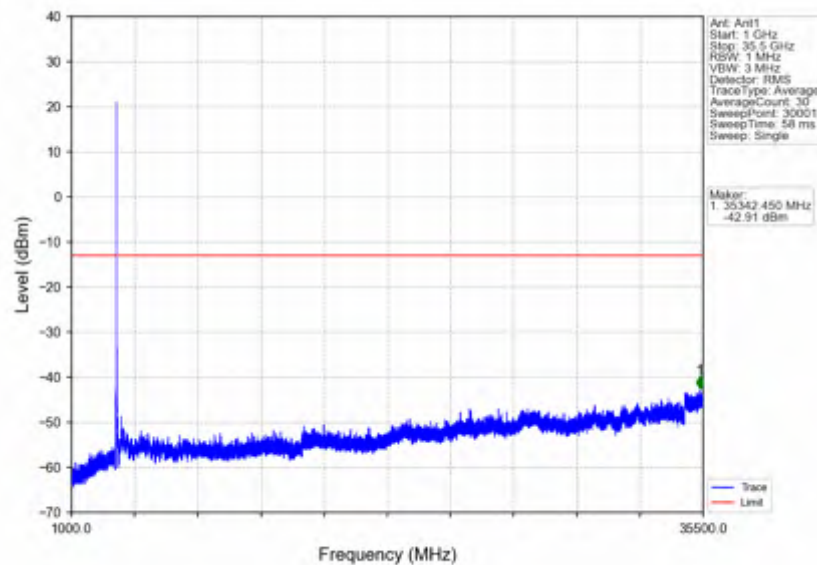
n78e_15kHz_SISO_NTNV_30MHz_DFT-s-OFDM QPSK_3465MHz_Edge_1RB_Left
