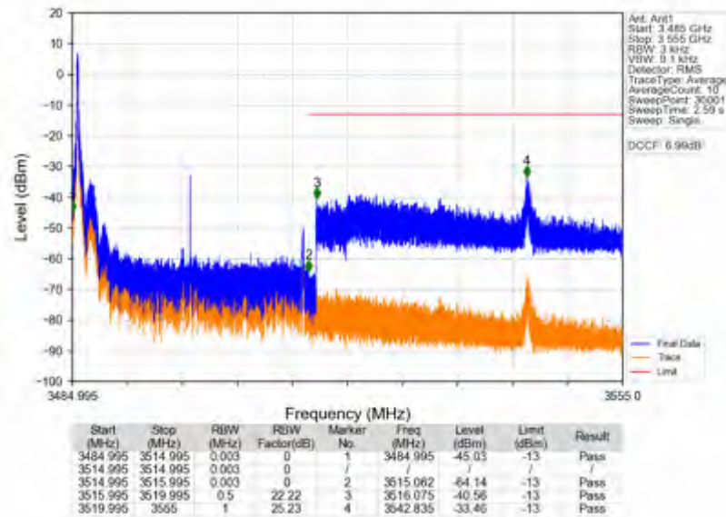
n78e_15kHz_SISO_NTV_30MHz_CP-OFDM QPSK_3499.995MHz_Edge_1RB_Left
