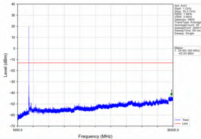
n78e_15kHz_SISO_NTNV_30MHz_CP-OFDM QPSK_3499.995MHz_Edge_1RB_Left
