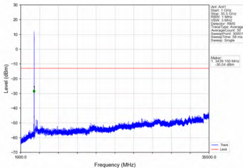
n78e_15kHz_SISO_NTNV_20MHz_DFT-s-OFDM QPSK_3460.005MHz_Inner_1RB_Left
