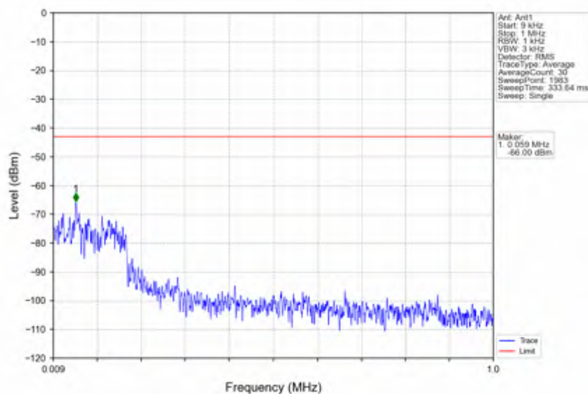
n78e_15kHz_SISO_NTNV_20MHz_DFT-s-OFDM_PI/2_BPSK_3460.005MHz_Edge_1RB_Left
