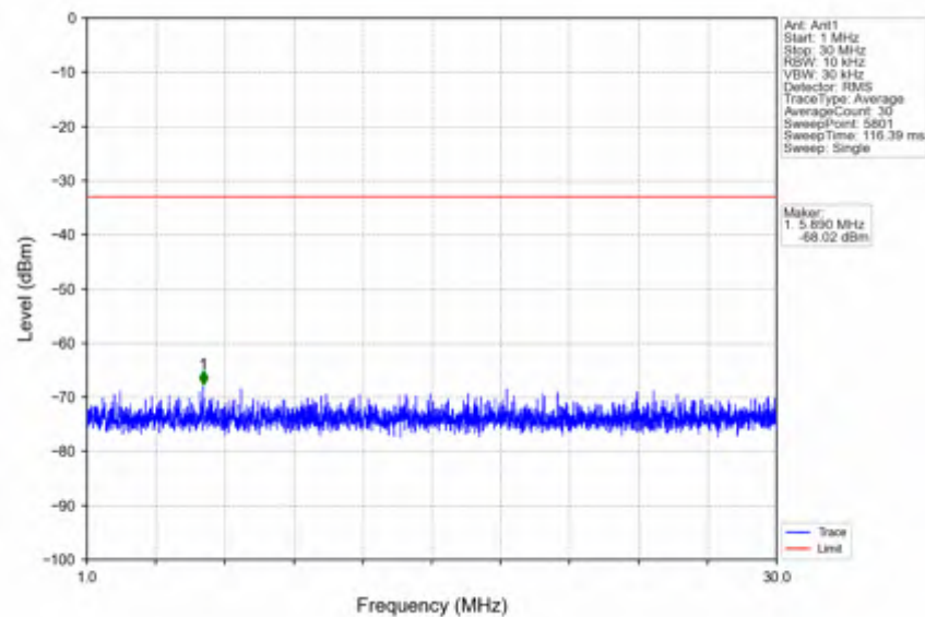
n78e_15kHz_SISO_NTNV_20MHz_DFT-s-OFDM QPSK_3499.995MHz_Edge_1RB_Left
