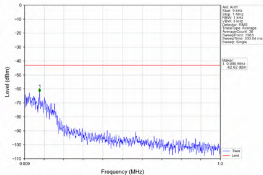
n78e_15kHz_SISO_NTNV_20MHz_CP-OFDM_QPSK_3499.995MHz_Edge_1RB_Left
