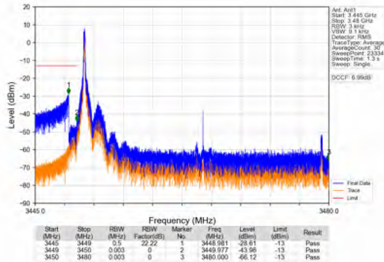
n78e_15kHz_SISO_NTNV_30MHz_CP-OFDM_QPSK_3465MHz_Inner_1RB_Left
