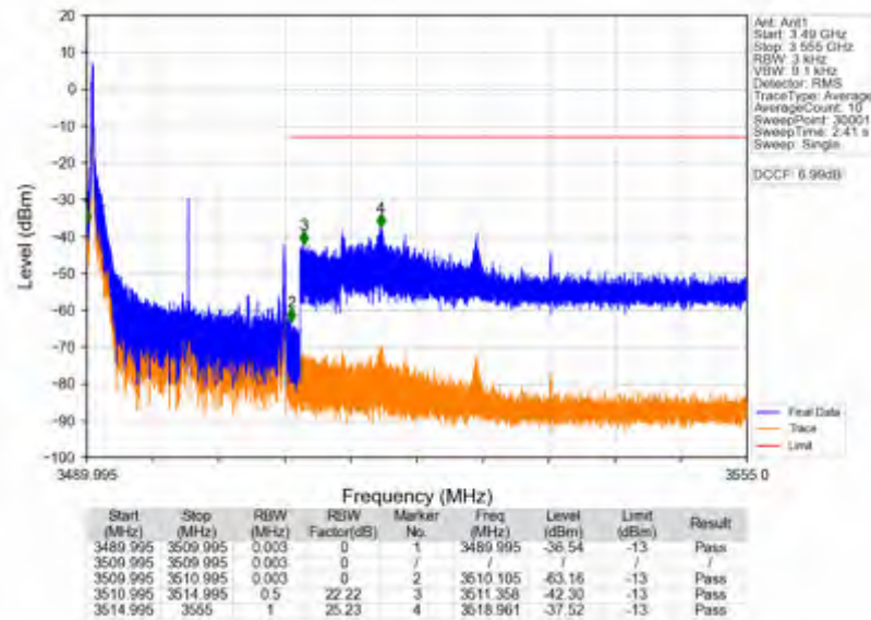
n78e_15kHz_SISO_NTNV_20MHz_DFT-s-OFDM QPSK_3499.995MHz_Edge_1RB_Left
