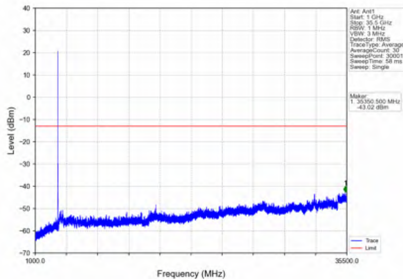
n78e_15kHz_SISO_NTNV_20MHz_CP-OFDM QPSK_3499.995MHz_Edge_1RB_Left
