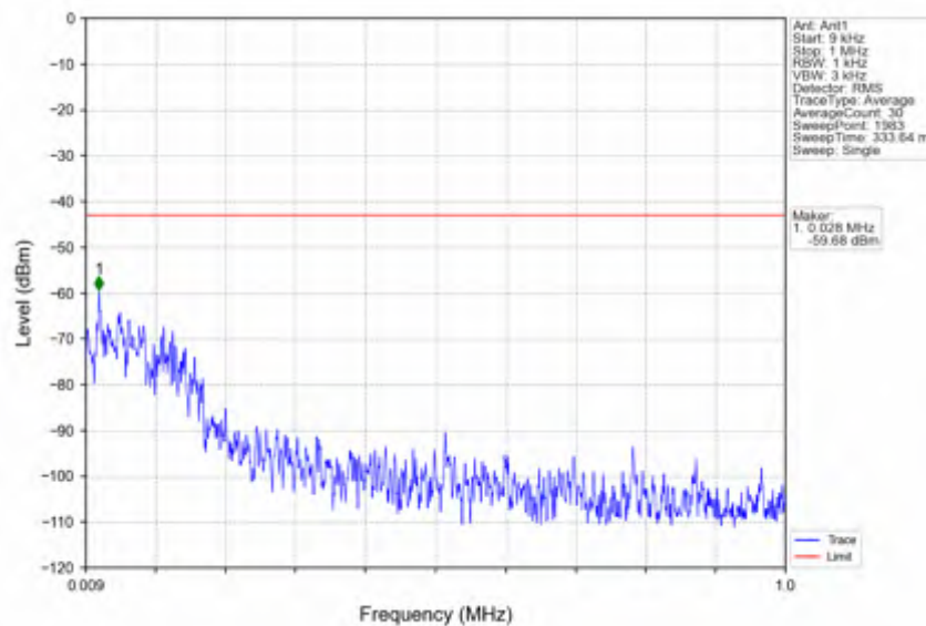
n78e_15kHz_SISO_NTNV_30MHz_CP-OFDM_QPSK_3465MHz_Inner_1RB_Left
