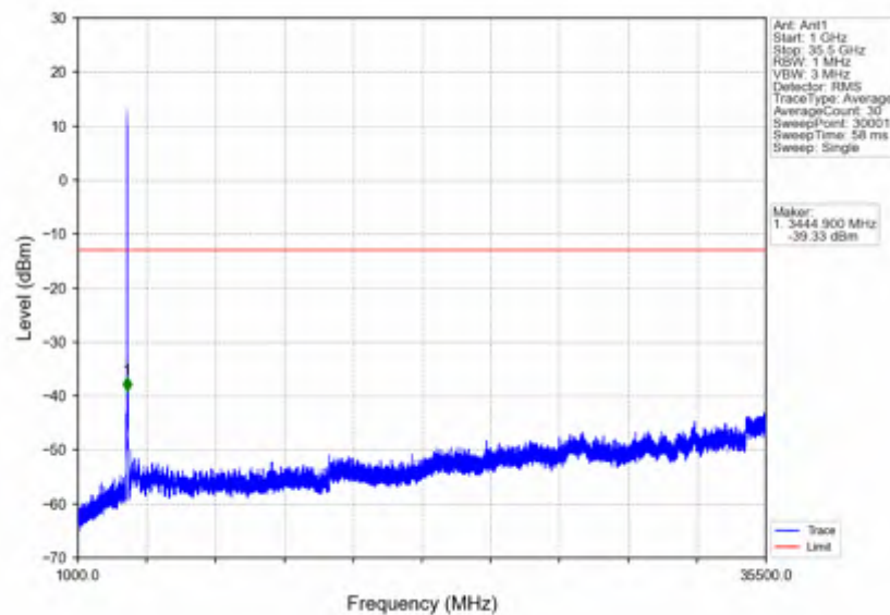
n78e_15kHz_SISO_NTNV_30MHz_DFT-s-OFDM_QPSK_3465MHz_Inner_1RB_Left
