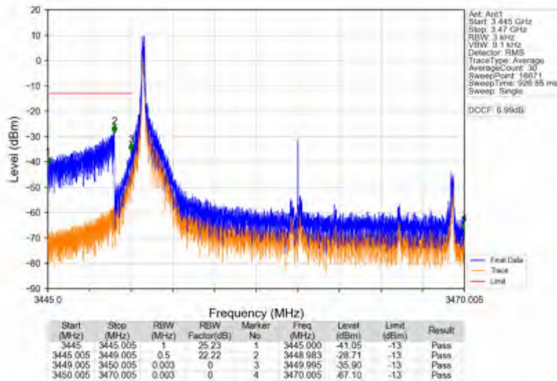
n78e_15kHz_SISO_NTNV_20MHz_DFT-s-OFDM QPSK_3460.005MHz_Inner_1RB_Left
