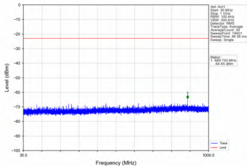
n78e_15kHz_SISO_NTNV_50MHz_DFT-s-OFDM QPSK_3475.005MHz_Inner_1RB_Left
