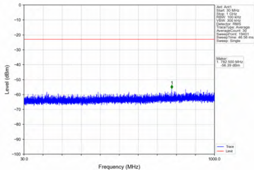
n78e_15kHz_SISO_NTNV_50MHz_CP-OFDM_QPSK_3499.995MHz_Edge_1RB_Left
