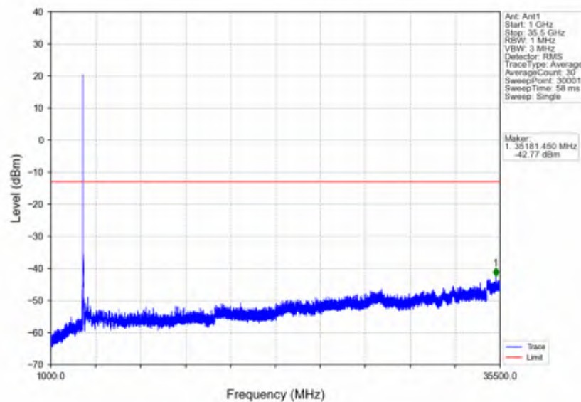
n78e_15kHz_SISO_NTNV_50MHz_DFT-s-OFDM QPSK_3475.005MHz_Inner_1RB_Left
