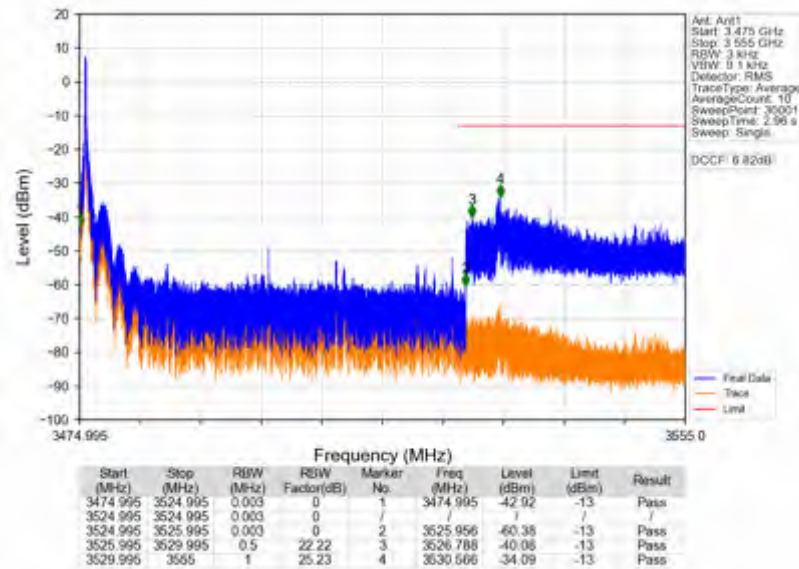
n78e_15kHz_SISO_NTNV_50MHz_CP-OFDM_QPSK_3499.995MHz_Edge_1RB_Left
