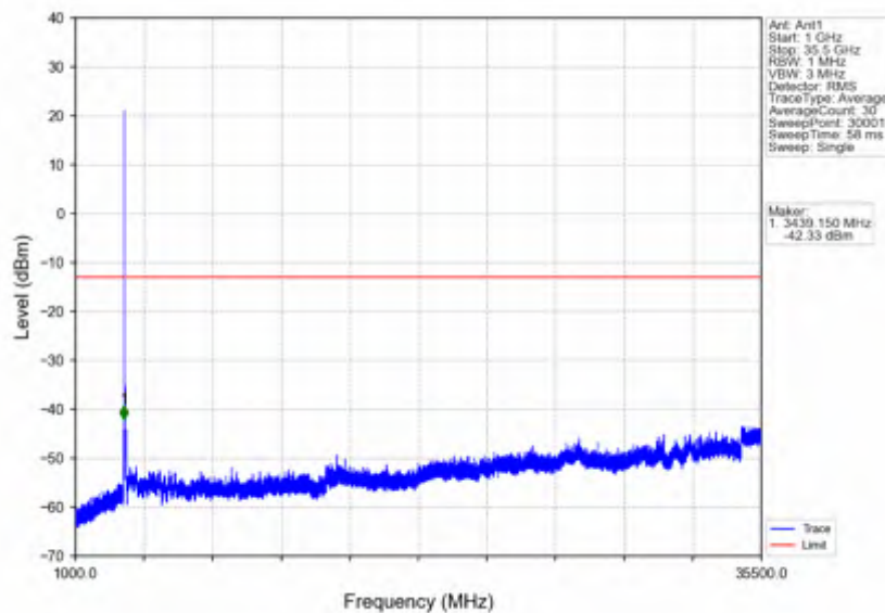
n78e_15kHz_SISO_NTNV_50MHz_CP-OFDM_QPSK_3499.995MHz_Edge_1RB_Left
