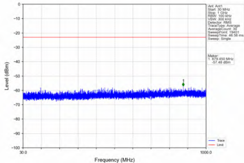
n78e_15kHz_SISO_NTNV_40MHz_CP-OFDM_QPSK_3499.995MHz_Edge_1RB_Left
