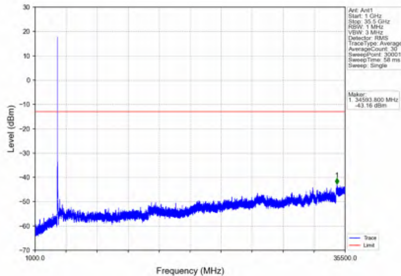
n78e_15kHz_SISO_NTNV_40MHz_CP-OFDM_QPSK_3499.995MHz_Edge_1RB_Left
