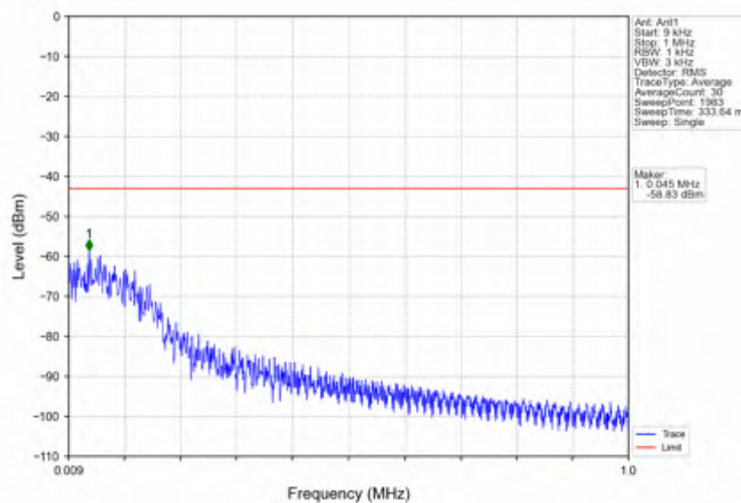
n25_15kHz_SISO_NTNV_30MHz_CP-OFDM_QPSK_1865MHz_Inner_1RB_Left
