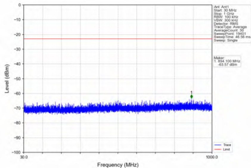
n25 15kHz SISO NTNv 20MHz CP-OFDM QPSK 1882.5MHz Edge 1RB Left
