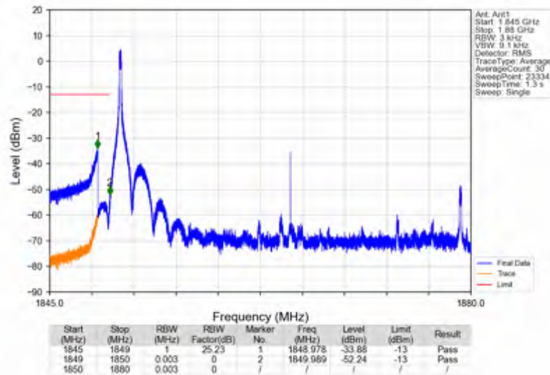
n25_15kHz_SISO_NTNV_30MHz_DFT-s-OFDM QPSK_1865MHz_Inner_1RB_Left
