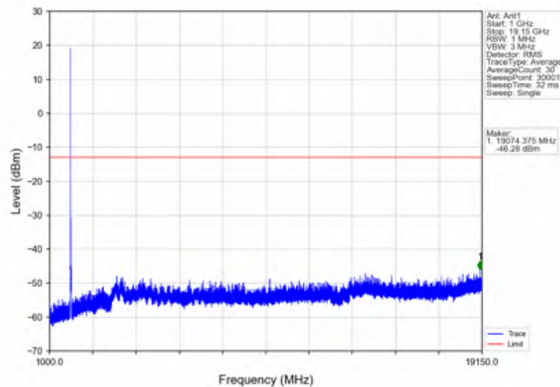
n25 15kHz SISO NTNv 20MHz CP-OFDM QPSK 1882.5MHz Edge 1RB Left
