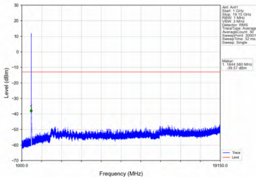
n25_15kHz_SISO_NTNV_20MHz_DFT-s-OFDM QPSK_1860MHz_Inner_1RB_Left
