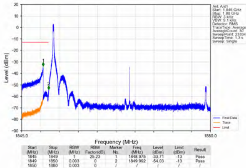
n25_15kHz_SISO_NTNV_30MHz_CP-OFDM_QPSK_1865MHz_Inner_1RB_Left
