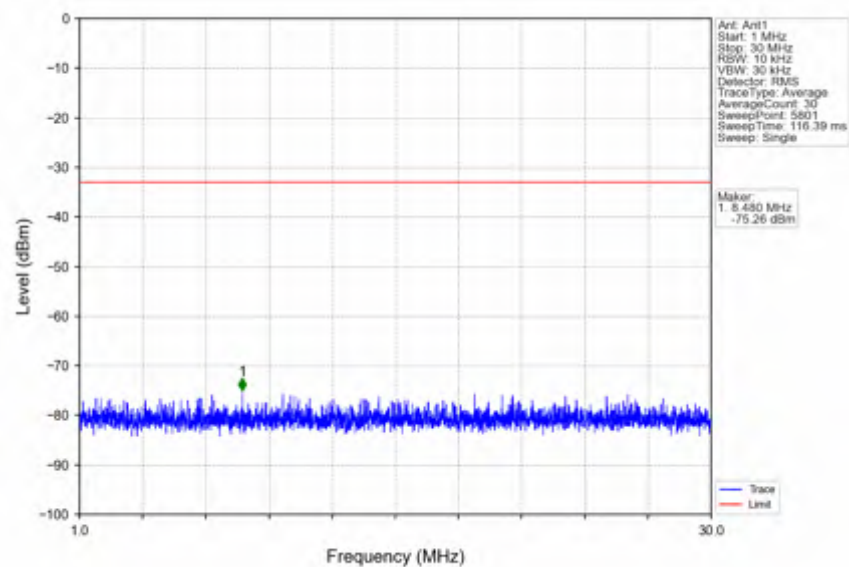
n25 15kHz SISO NTNV 30MHz CP-OFDM QPSK 1882.5MHz Edge 1RB Left
