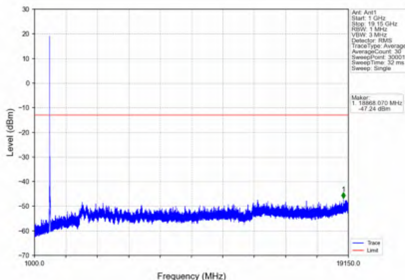
n25 15kHz SISO NTN 25MHz CP-OFDM QPSK 1882.5MHz Edge 1RB Left
