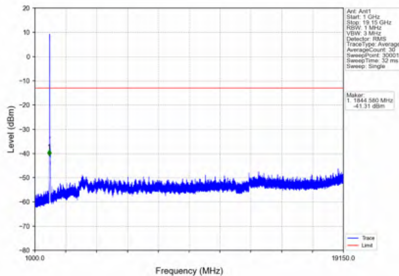
n25_15kHz_SISO_NTNV_30MHz_DFT-s-OFDM QPSK_1865MHz_Inner_1RB_Left
