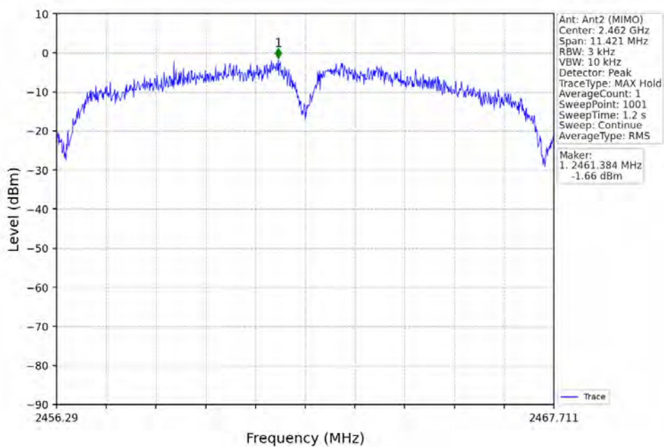
802.11b_HCH_2462MHz_Ant2 (MIMO)_NTNV
