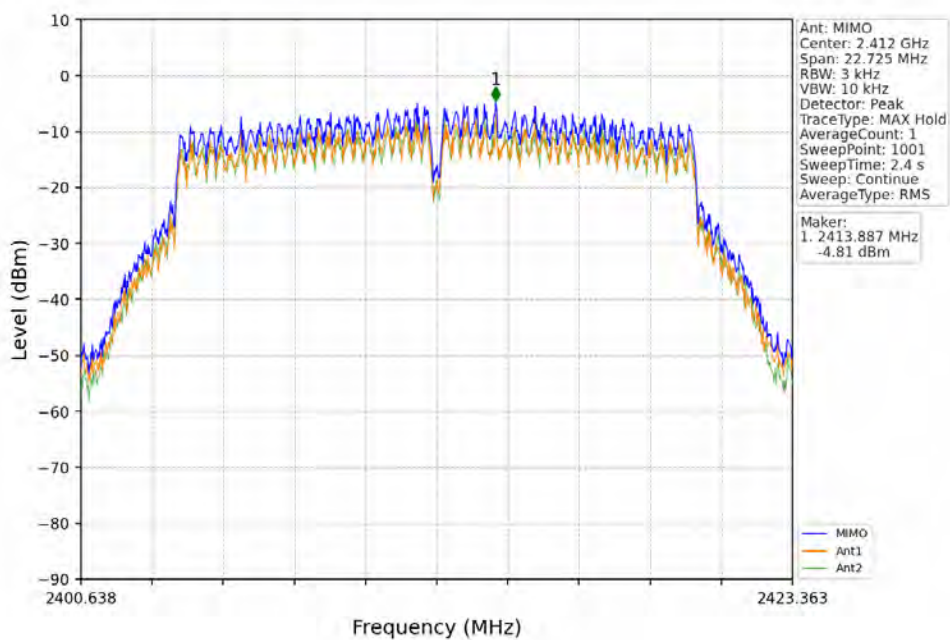
802.11g_LCH_2412MHz_MIMO_NTNV
