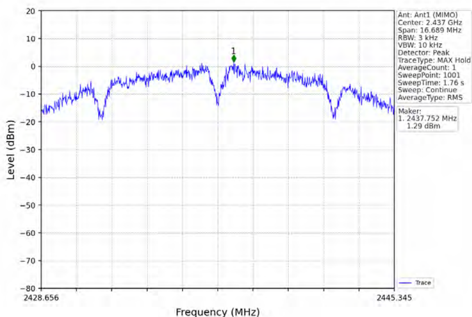
802.11b_MCH_2437MHz_Ant1 (MIMO)_NTNV
