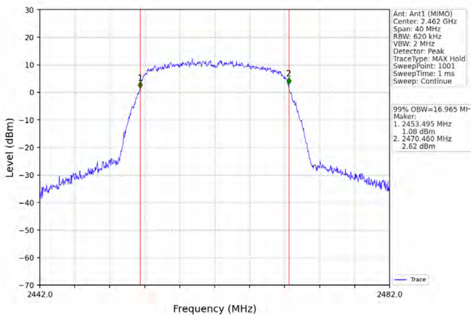
802.11g_HCH_2462MHz_Ant1 (MIMO)_NTNV
