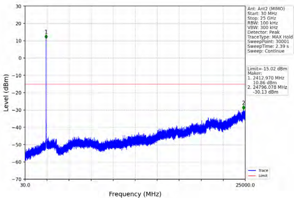
802.11b_LCH_2412MHz_Ant2 (MIMO)_NTNV
