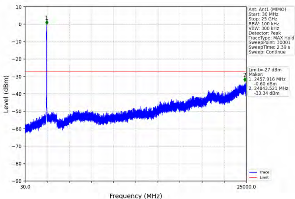
802.11ax(HEW40)_HCH_2452MHz_RU484_Left_Ant1 (MIMO)_NTNV
