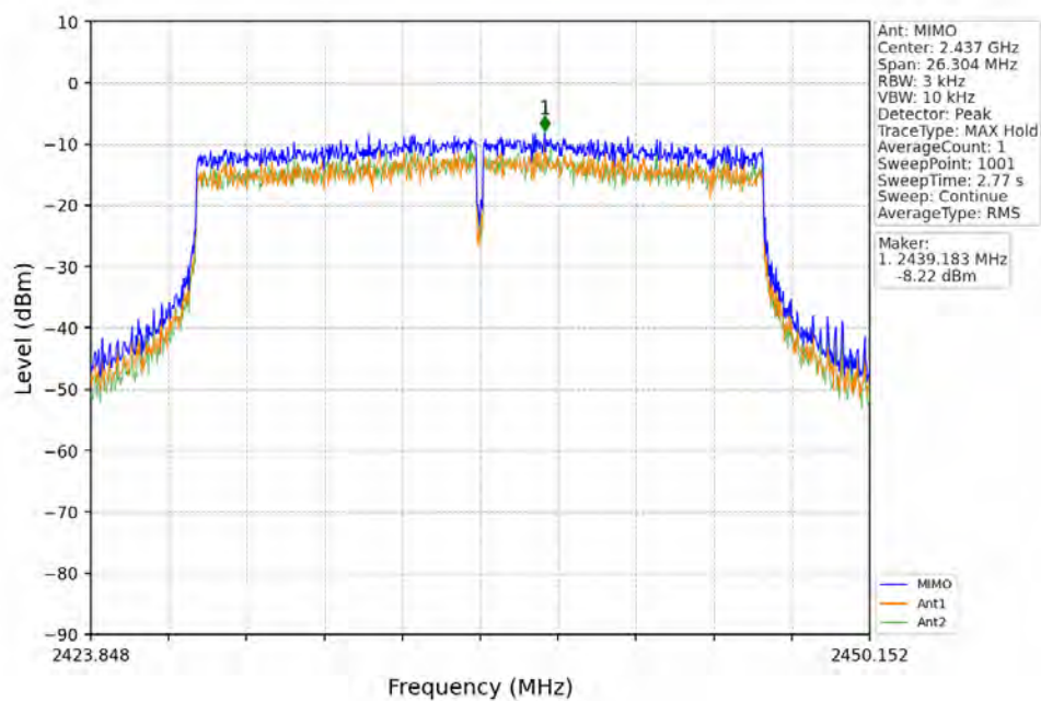
802.11ax(HEW20)_MCH_2437MHz_RU242_Left_MIMO_NTNV
