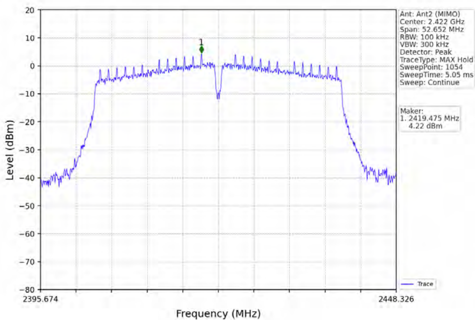
802.11n(HT40)_LCH_2422MHz_Ant2 (MIMO)_NTNV
