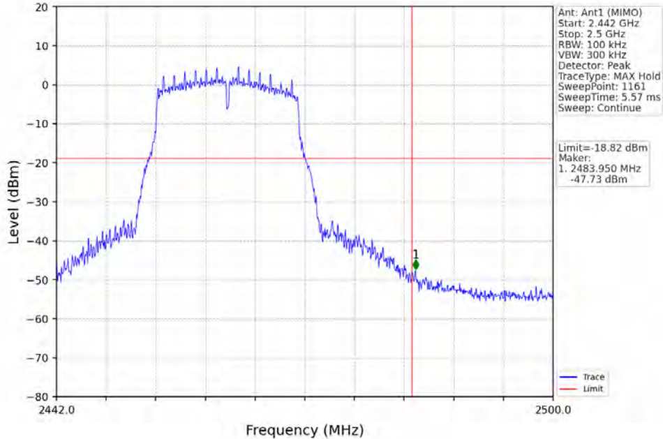
802.11g_HCH_2462MHz_Ant1 (MIMO)_NTNV
