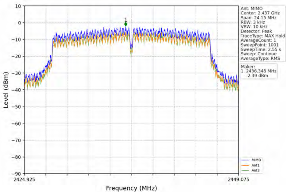
802.11n(HT20)_MCH_2437MHz_MIMO_NTNV
