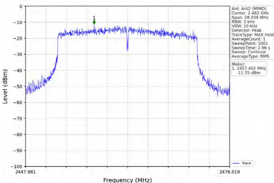
802.11ax(HEW20)_HCH_2462MHz_RU242_Left_Ant2 (MIMO)_NTNV
