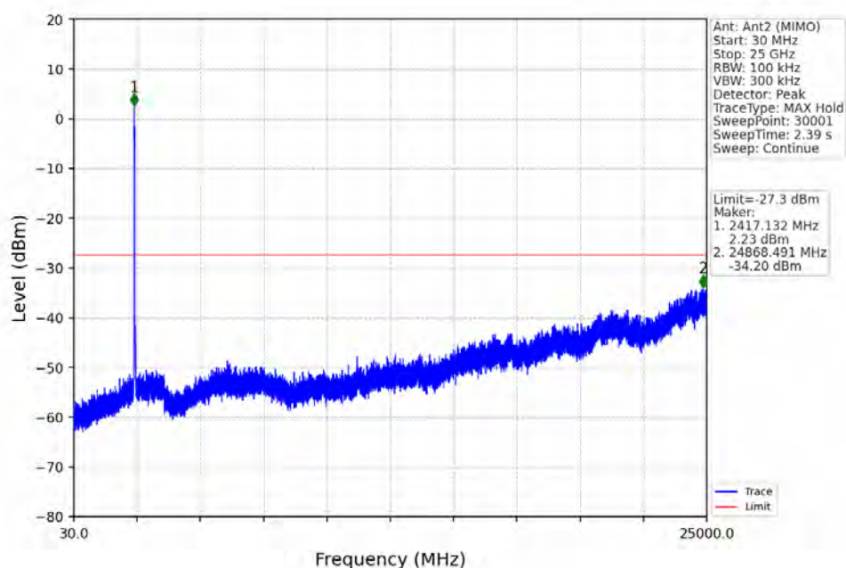
802.11ax(HEW40)_LCH_2422MHz_RU484_Left_Ant2 (MIMO)_NTNV
