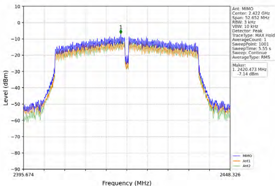
802.11n(HT40)_LCH_2422MHz_MIMO_NTNV
