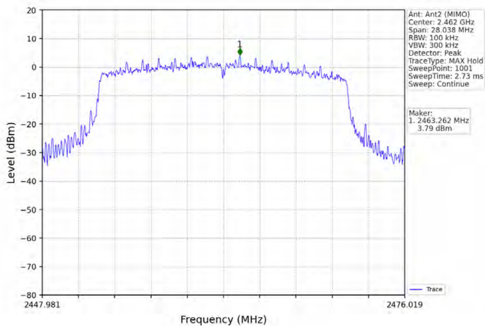
802.11ax(HEW20)_HCH_2462MHz_RU242_Left_Ant2 (MIMO)_NTNV
