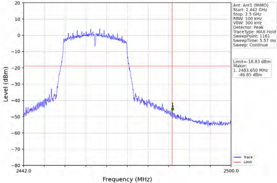
802.11n(HT20)_HCH_2462MHz_Ant1 (MIMO)_NTNV
