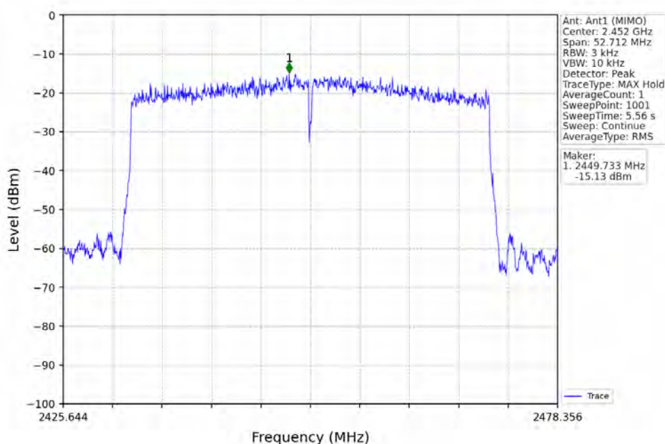
802.11ax(HEW40)_HCH_2452MHz_RU484_Left_Ant1 (MIMO)_NTNV
