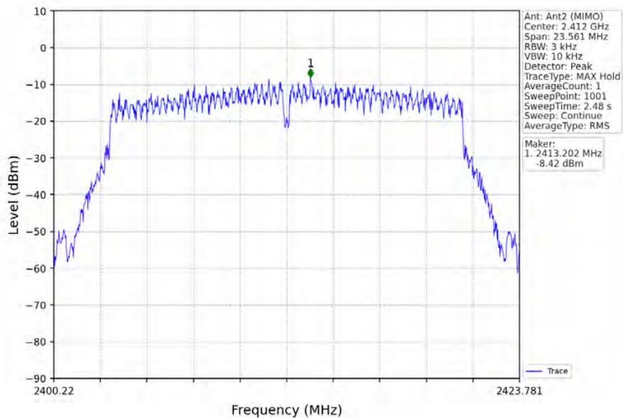
802.11n(HT20)_LCH_2412MHz_Ant2 (MIMO)_NTNV
