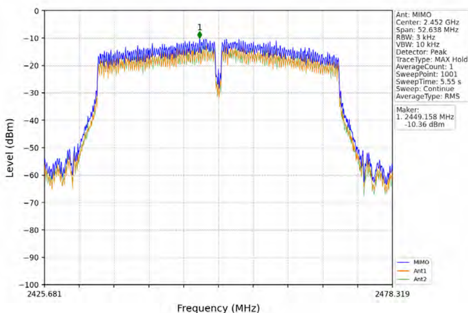
802.11n(HT40)_HCH_2452MHz_MIMO_NTNV
