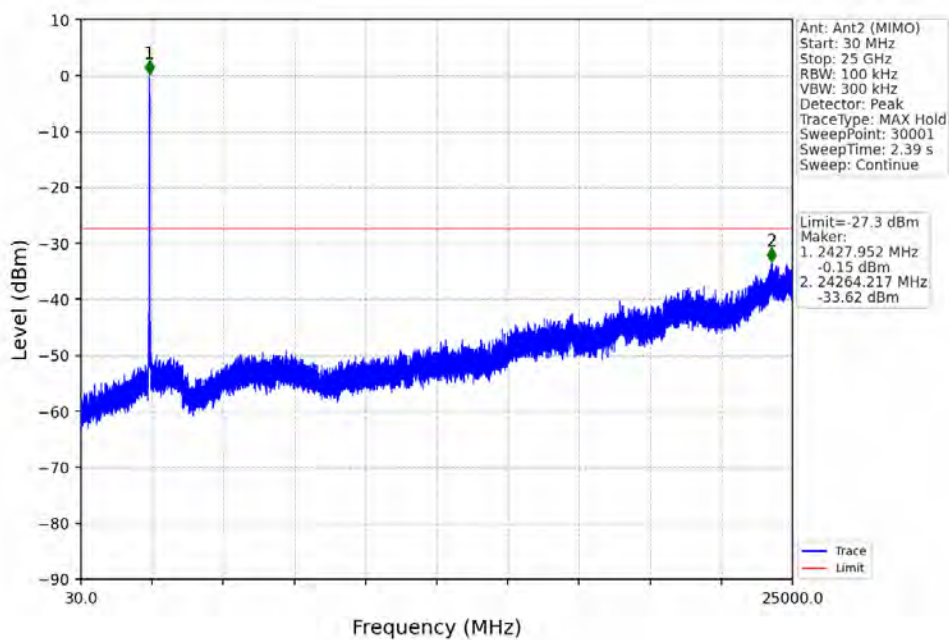
802.11ax(HEW40)_MCH_2437MHz_RU484_Left_Ant2 (MIMO)_NTNV
