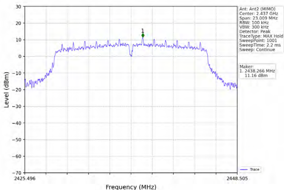
802.11g_MCH_2437MHz_Ant2 (MIMO)_NTNV
