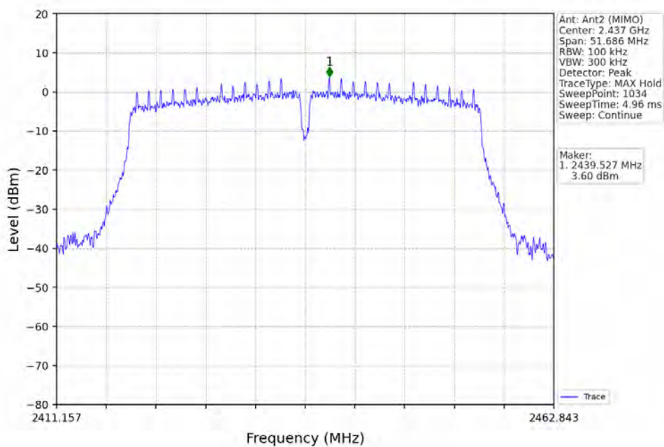
802.11n(HT40)_MCH_2437MHz_Ant2 (MIMO)_NTNV
