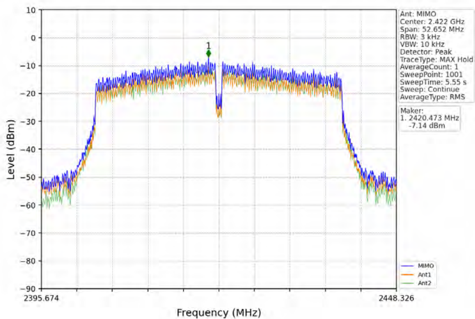
802.11n(HT40)_LCH_2422MHz_MIMO_NTNV
