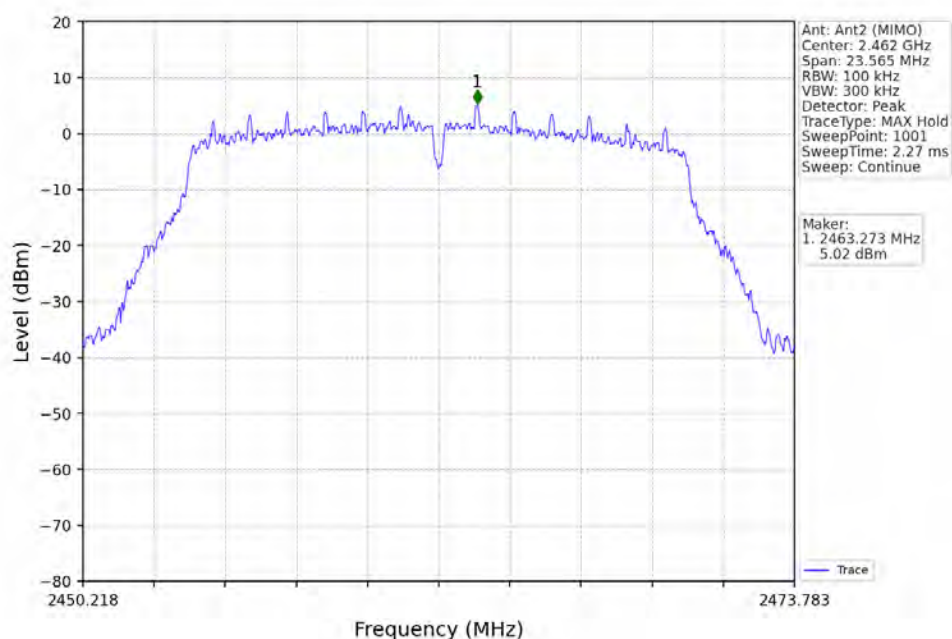
802.11g_HCH_2462MHz_Ant2 (MIMO)_NTNV
