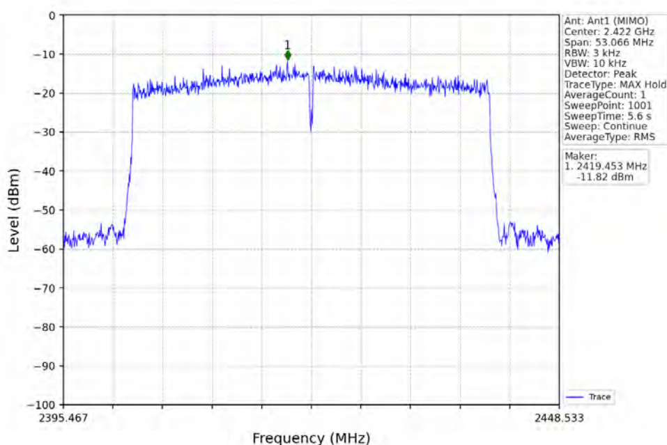
802.11ax(HEW40)_LCH_2422MHz_RU484_Left_Ant1 (MIMO)_NTNV
