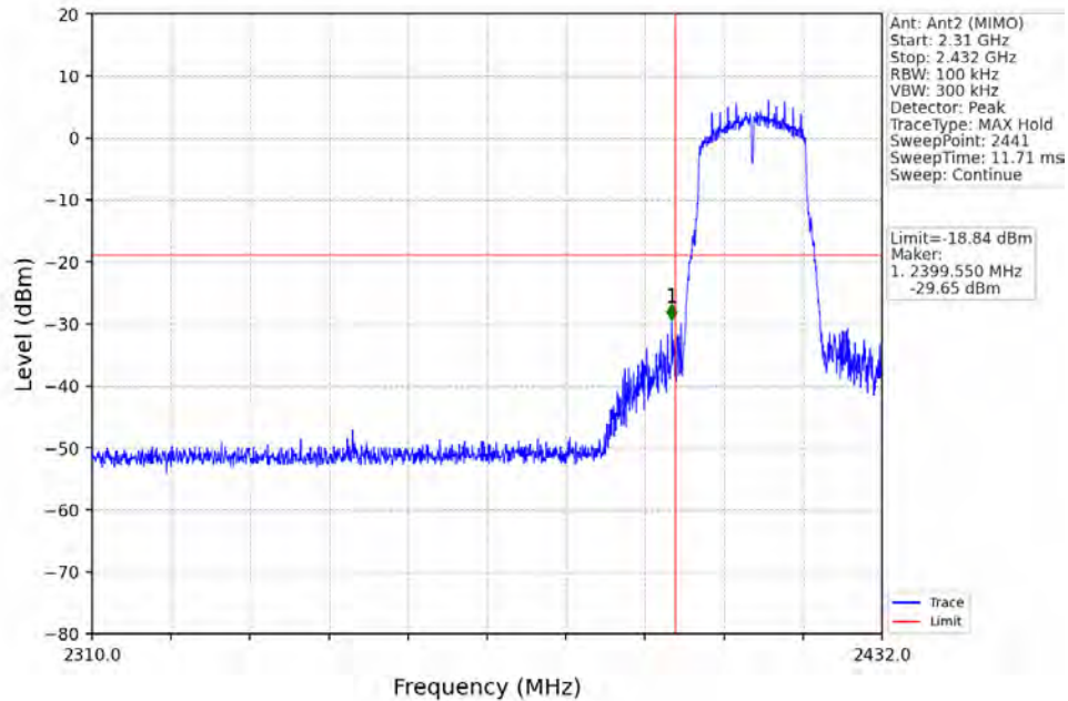
802.11g_LCH_2412MHz_Ant2 (MIMO)_NTNV
