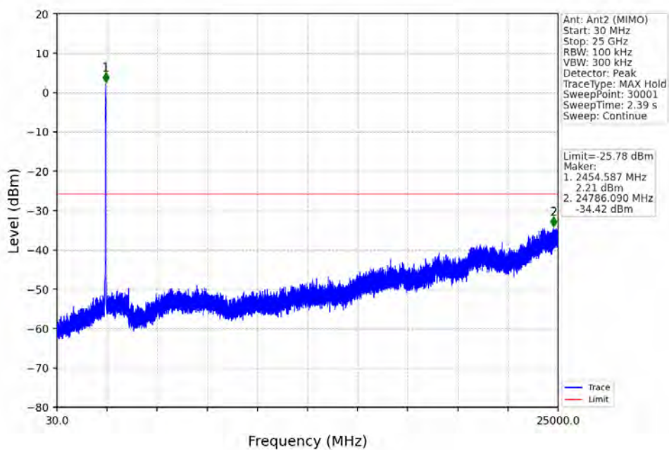
802.11n(HT40)_HCH_2452MHz_Ant2 (MIMO)_NTNV
