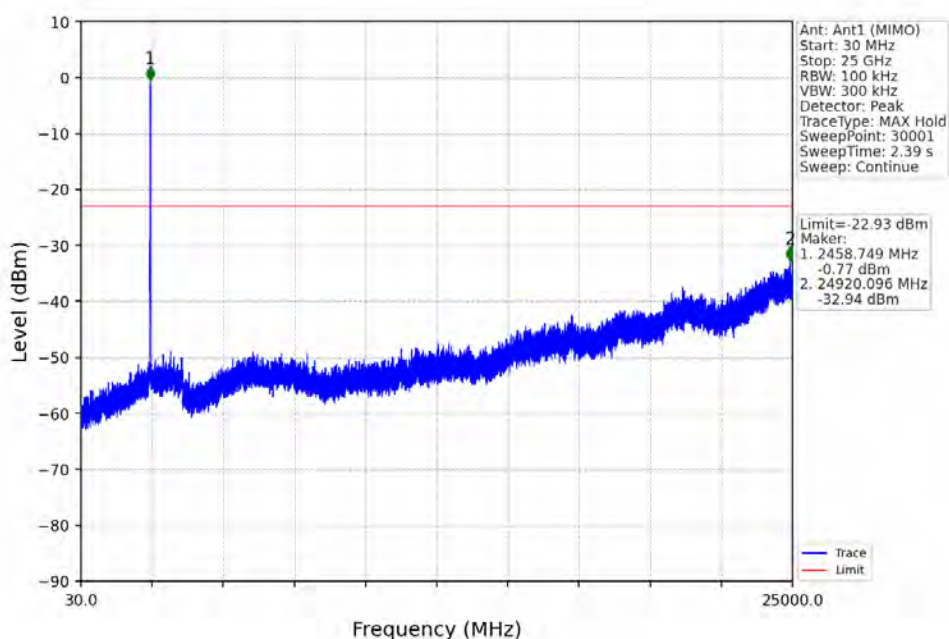
802.11ax(HEW20)_HCH_2462MHz_RU242_Left_Ant1 (MIMO)_NTNV
