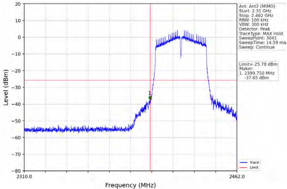
802.11n(HT40)_LCH_2422MHz_Ant2 (MIMO)_NTNV
