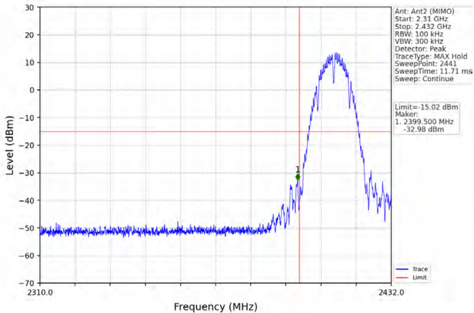
802.11b_LCH_2412MHz_Ant2 (MIMO)_NTNV
