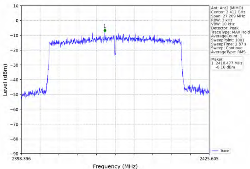
802.11ax(HEW20)_LCH_2412MHz_RU242_Left_Ant2 (MIMO)_NTNV
