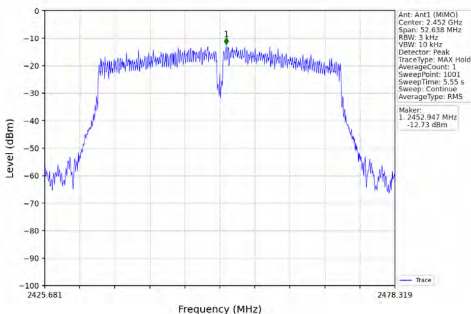
802.11n(HT40)_HCH_2452MHz_Ant1 (MIMO)_NTNV
