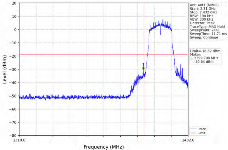
802.11g_LCH_2412MHz_Ant1 (MIMO)_NTNV
