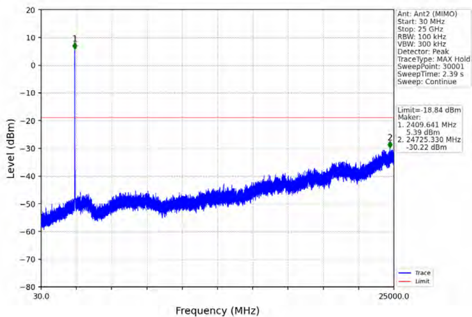
802.11g_LCH_2412MHz_Ant2 (MIMO)_NTNV
