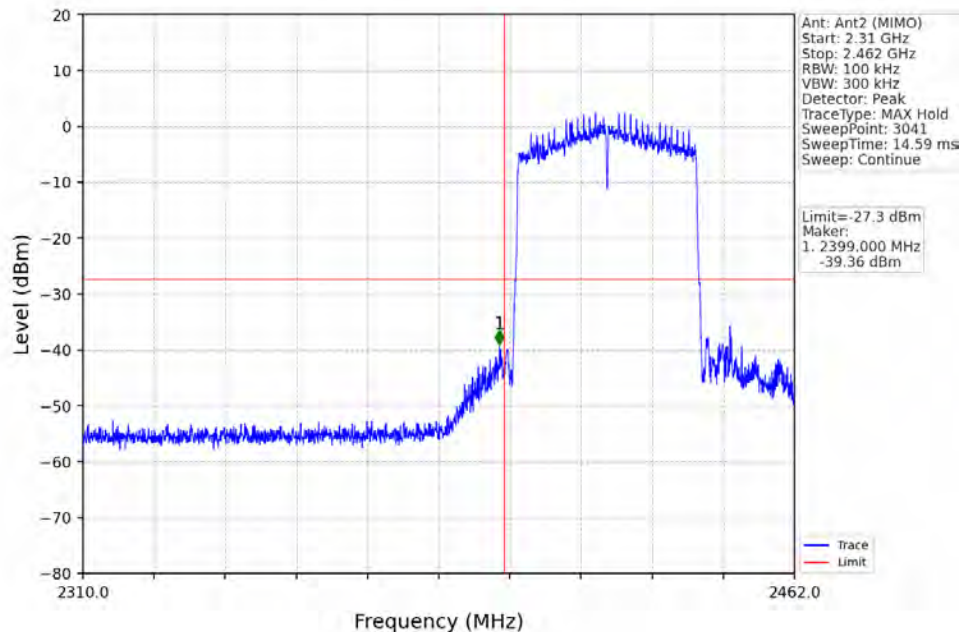
802.11ax(HEW40)_LCH_2422MHz_RU484_Left_Ant2 (MIMO)_NTNV
