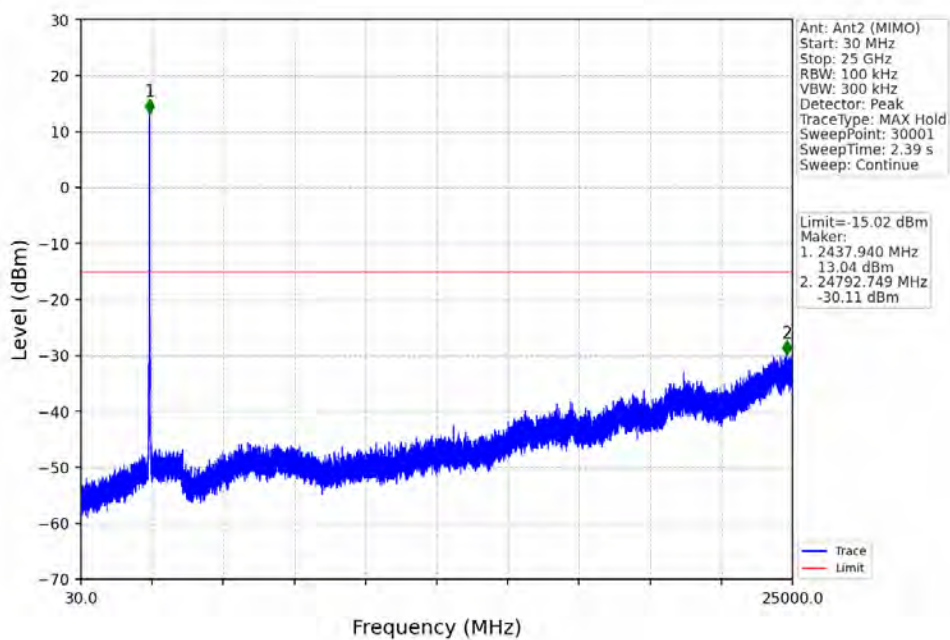
802.11b_MCH_2437MHz_Ant2 (MIMO)_NTNV
