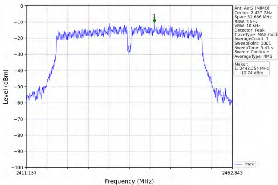
802.11n(HT40)_MCH_2437MHz_Ant2 (MIMO)_NTNV
