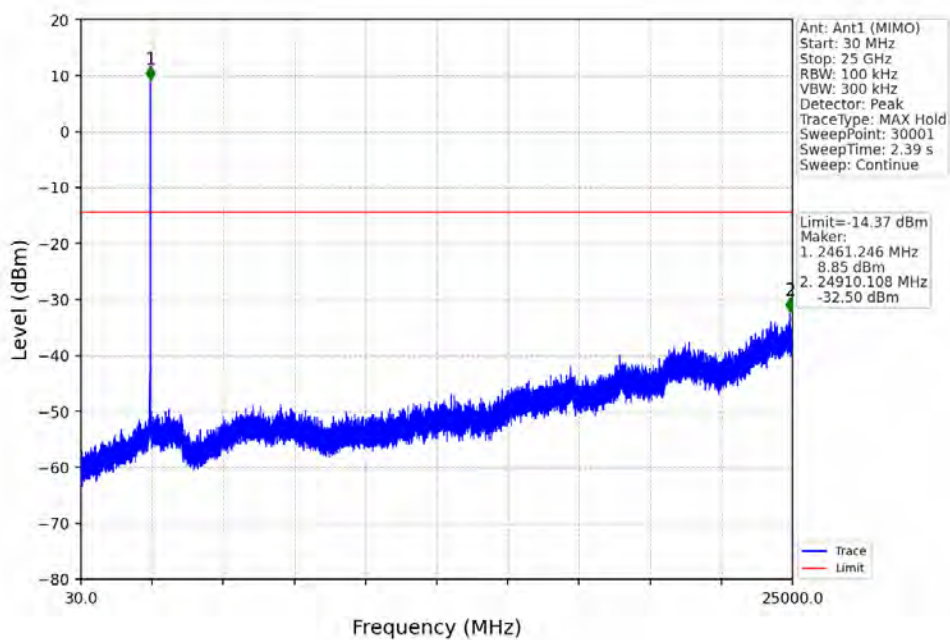
802.11b_HCH_2462MHz_Ant1 (MIMO)_NTNV
