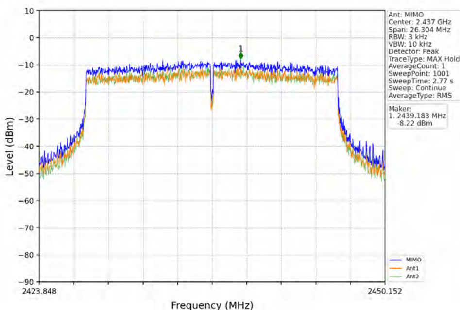
802.11ax(HEW20)_MCH_2437MHz_RU242_Left_MIMO_NTNV
