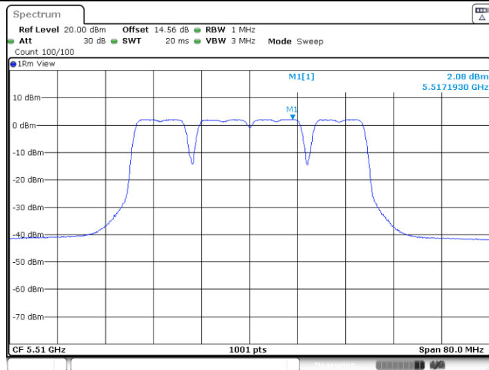
11BE40MIMO_Ant4_5510_52Tone_RU8
