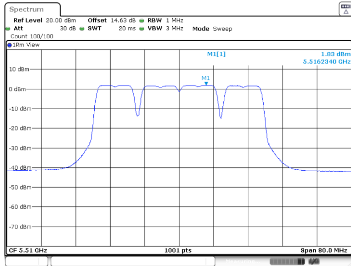
11BE40MIMO_Ant3_5510_52Tone_RU8
