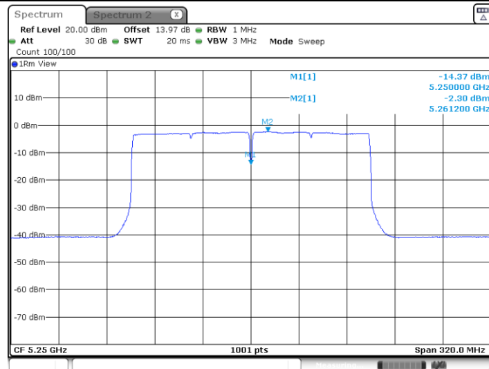
11BE160MIMO_Ant2_5250_UNII-2A
