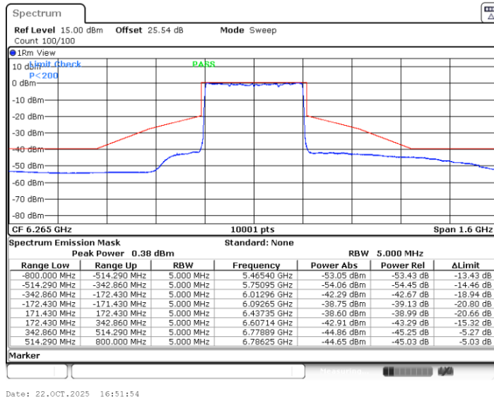
11BE320MIMO_Ant2_6265
