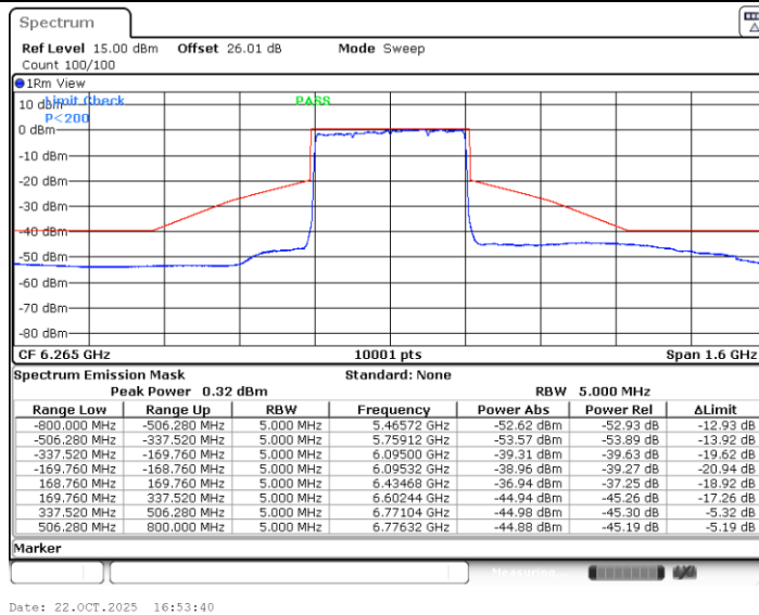
11BE320MIMO_Ant2_6265
