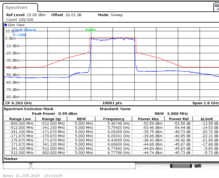
11BE320MIMO_Ant2_6265
