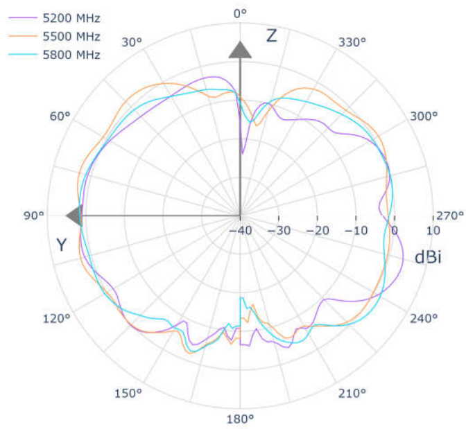
YZ_Pol._Theta_Ant.2@5G
