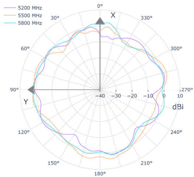
XY_Pol._Theta_Ant.2@5G
