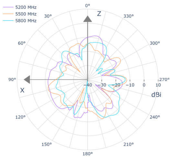
XZ_Pol._Phi_Ant.3@5G
