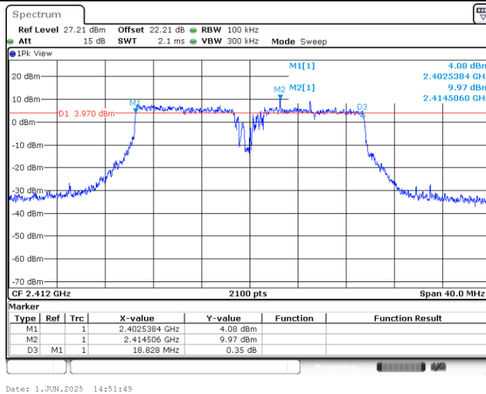
11BE20MIMO_Ant2_2412_52RU*4_RU4
