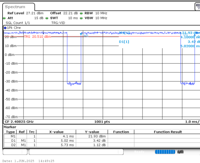
11BE20MIMO_Ant2_2412_52RU*4
