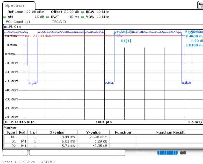
11BE20MIMO_Ant2_2412_52RU*4
