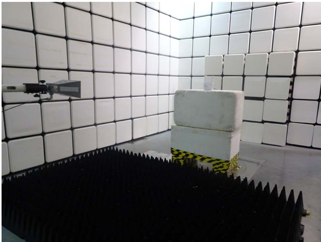
1GHz-18GHz
