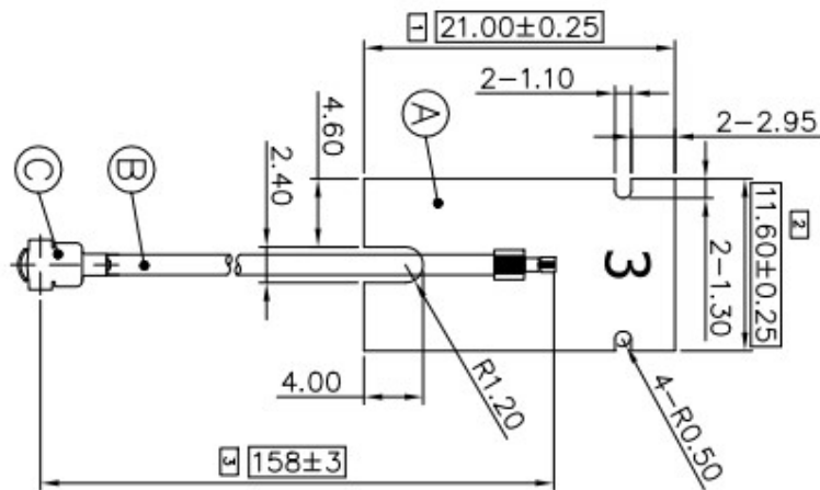
5G ANT 3
