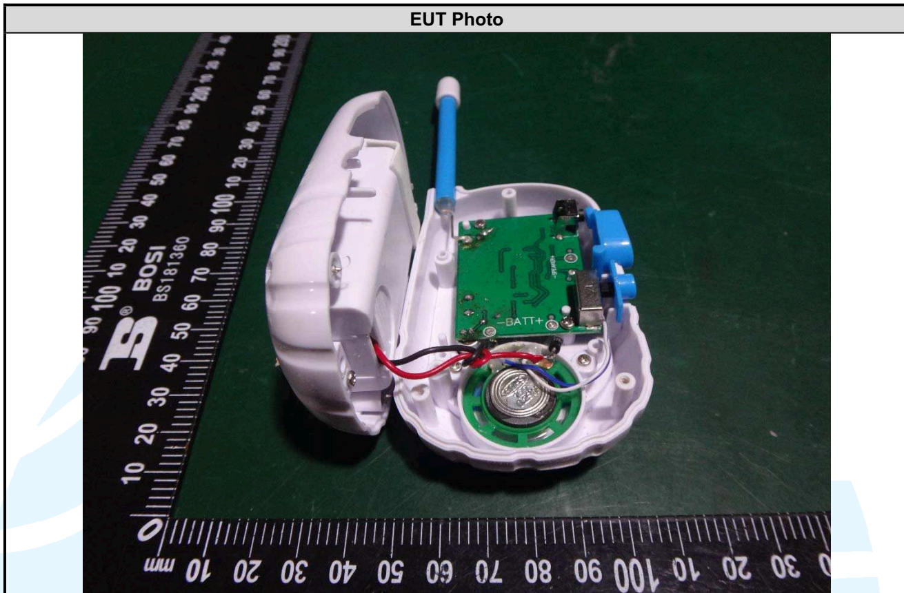
EUT Photo
