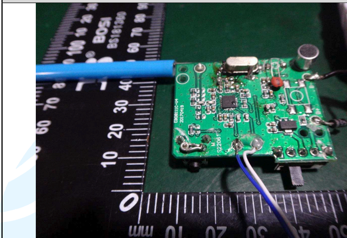
EUT Photo
