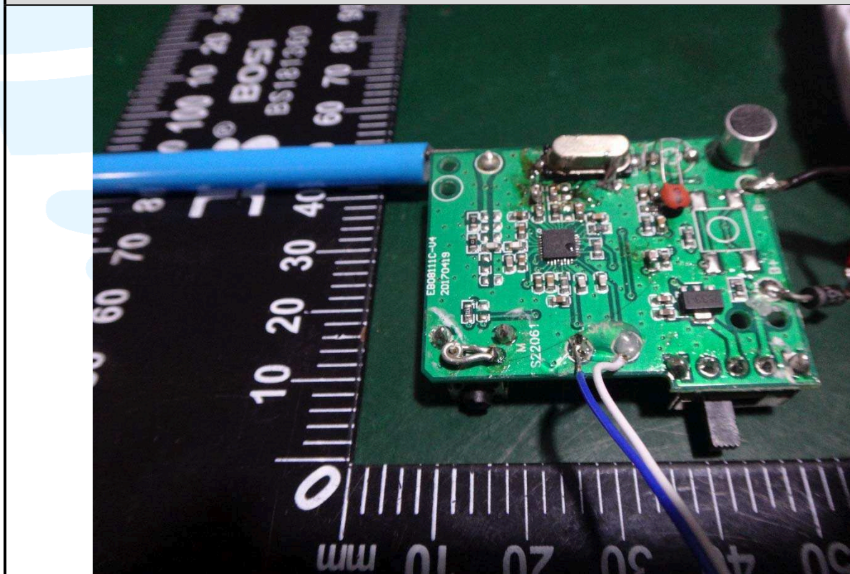
EUT Photo
