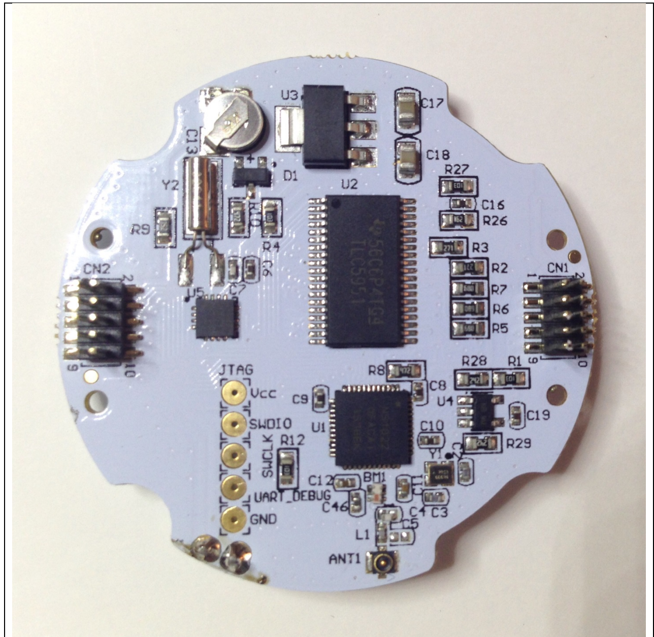
BLE Radio Board Bottom
