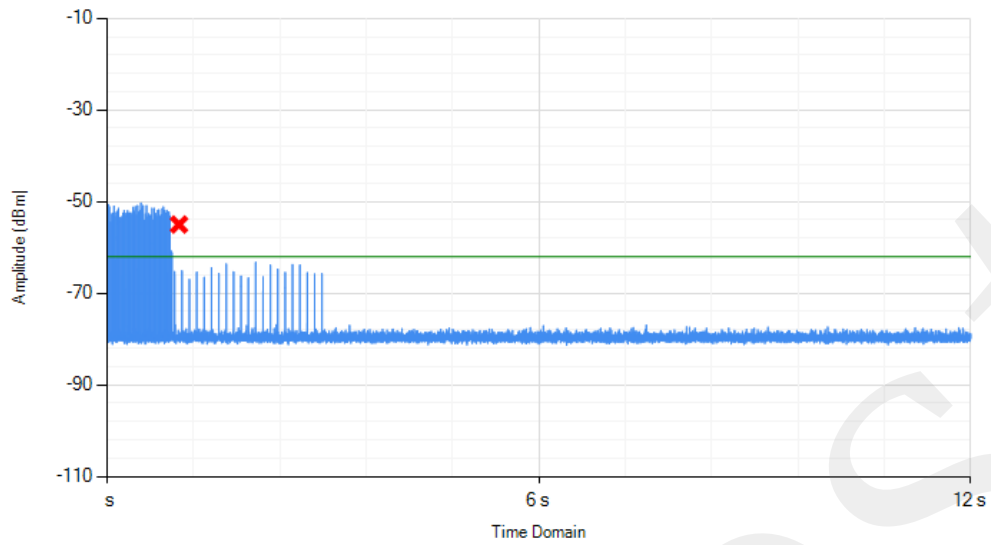
80MHz/5290MHz
