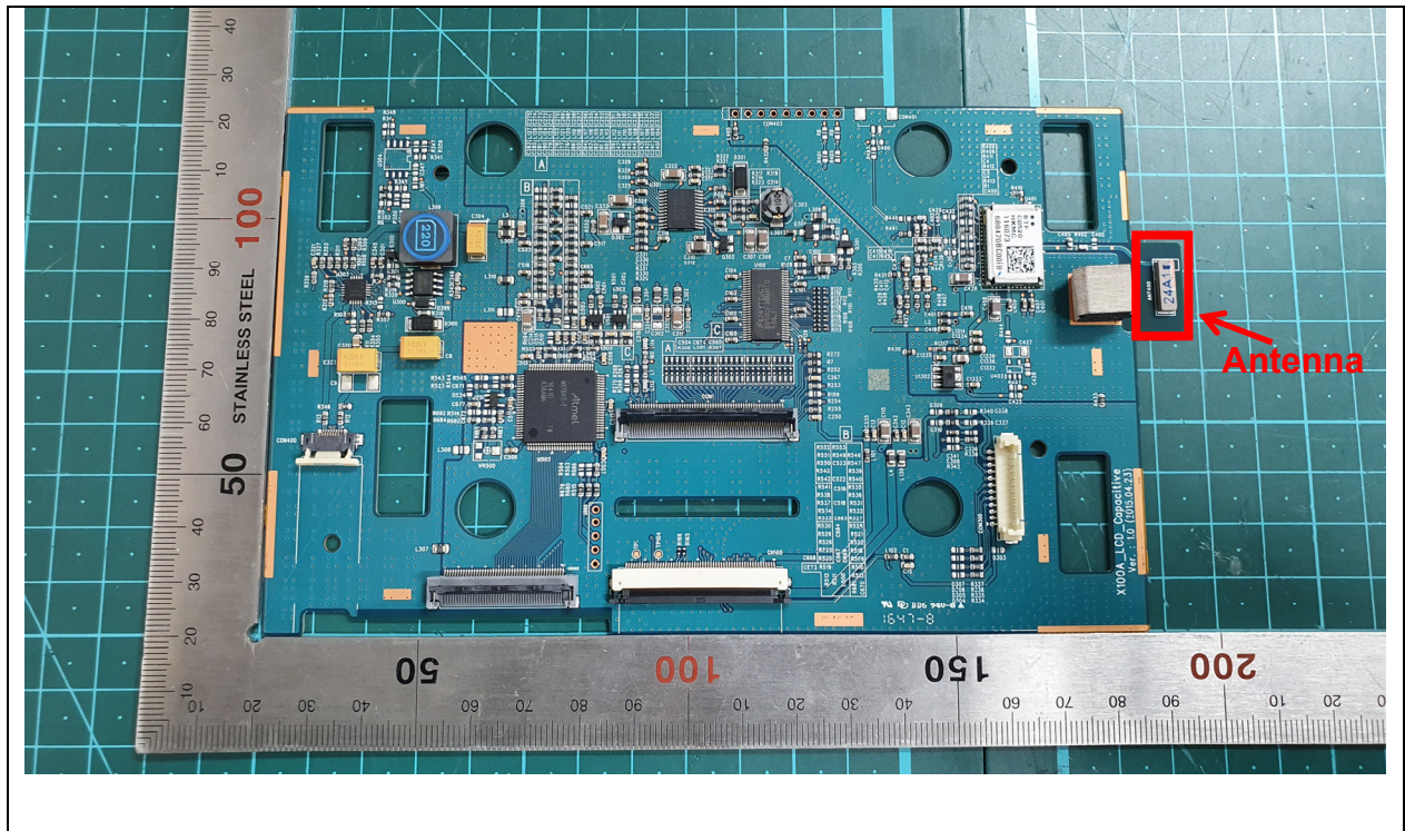
Antenna
