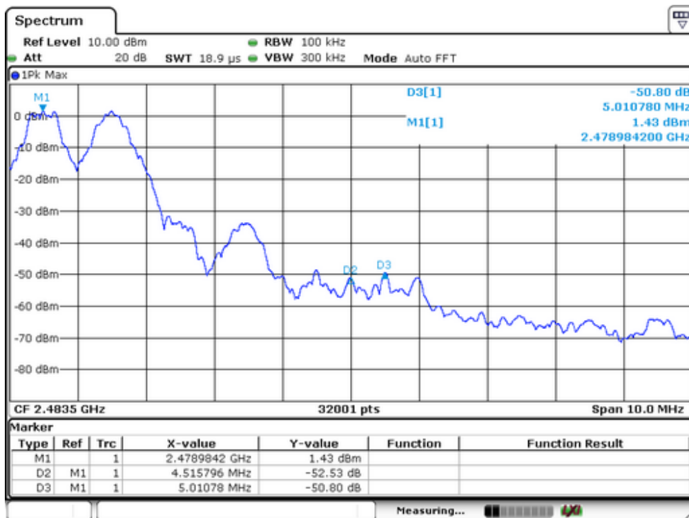
Test plots of \pi/4 -DQPSK
