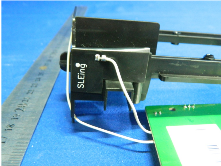
WIFI&BT ANTENNA
