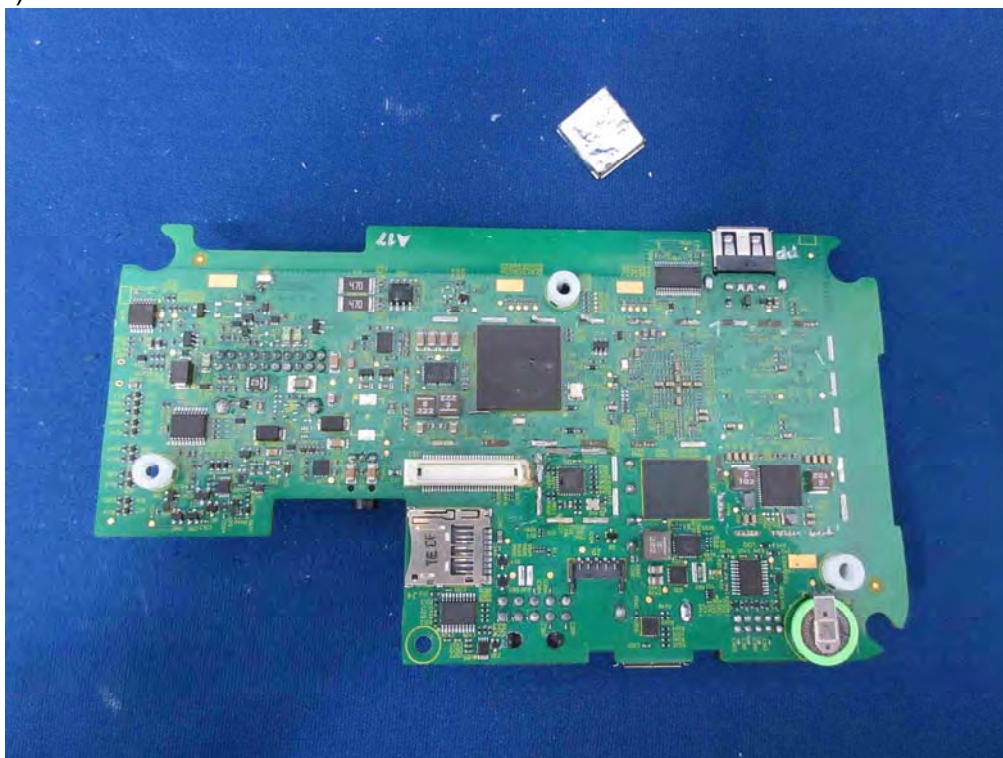
(72) EUT Photo
