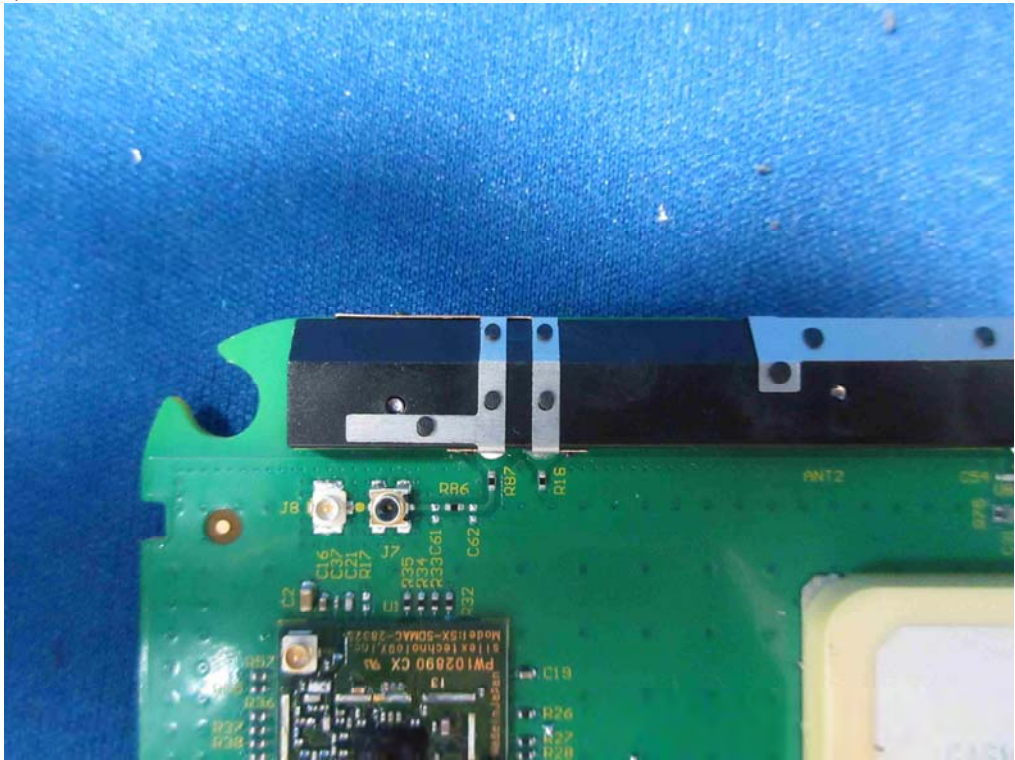
(70) EUT Photo
