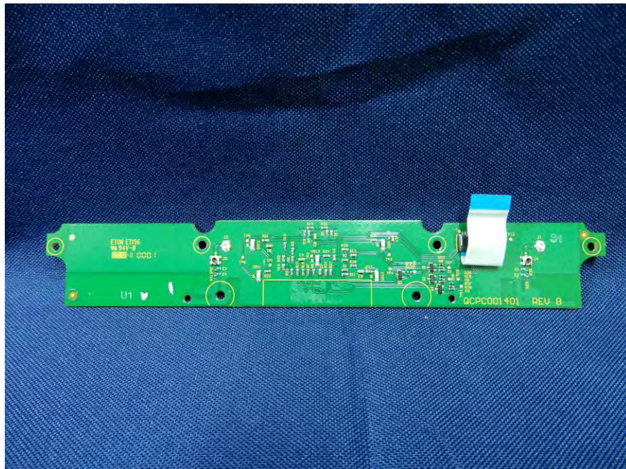
(30) EUT Photo
