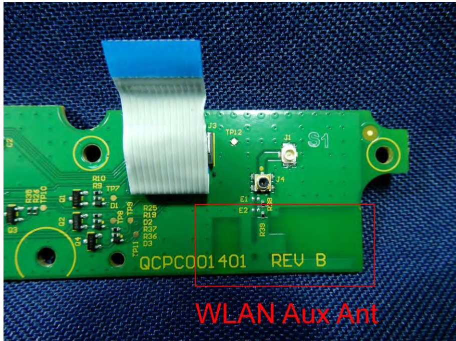
(31) EUT Photo
