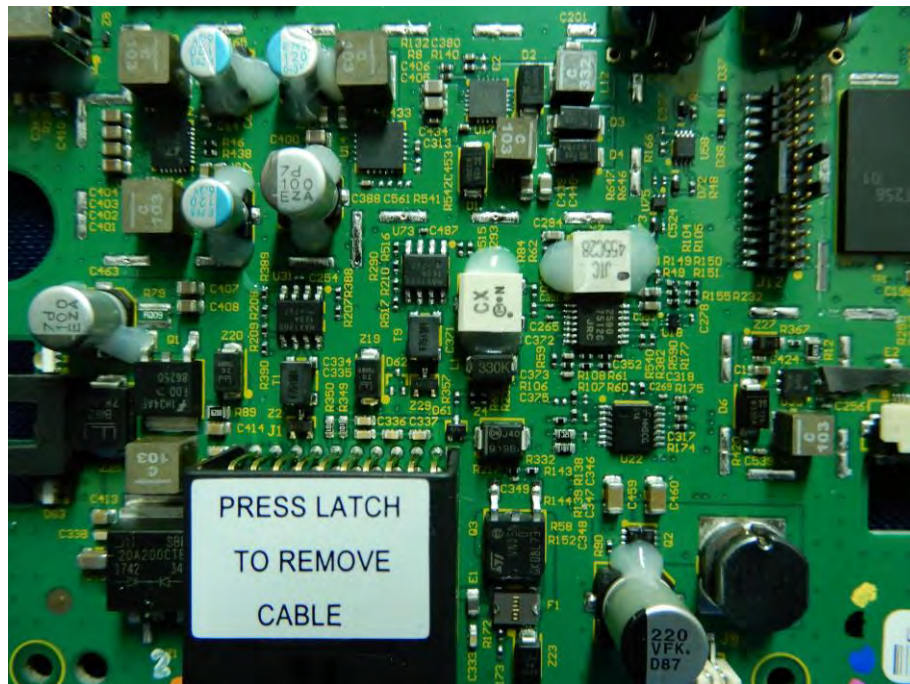
(19) EUT Photo
