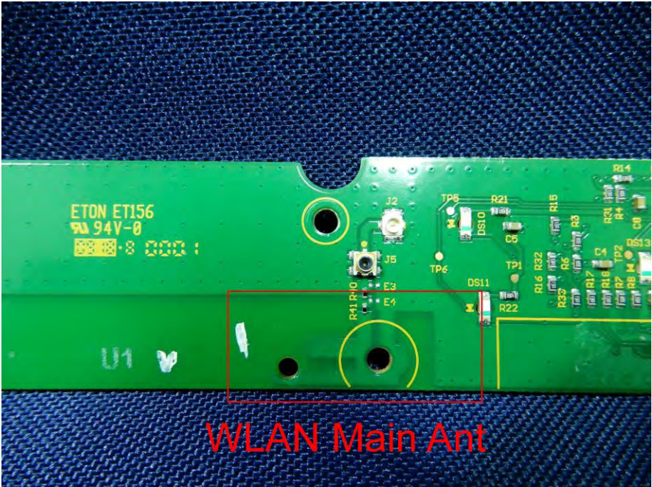
(33) EUT Photo
