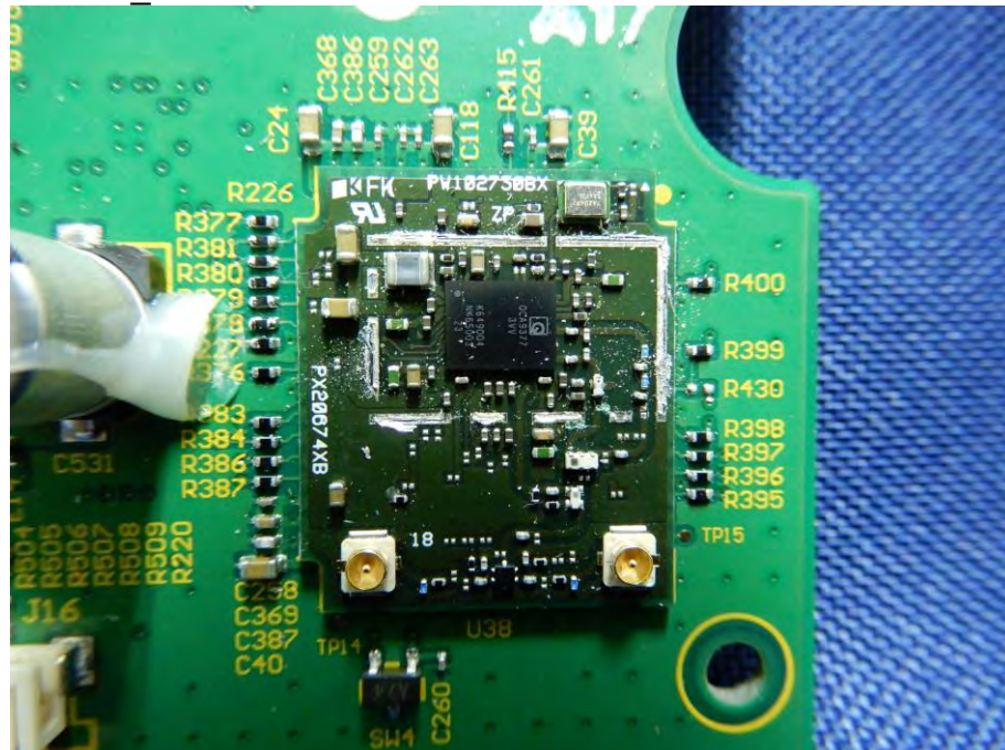
(16) EUT Photo_WLAN Module
