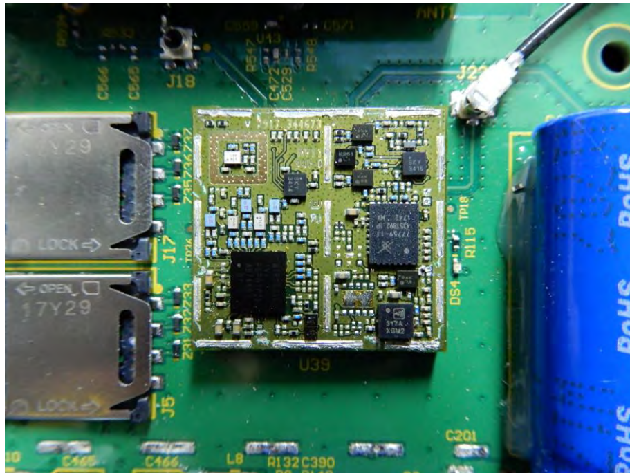
(15) EUT Photo_WWAN Module
