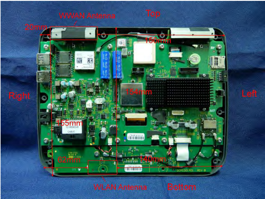
(8) EUT Photo
