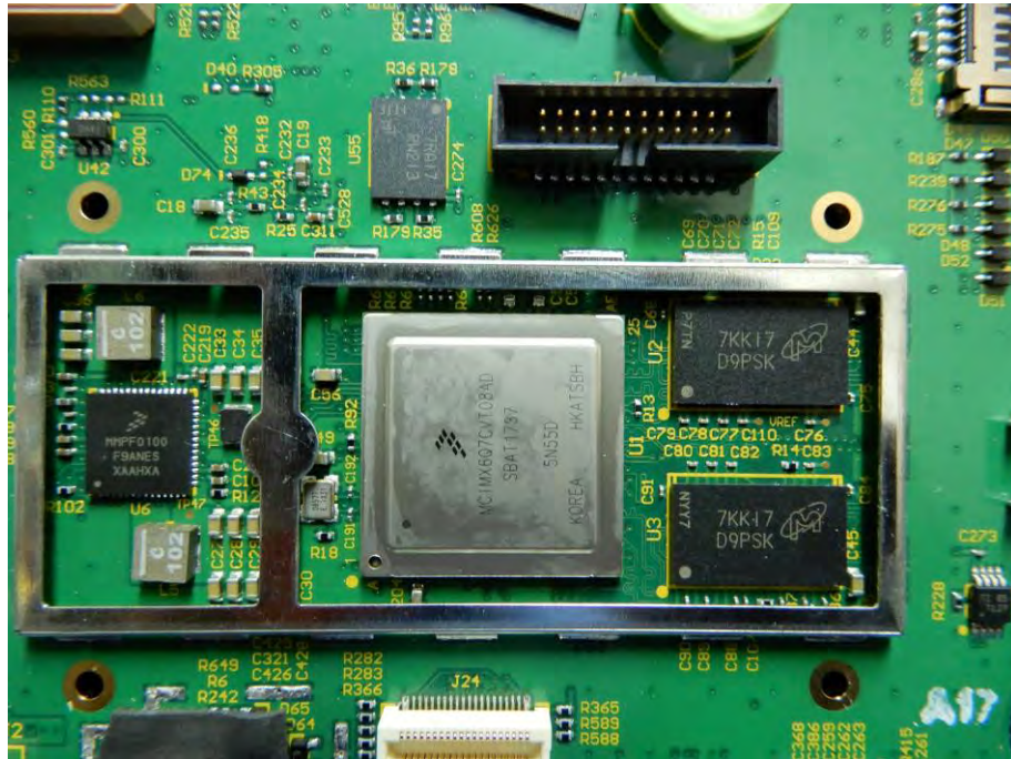
(17) EUT Photo
