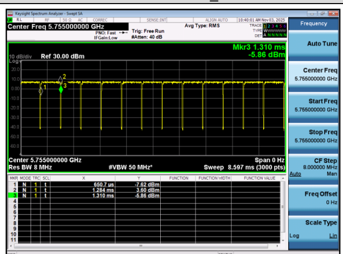
IEEE 802.11n-HT40_U-NII 3
