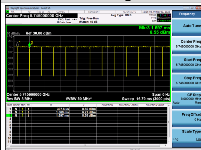
IEEE 802.11n-HT20_U-NII 3
