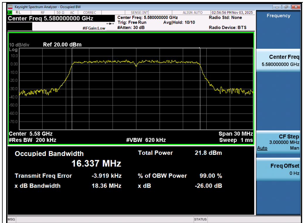
Test_Graph_802.11a_Ant 2_5580_6Mbps_OBW
