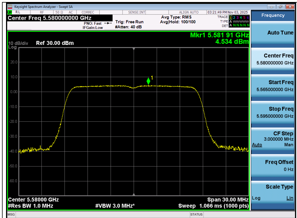
Test_Graph_802.11a_Ant 2_5580_6Mbps_PSD
